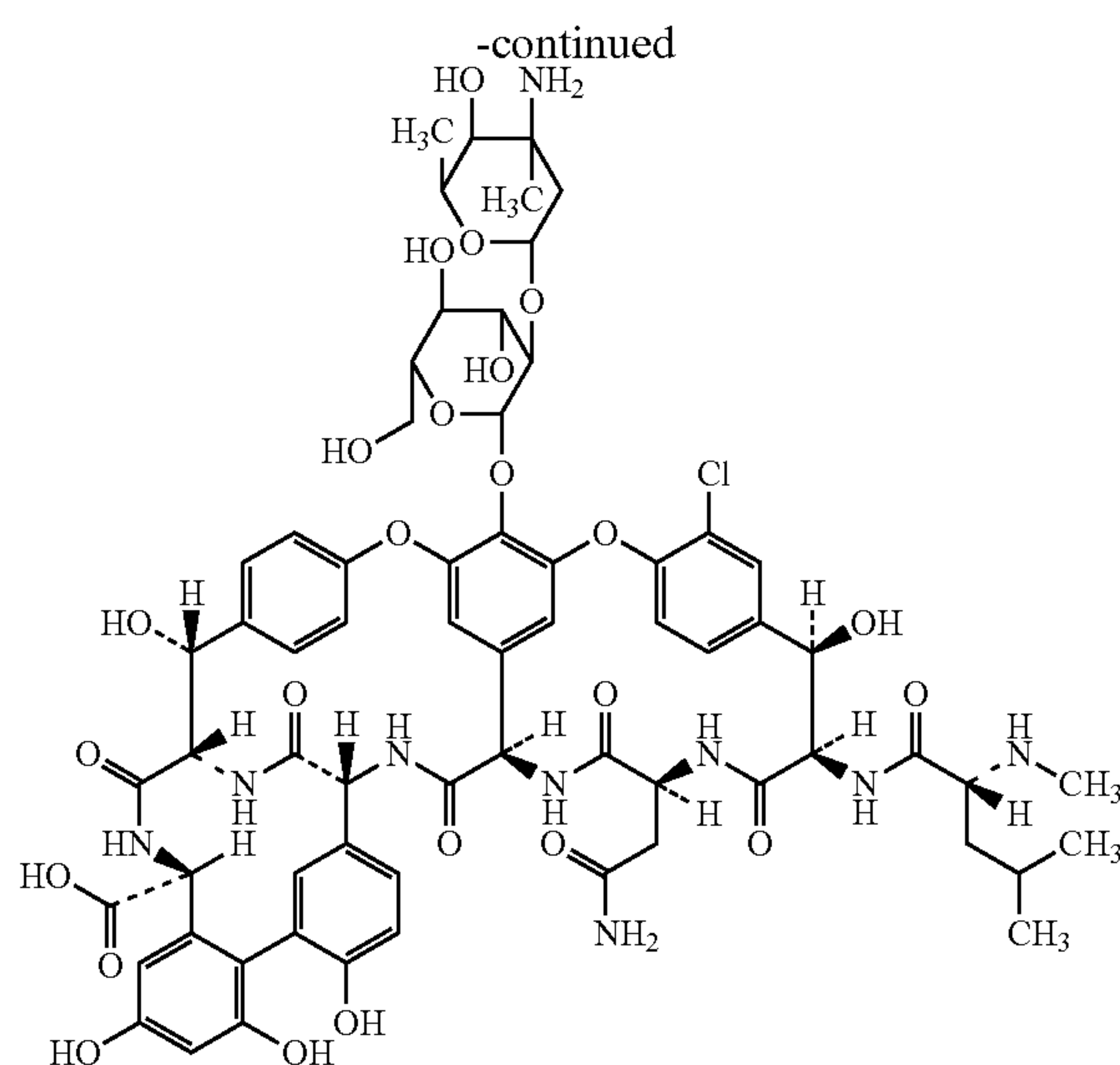
Monodechlorovancomycin
