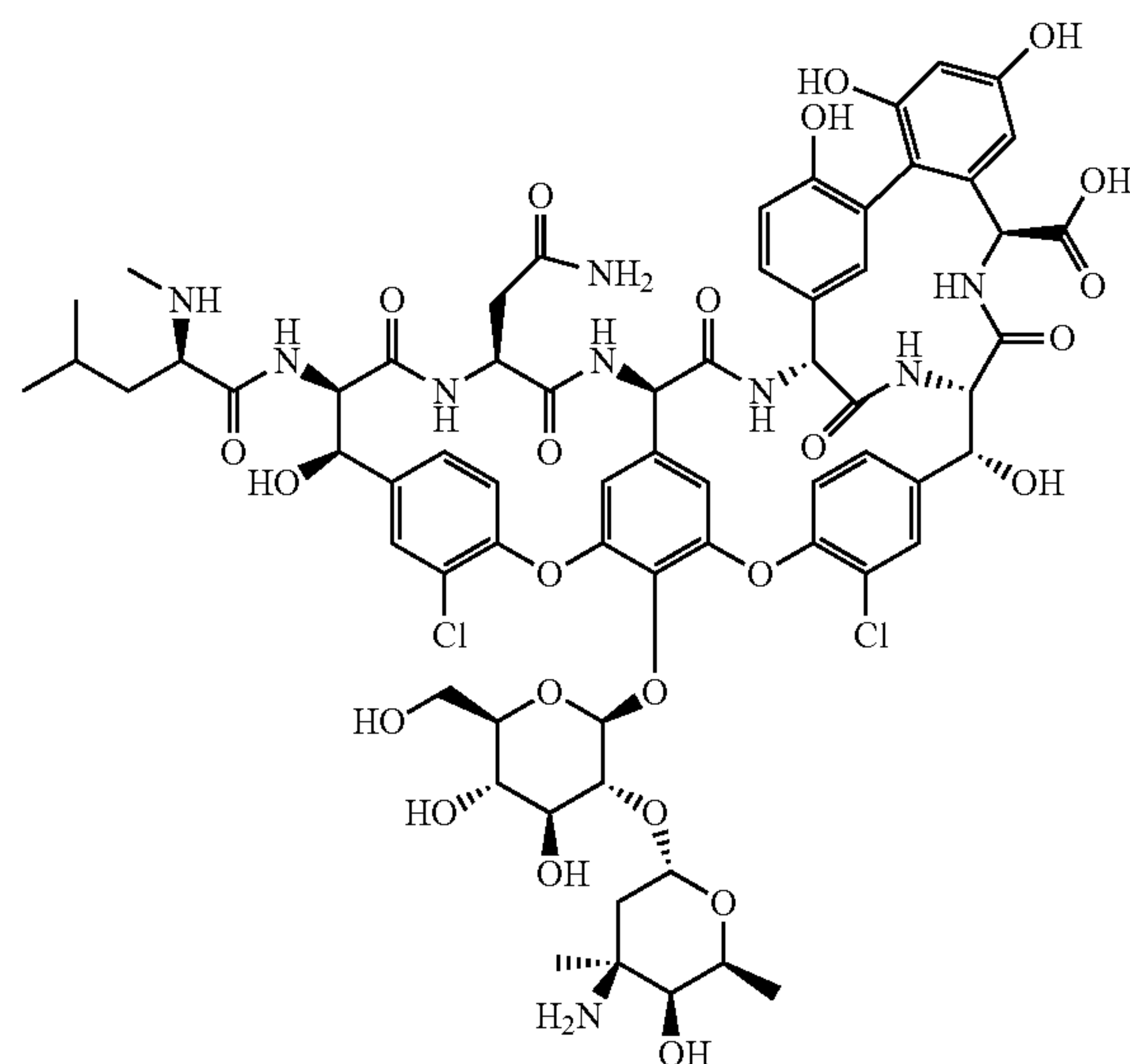
Vancomycin
