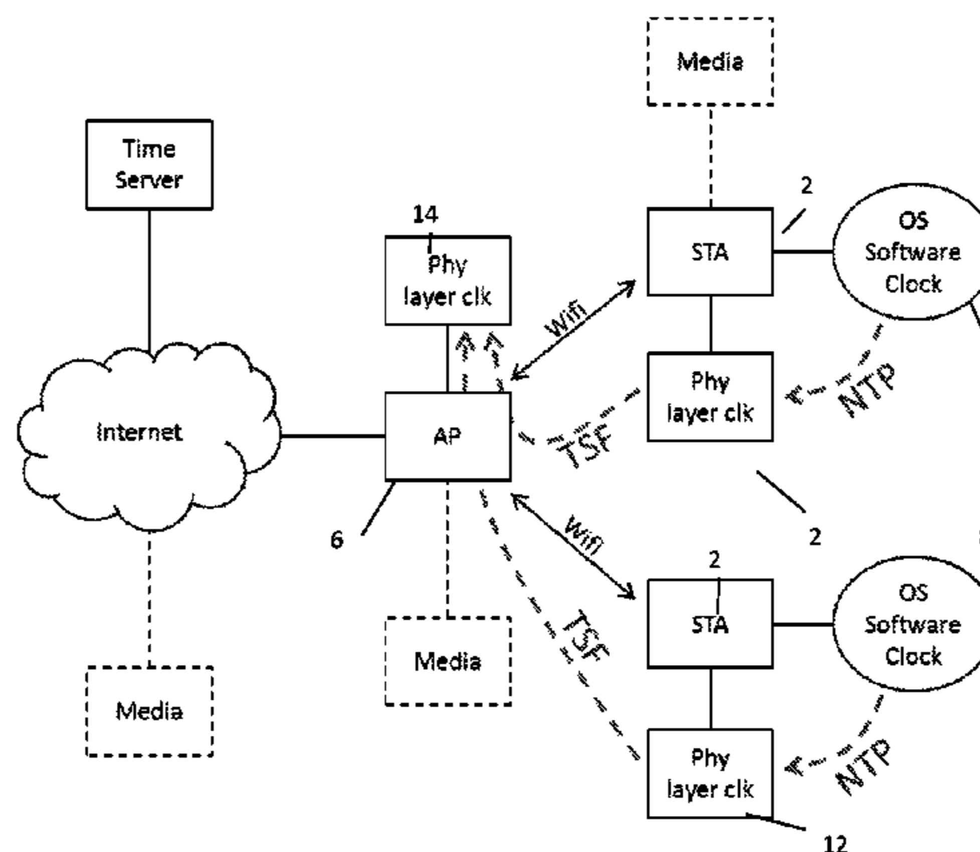
Multiple-protocol layer synchronisation technique
