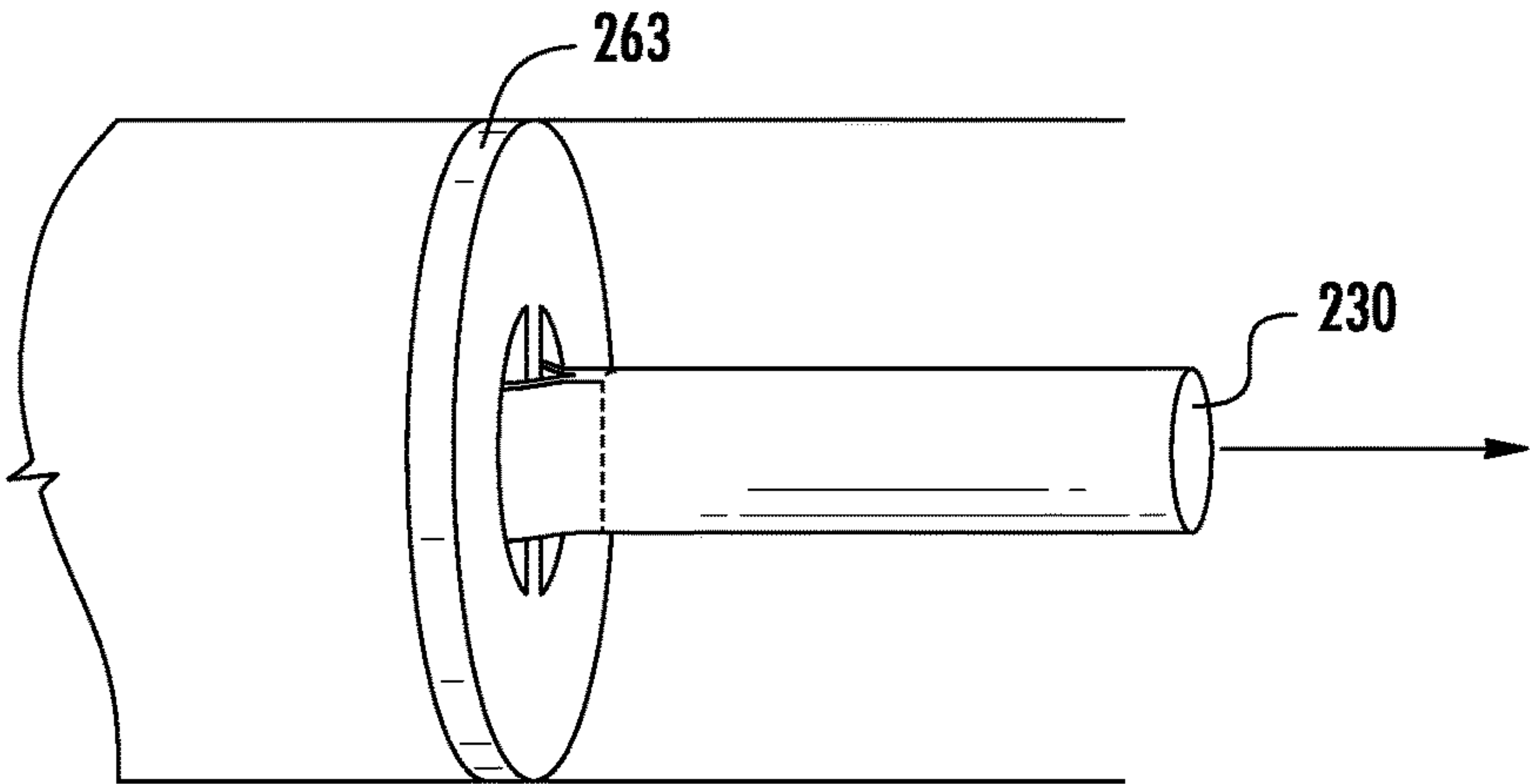
FIG. 2C
