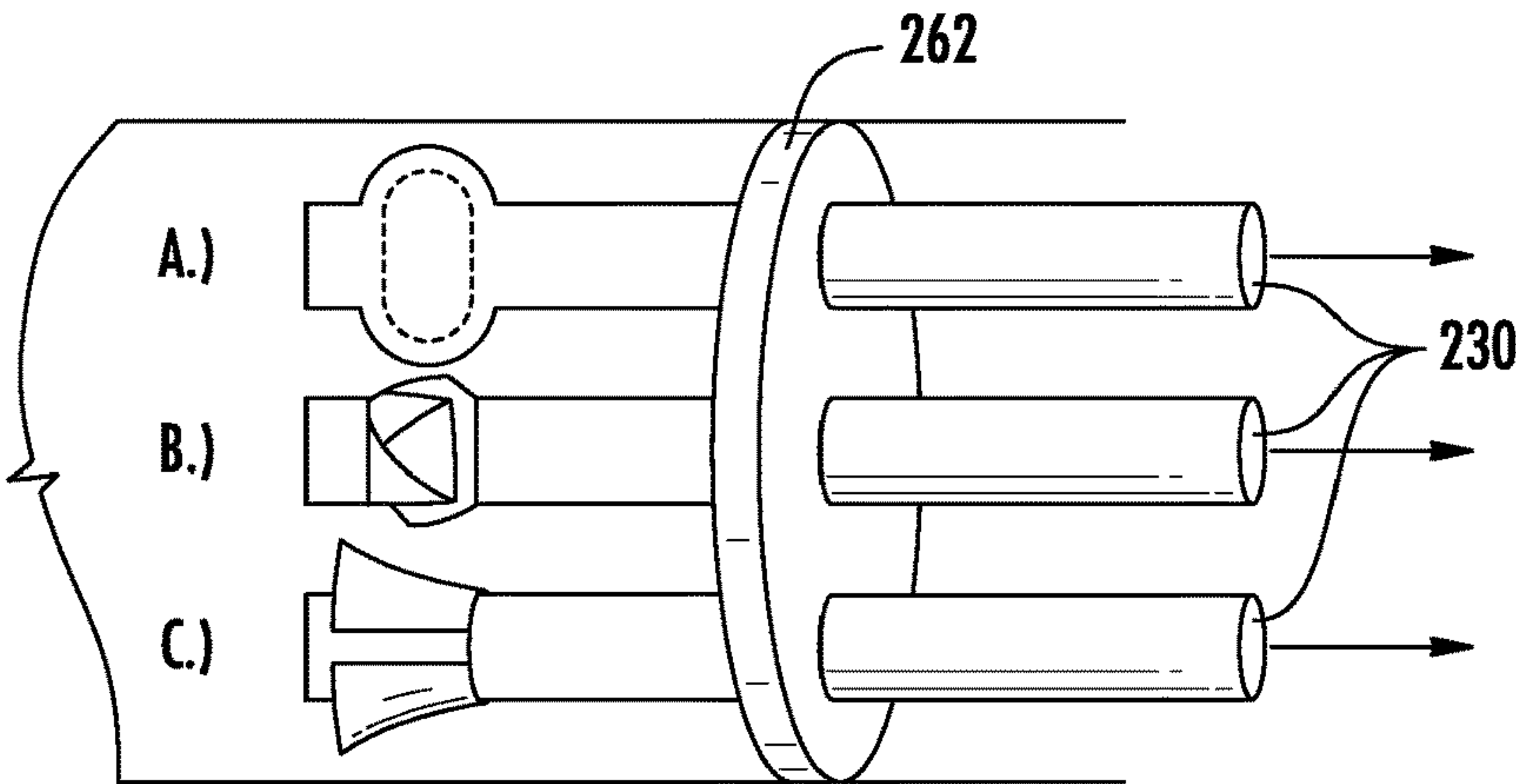
FIG. 2B
