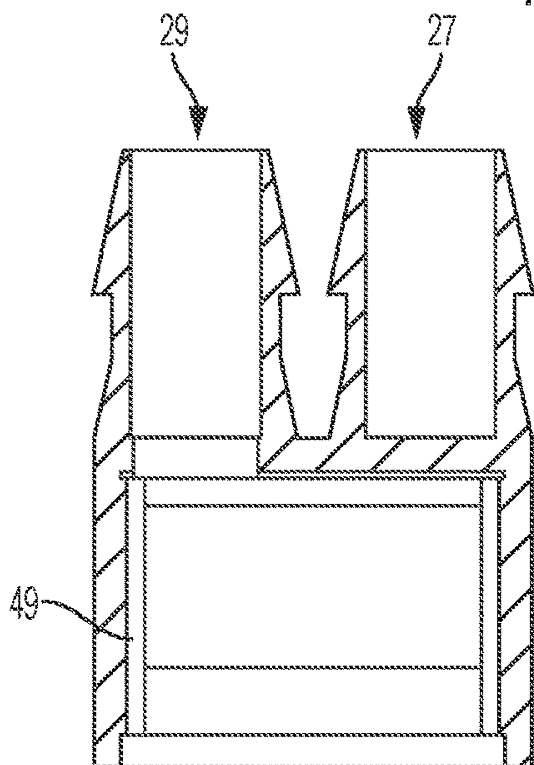
SECTION D-D
