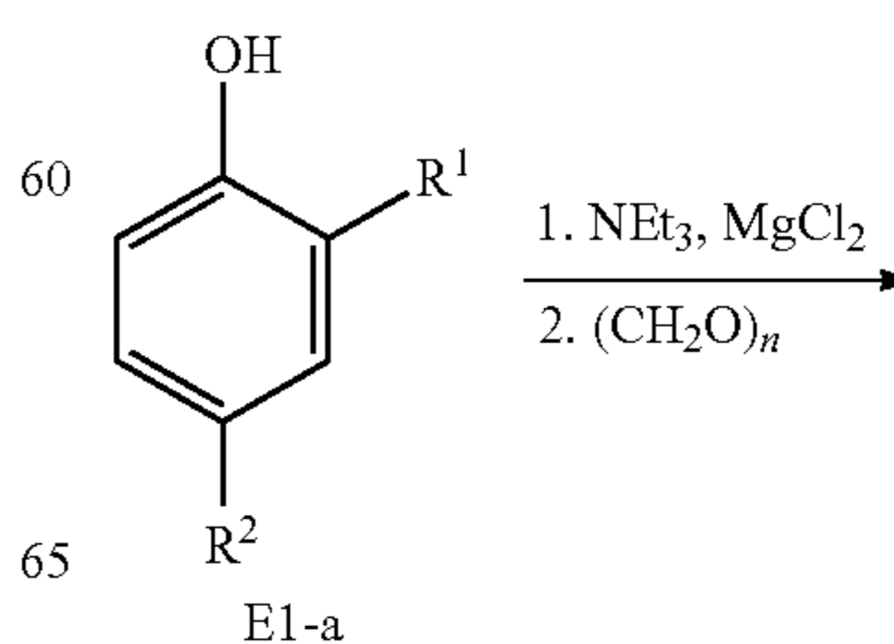
Scheme E1
