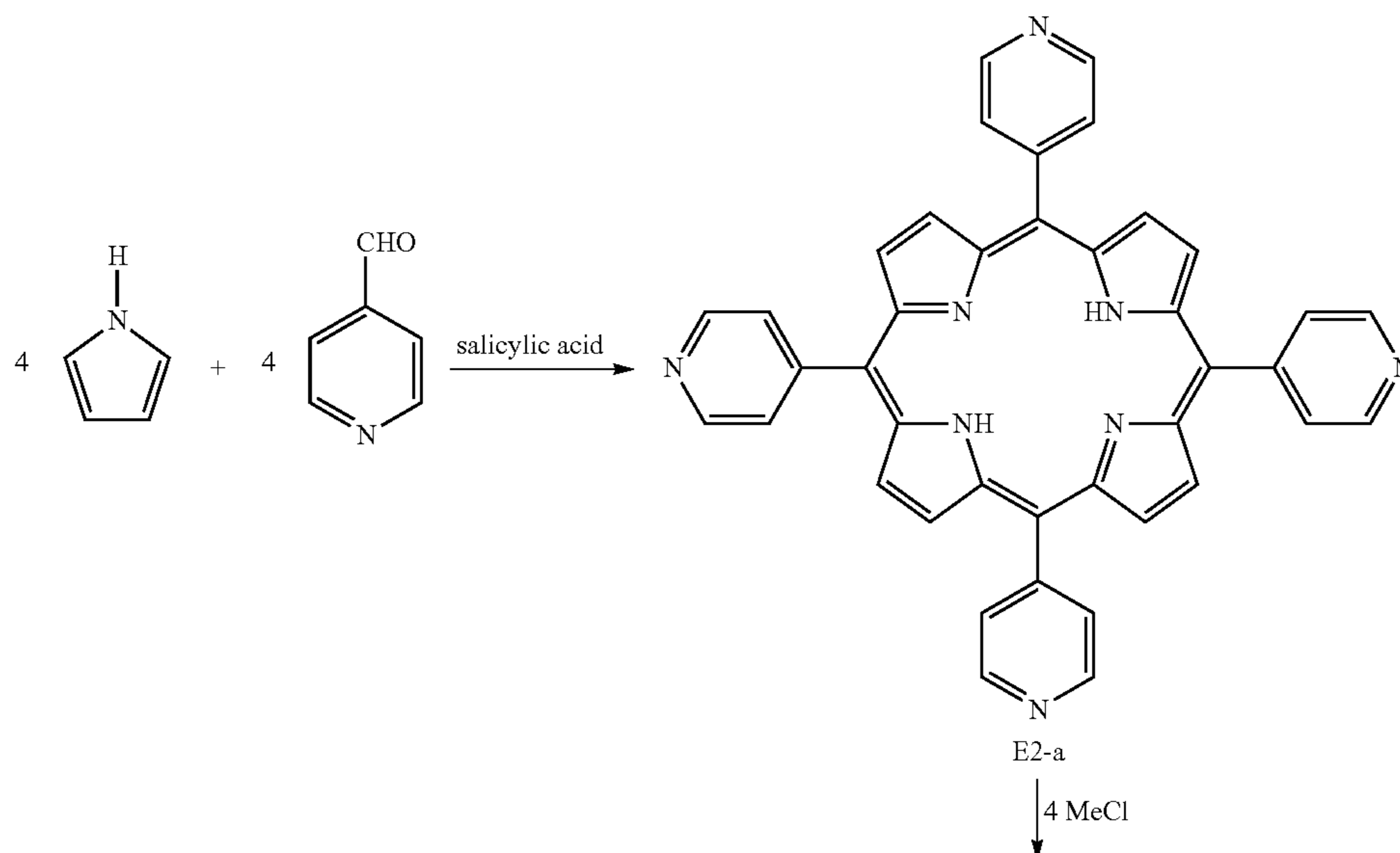
Scheme E2
