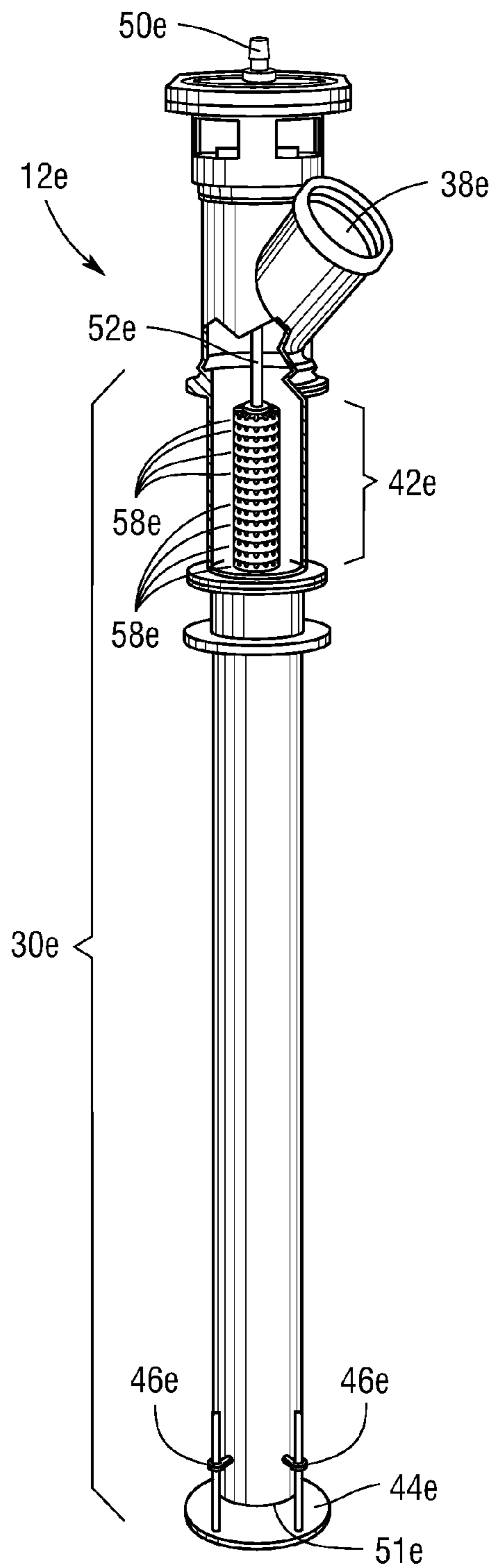
Fig. 7B
