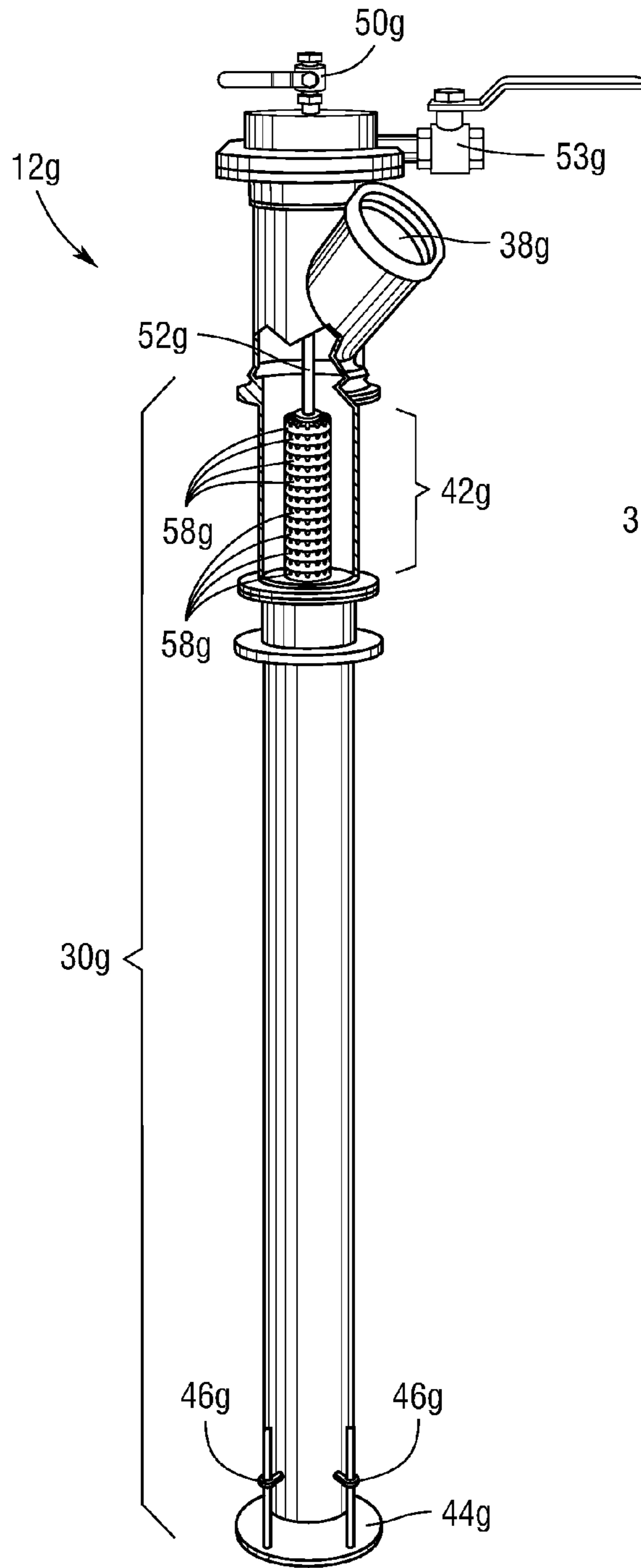
Fig. 9A
