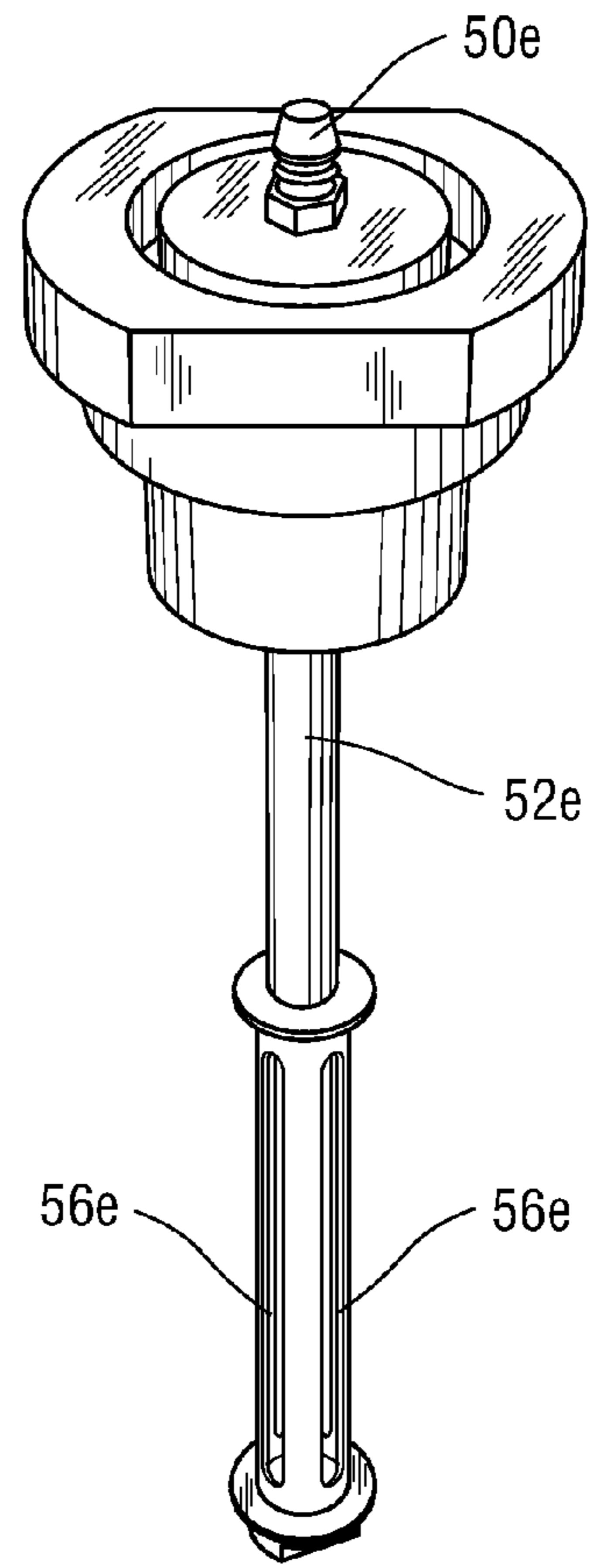
Fig. 7D
