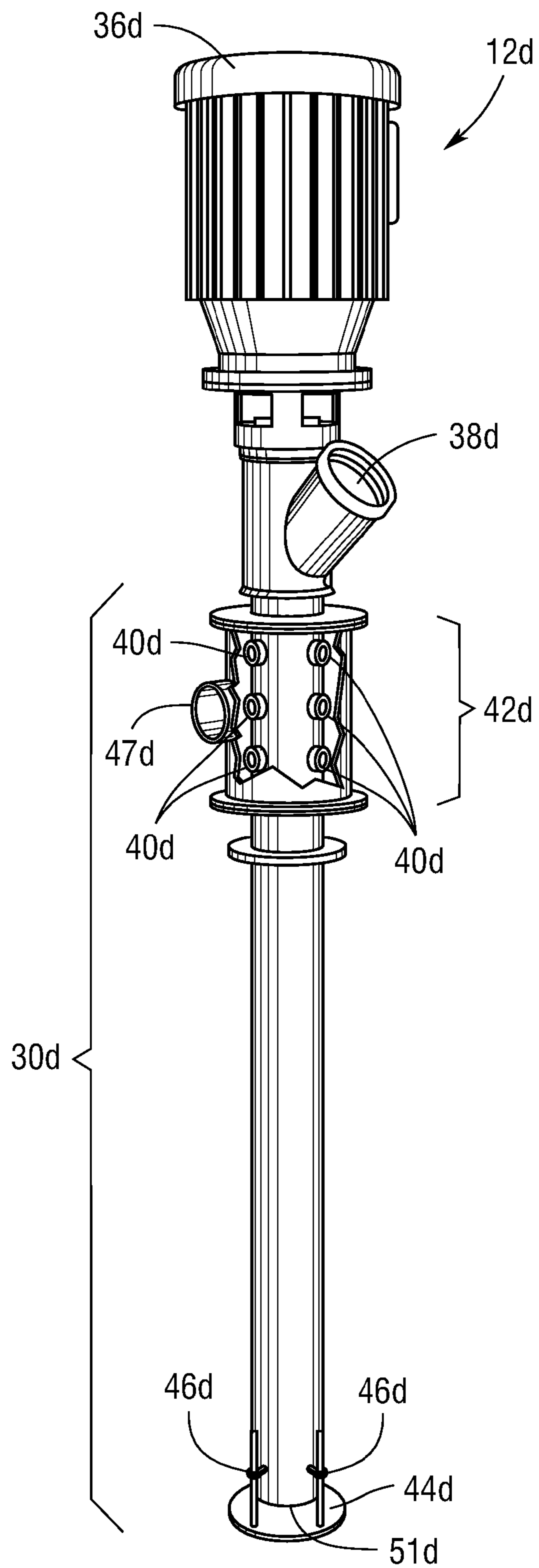
Fig. 6A
