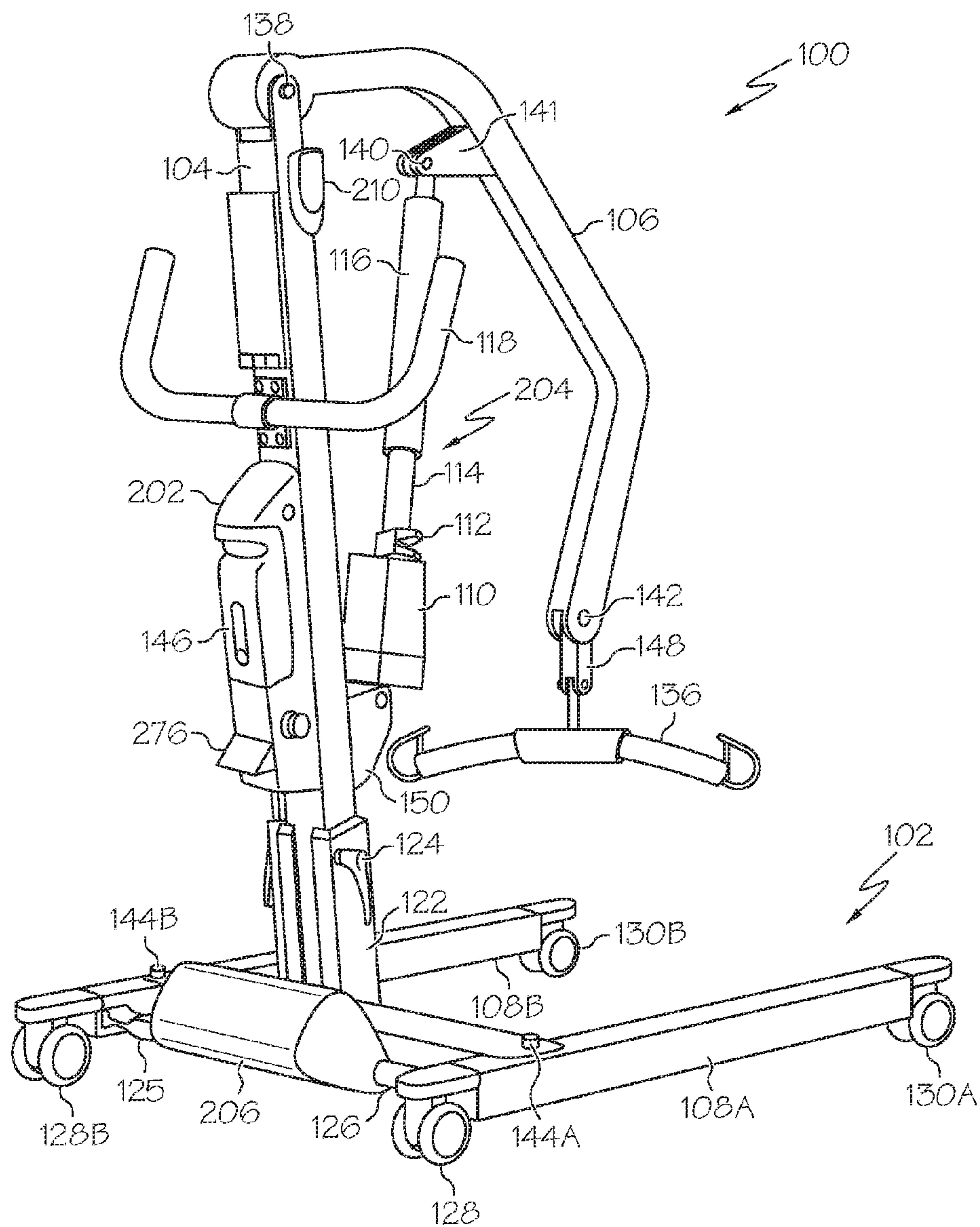
FIG. 1B
