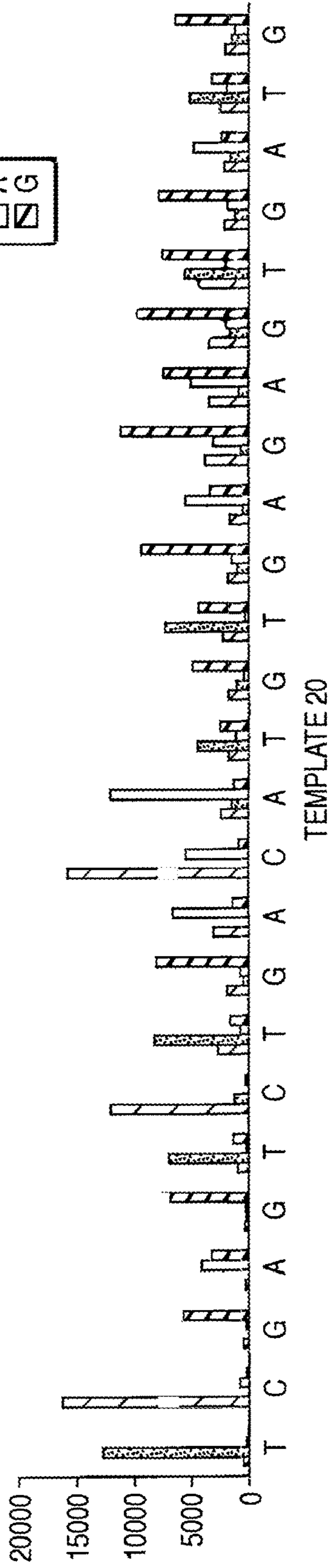
FIG. 24A SEQ ID NO 6
