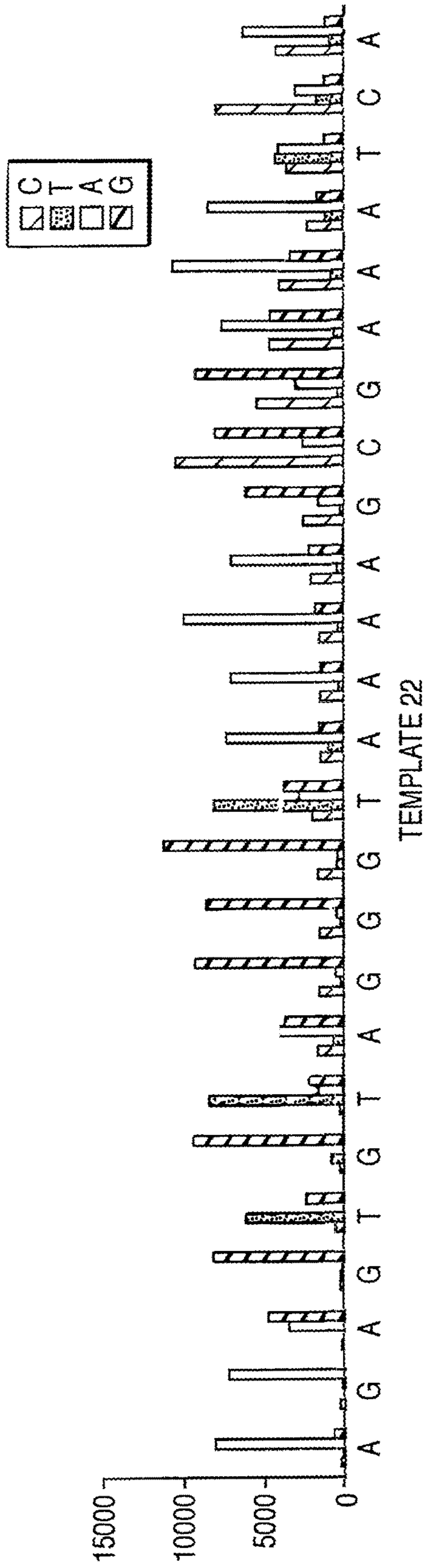
FIG. 24C SEQ ID NO 8
