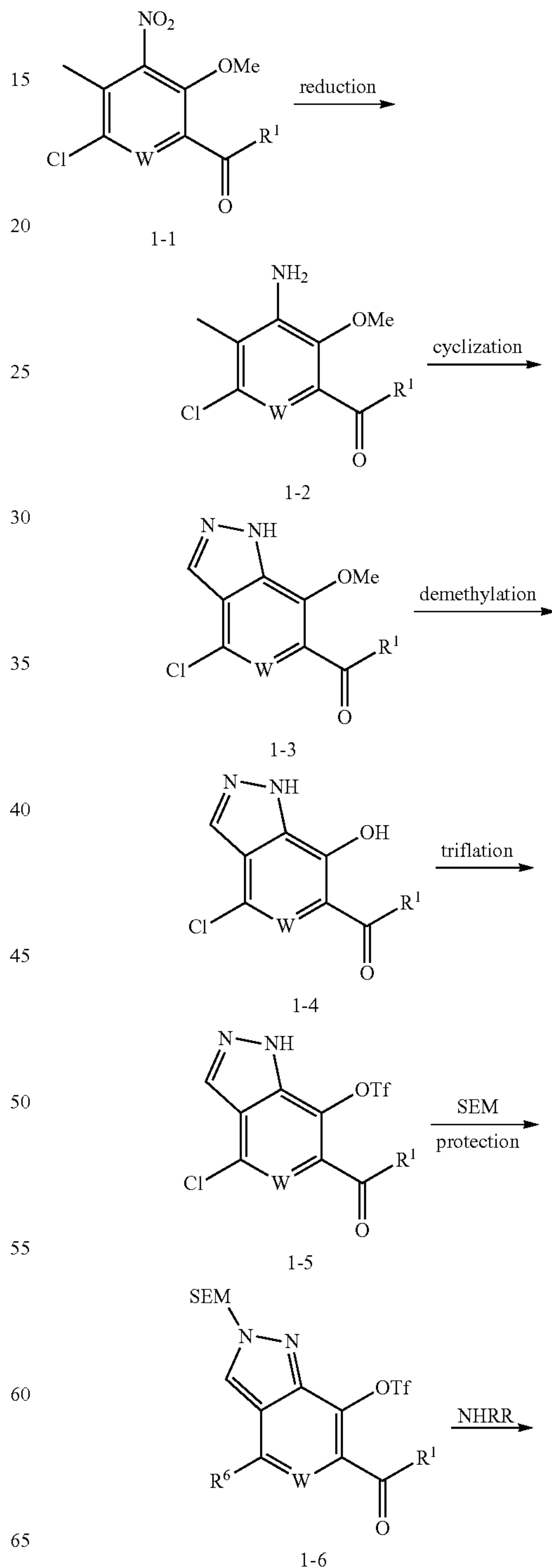
Scheme 14.
