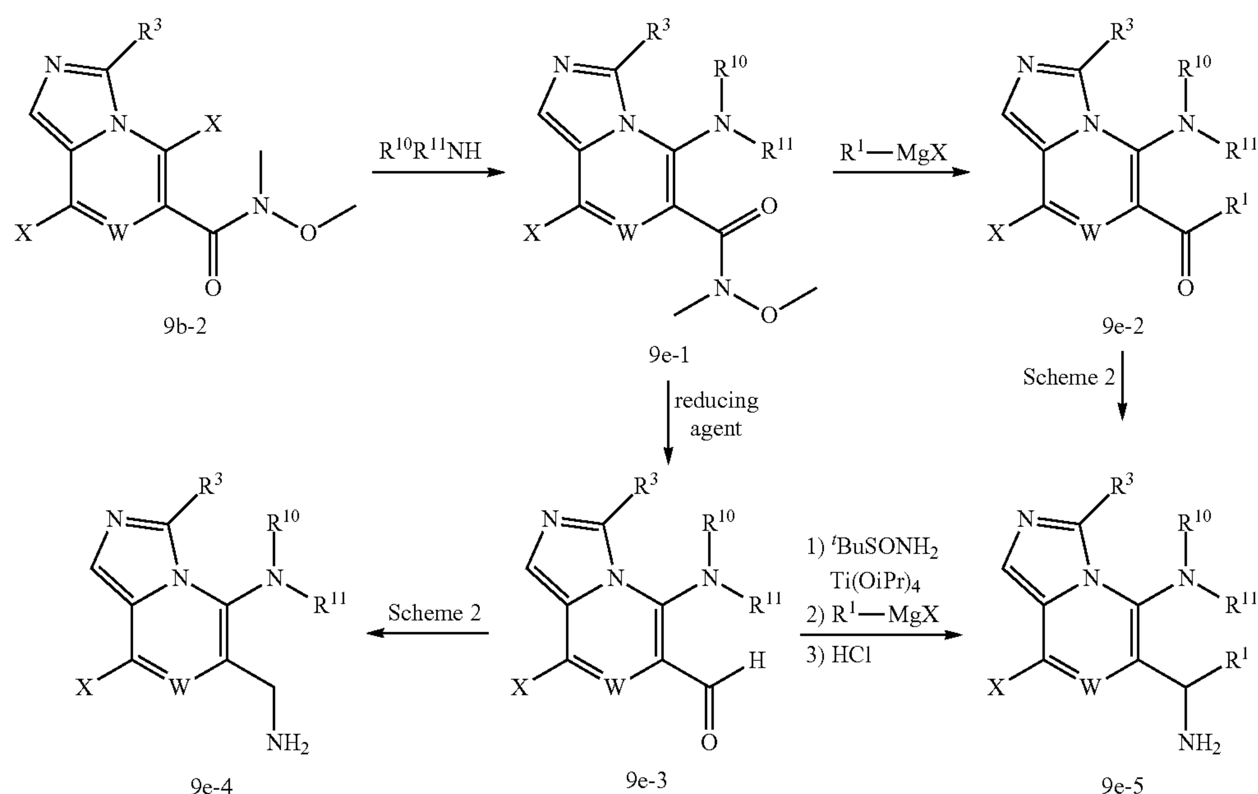
Scheme 9e.
