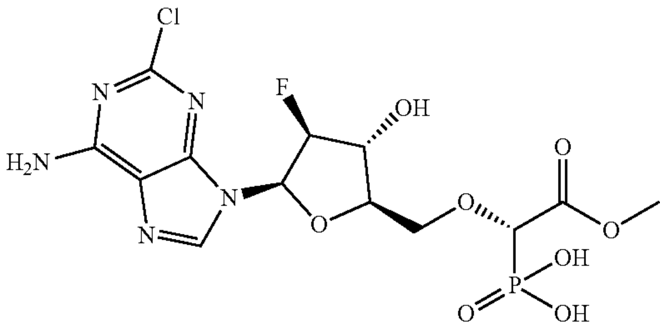
((S)-1-(((2R,3R,4S,5R)-5-(6-amino-2-chloro-9H-purin-9-yl)-4-fluoro-3-hydroxytetrahydrofuran-2-yl)methoxy)-2-methoxy-2-oxoethyl)phosphonic acid;
