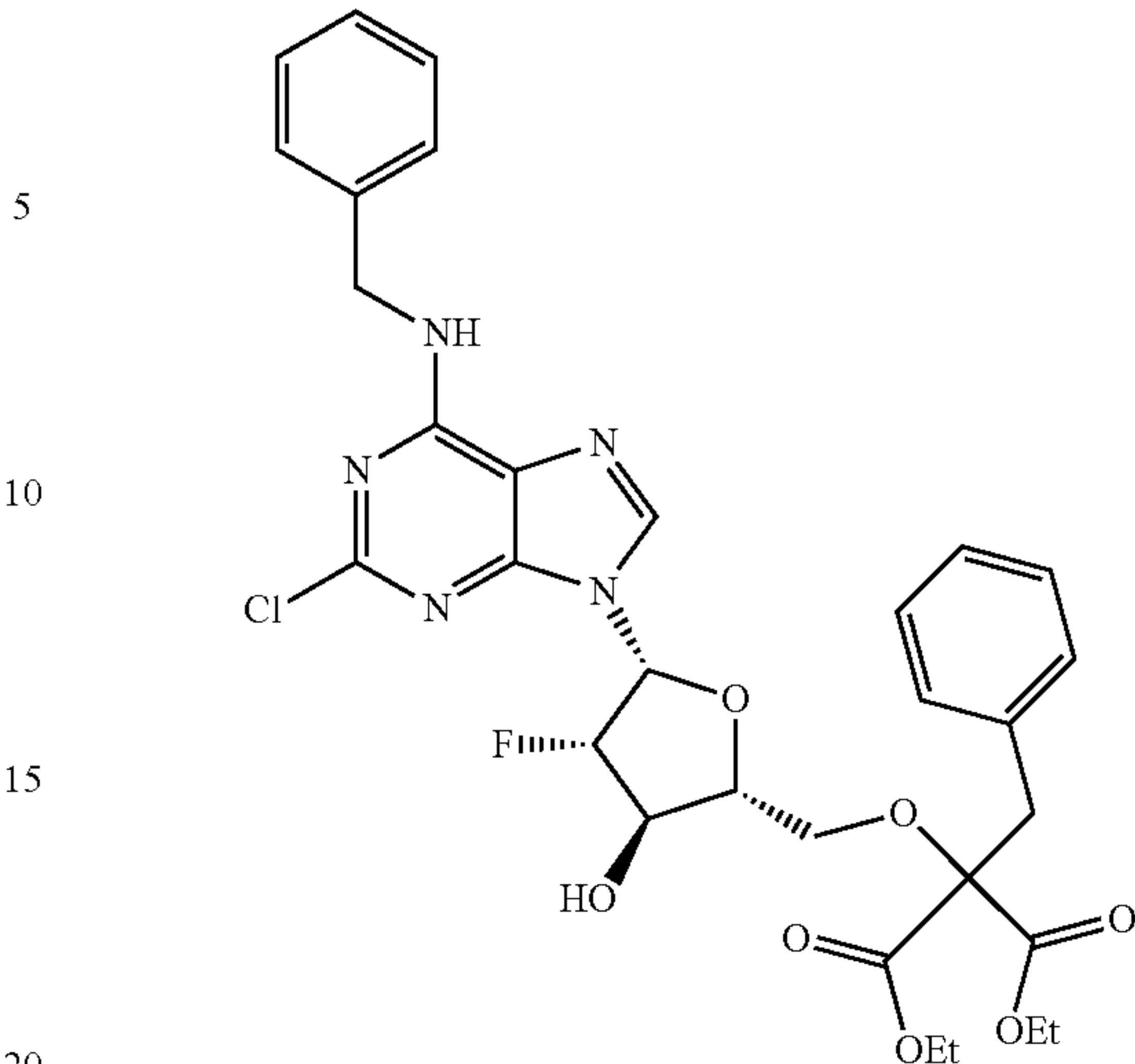
diethyl 2-benzyl-2-(((2R,3R,4S,5R)-5-(6-(benzylamino)-2-chloro-9H-purin-9-yl)-4-fluoro-3-hydroxytetrahydrofuran-2-yl)methoxy)malonate;
