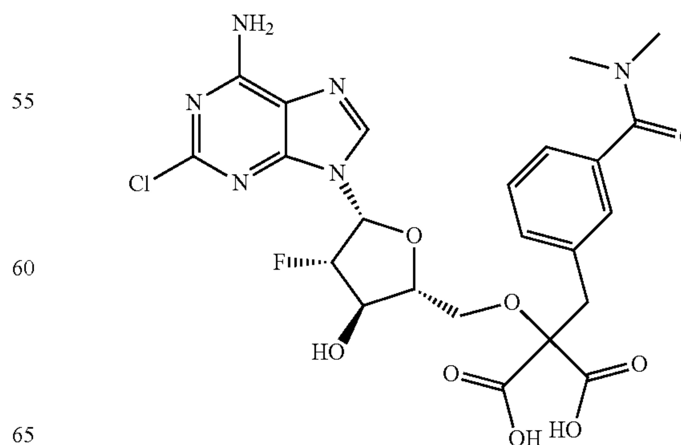
diethyl 2-(((2R,3R,4S,5R)-5-(6-amino-2-chloro-9H-purin-9-yl)-4-fluoro-3-hydroxytetrahydrofuran-2-yl)methoxy)-2-(4-(methylsulfonyl)benzyl)malonate;
