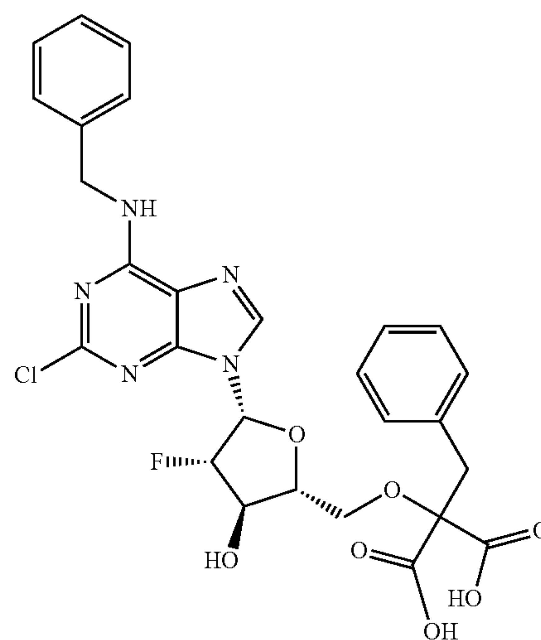
2-benzyl-2-(((2R,3R,4S,5R)-5-(6-(benzylamino)-2-chloro-9H-purin-9-yl)-4-fluoro-3-hydroxytetrahydrofuran-2-yl)methoxy)malonic acid;
