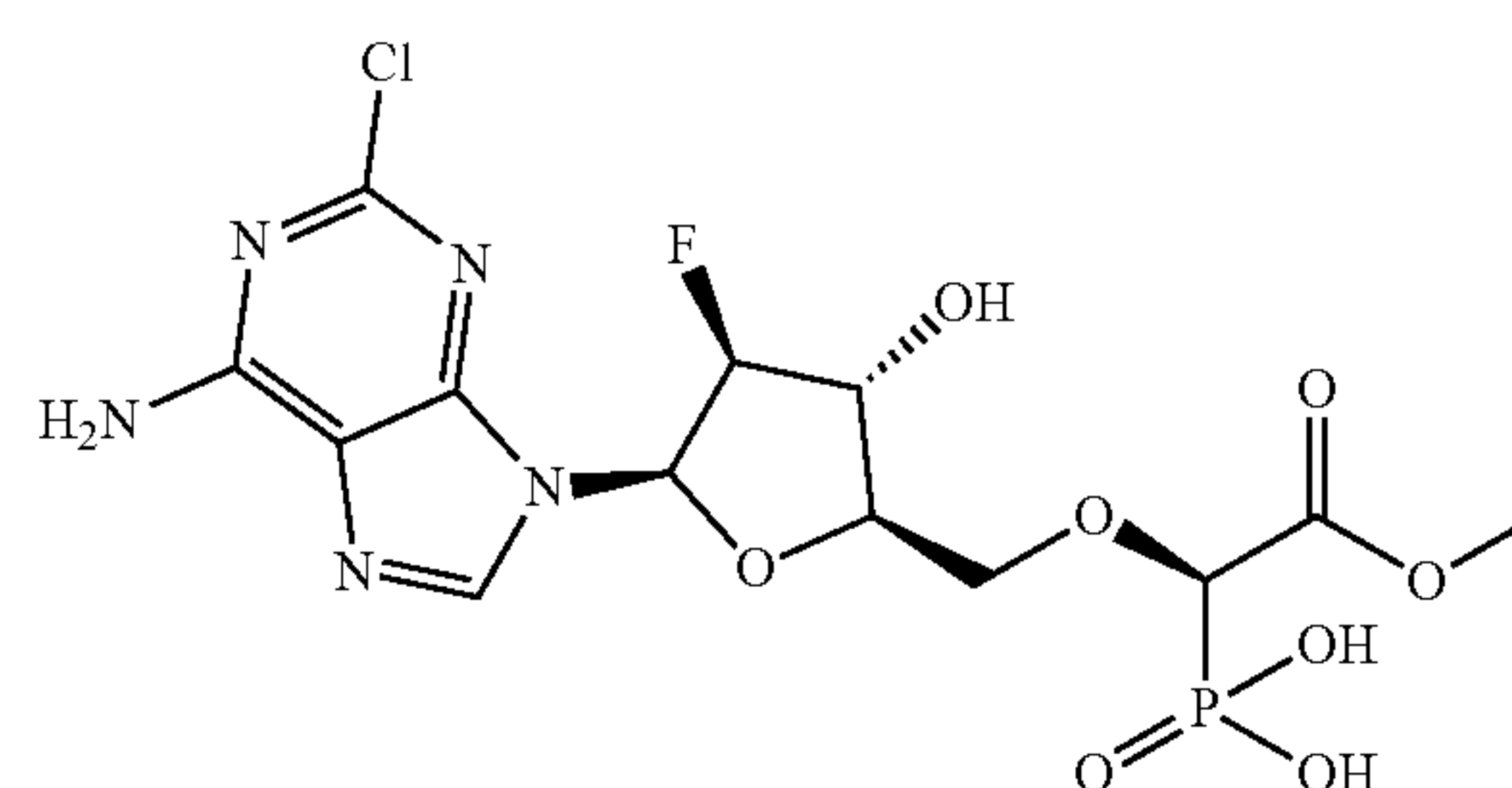
((R)-1-(((2R,3R,4S,5R)-5-(6-amino-2-chloro-9H-purin-9-yl)-4-fluoro-3-hydroxytetrahydrofuran-2-yl)methoxy)-2-methoxy-2-oxoethyl)phosphonic acid;
