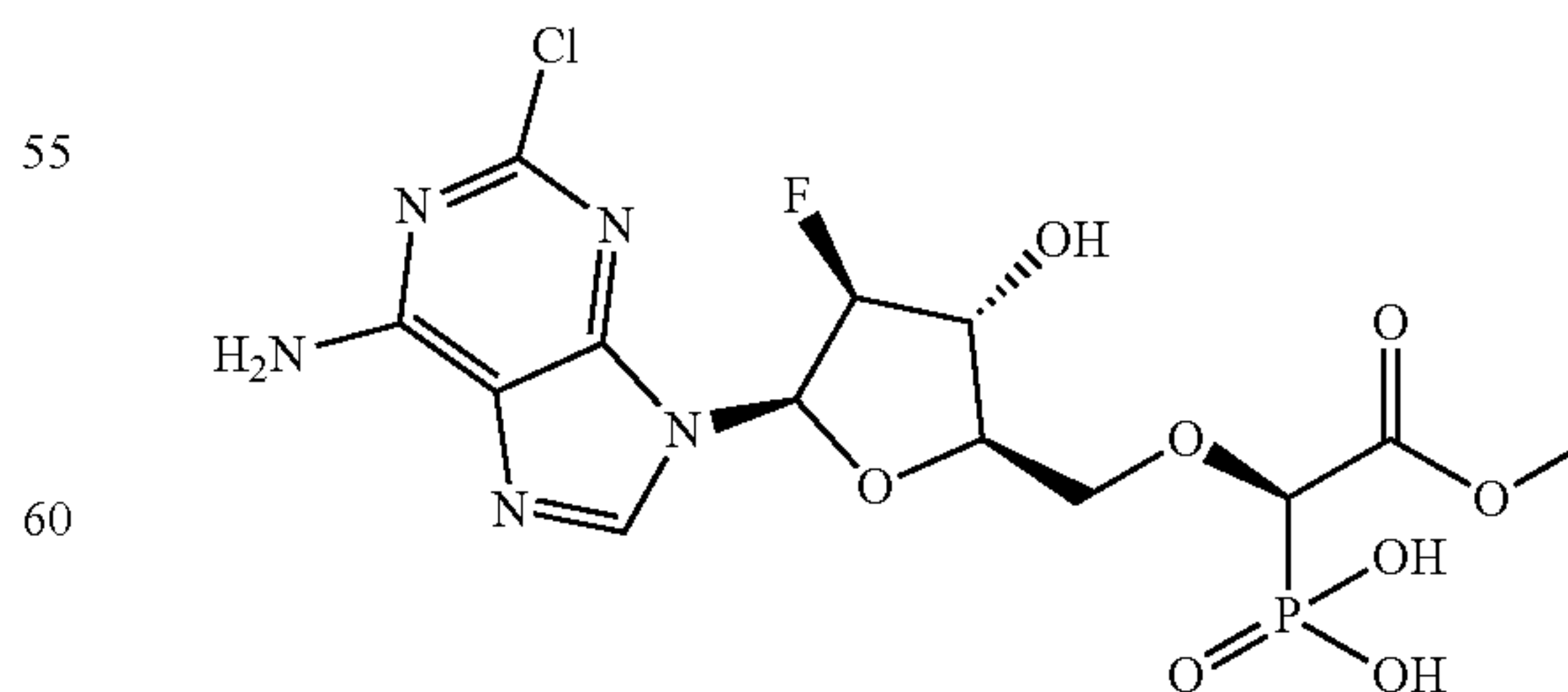
((R)-1-(((2R,3R,4S,5R)-5-(6-amino-2-chloro-9H-purin-9-yl)-4-fluoro-3-hydroxytetrahydrofuran-2-yl)methoxy)-2-methoxy-2-oxoethyl)phosphonic acid;
