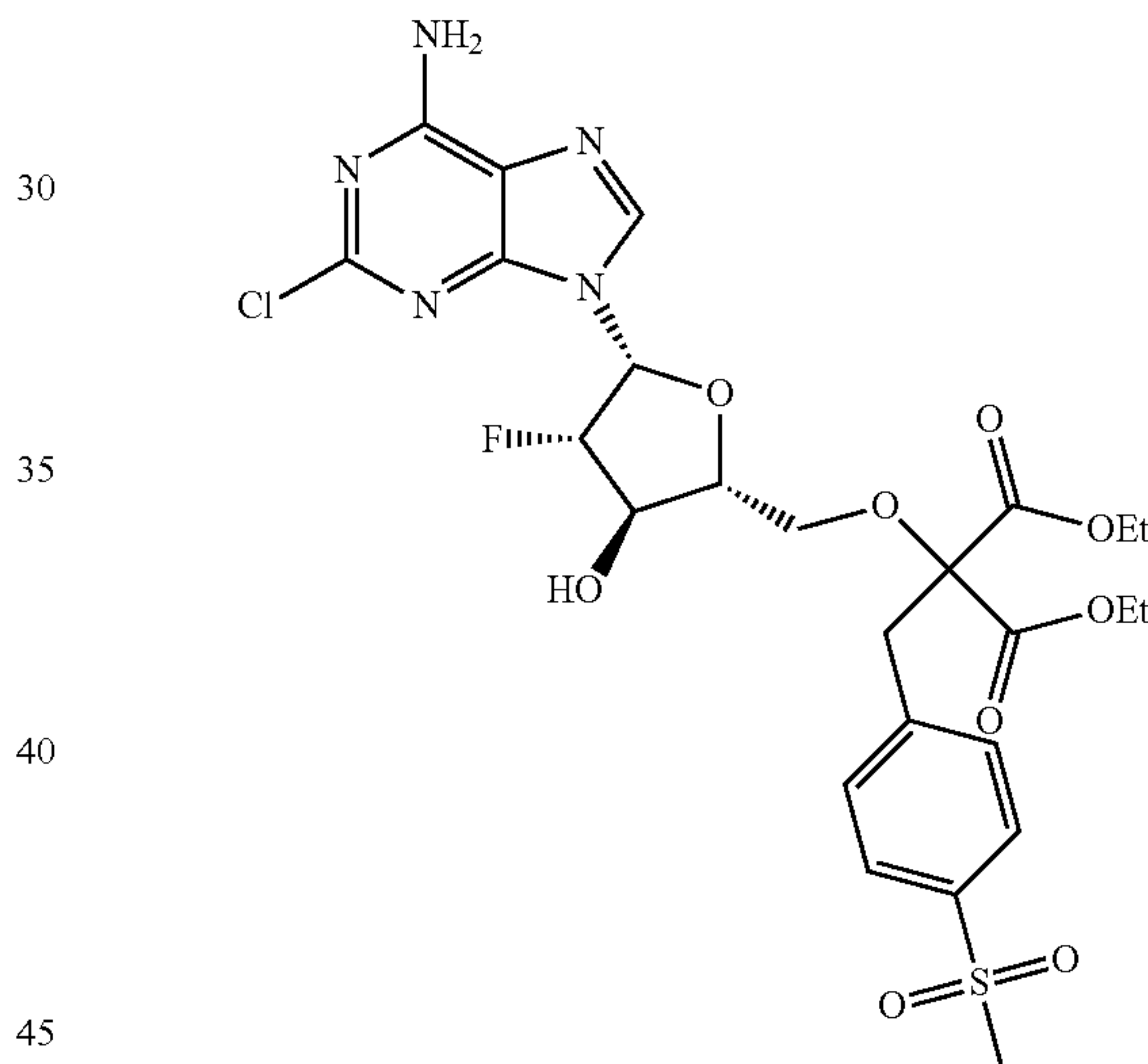
diethyl 2-(((2R,3R,4S,5R)-5-(6-amino-2-chloro-9H-purin-9-yl)-4-fluoro-3-hydroxytetrahydrofuran-2-yl)methoxy)-2-(4-(methylsulfonyl)benzyl)malonate;
