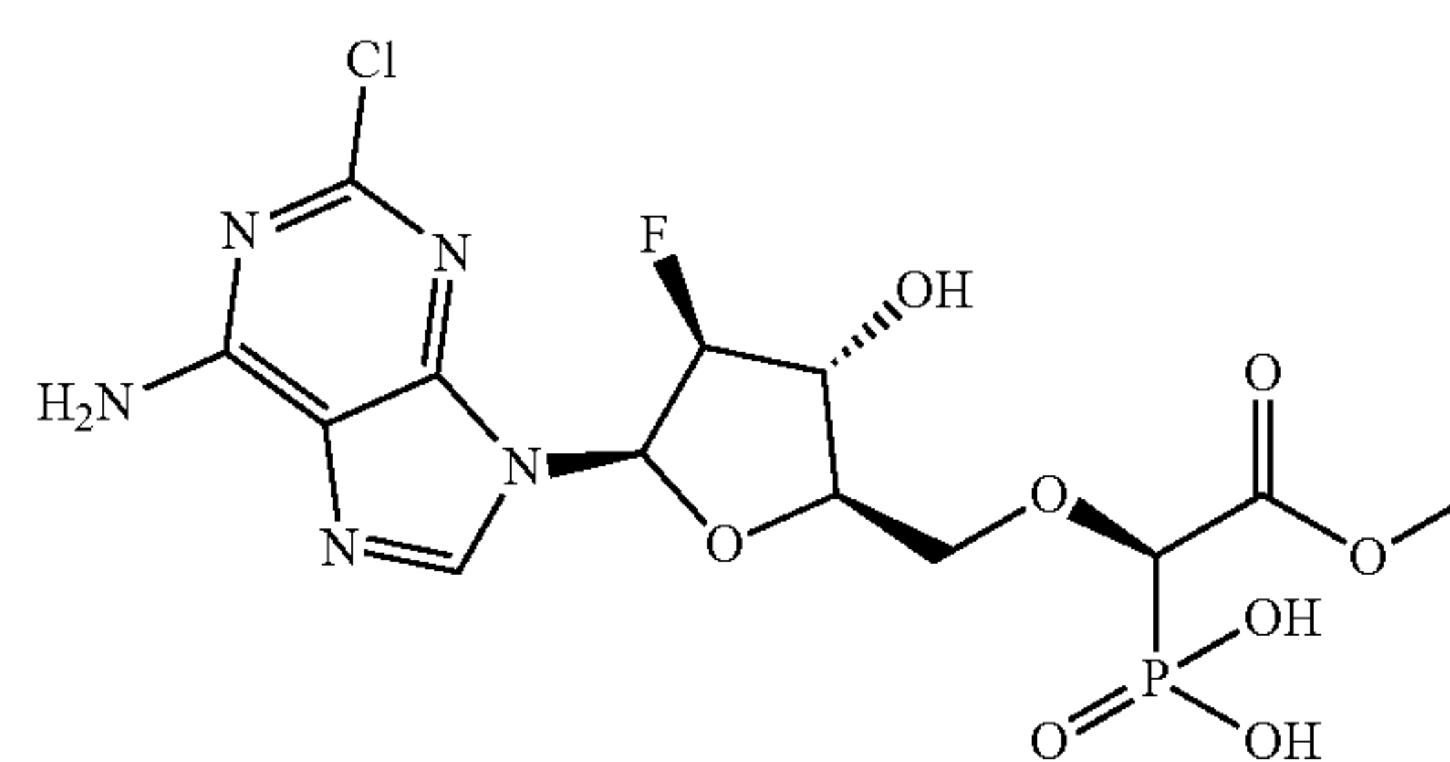
((R)-1-(((2R,3R,4S,5R)-5-(6-amino-2-chloro-9H-purin-9-yl)-4-fluoro-3-hydroxytetrahydrofuran-2-yl)methoxy)-2-methoxy-2-oxoethyl)phosphonic acid;
