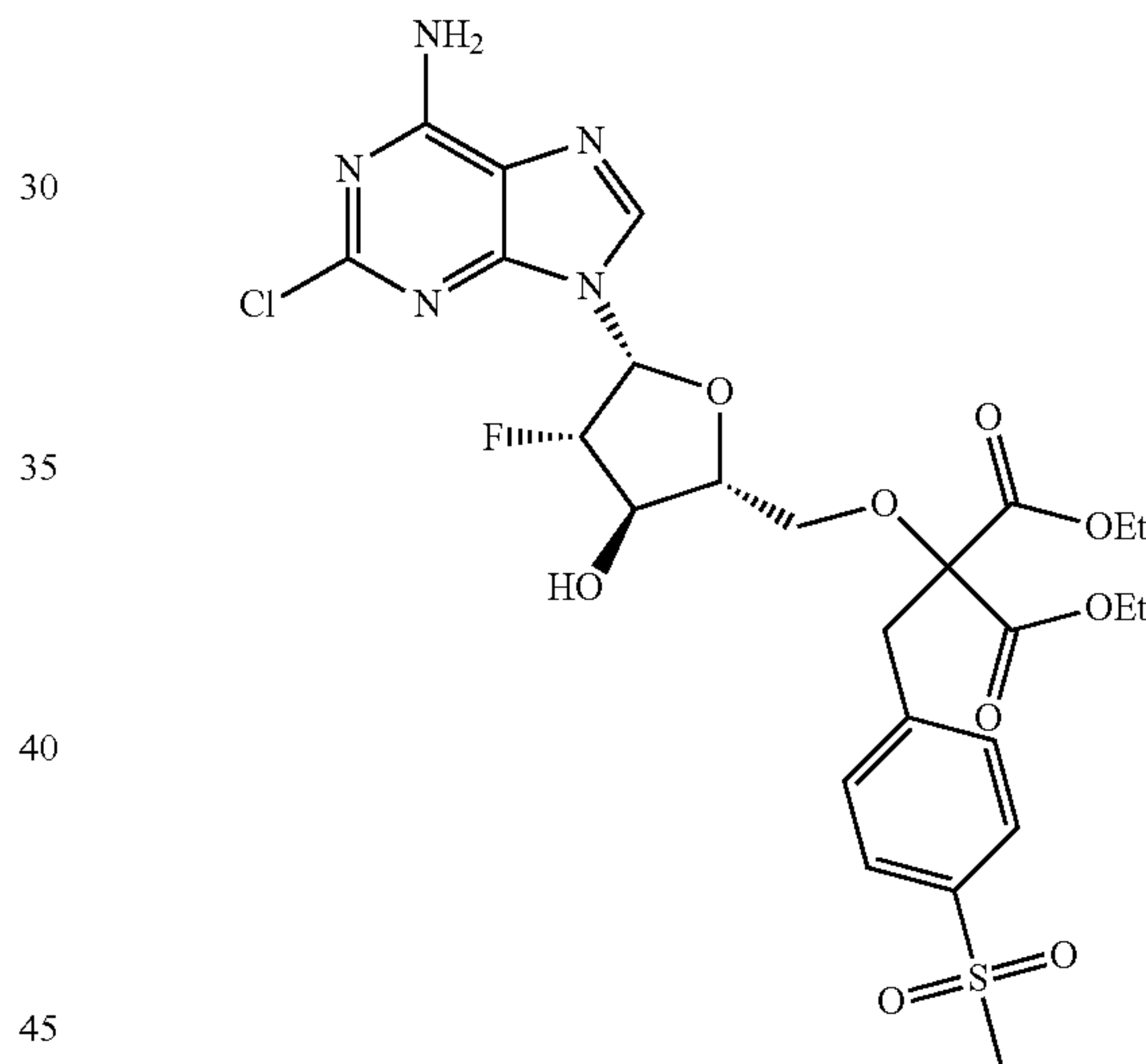
diethyl 2-(((2R,3R,4S,5R)-5-(6-amino-2-chloro-9H-purin-9-yl)-4-fluoro-3-hydroxytetrahydrofuran-2-yl)methoxy)-2-(4-(methylsulfonyl)benzyl)malonate;
