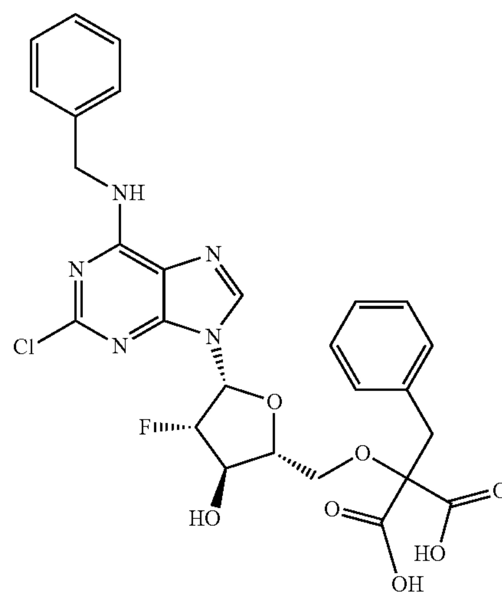
2-benzyl-2-(((2R,3R,4S,5R)-5-(6-(benzylamino)-2-chloro-9H-purin-9-yl)-4-fluoro-3-hydroxytetrahydrofuran-2-yl)methoxy)malonic acid;
