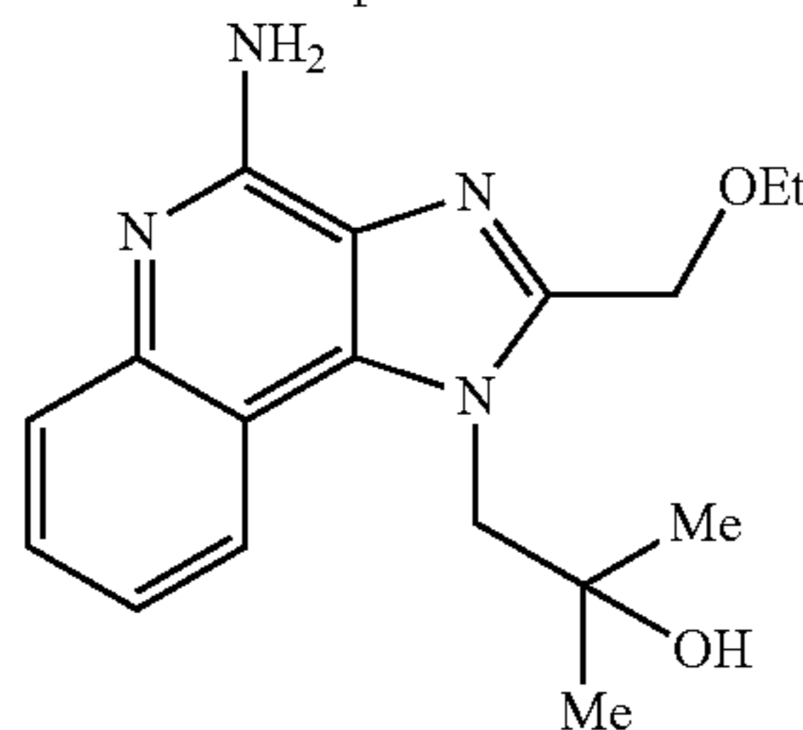
Resiquimod
