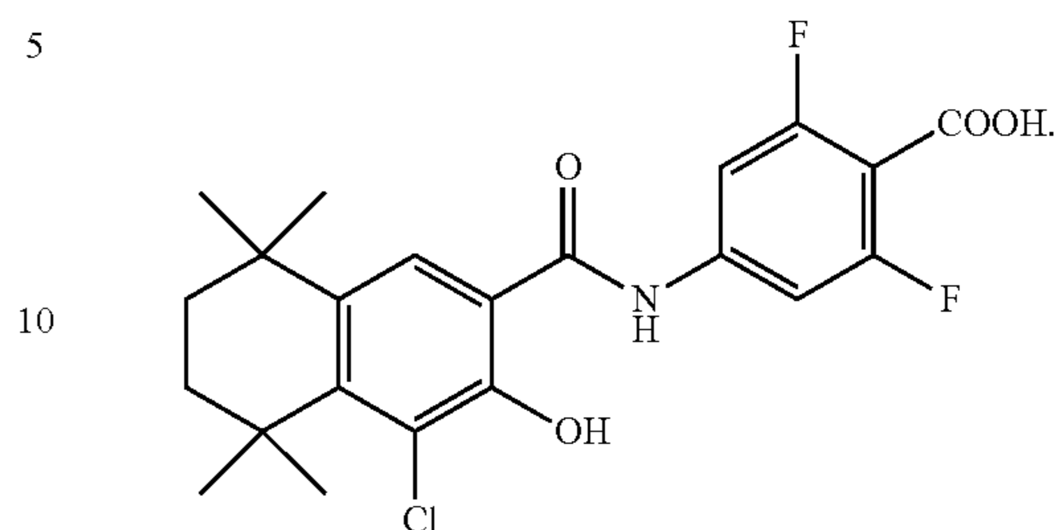
(VII; IRX5183)
