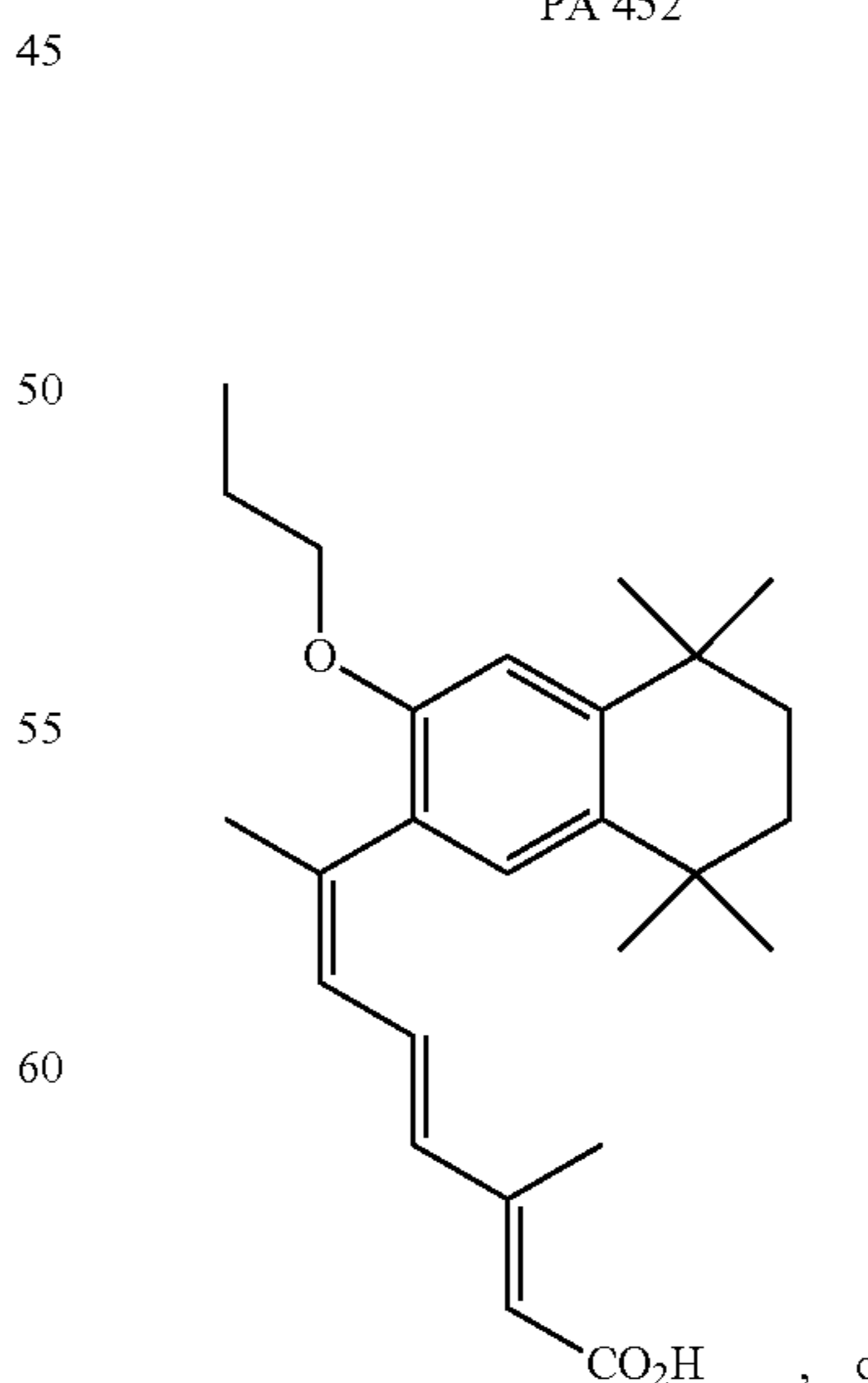
LG 100754
