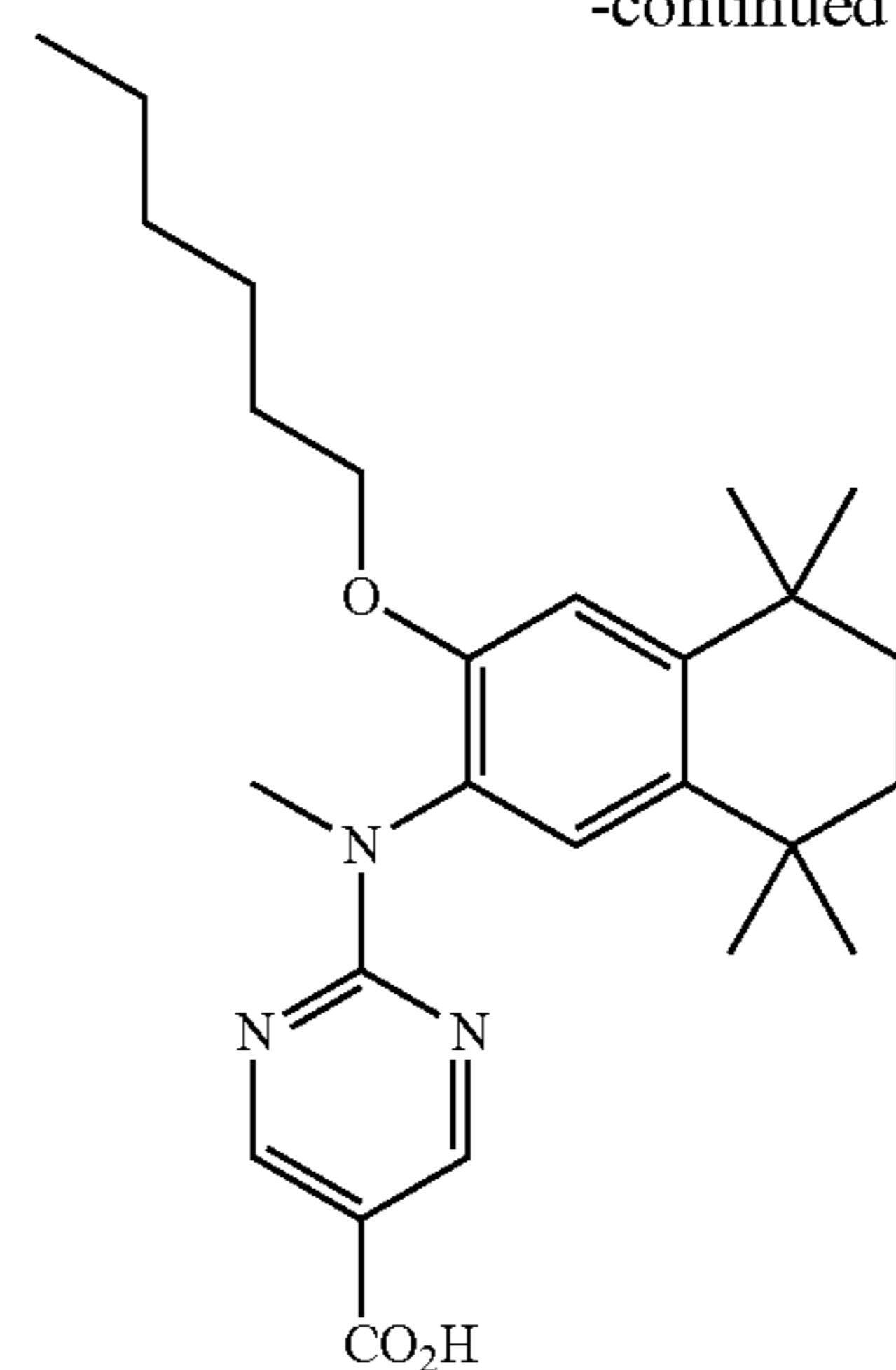
PA 452
