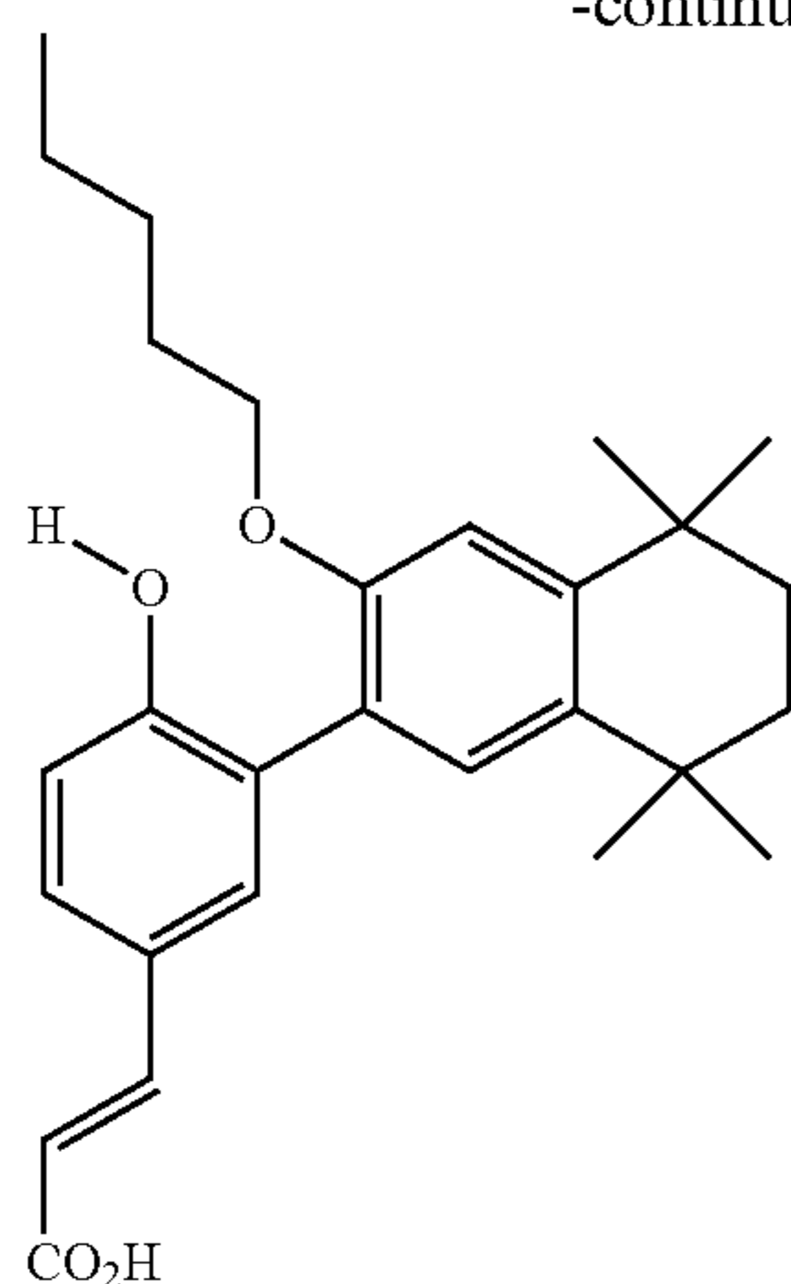
UVI 3003
