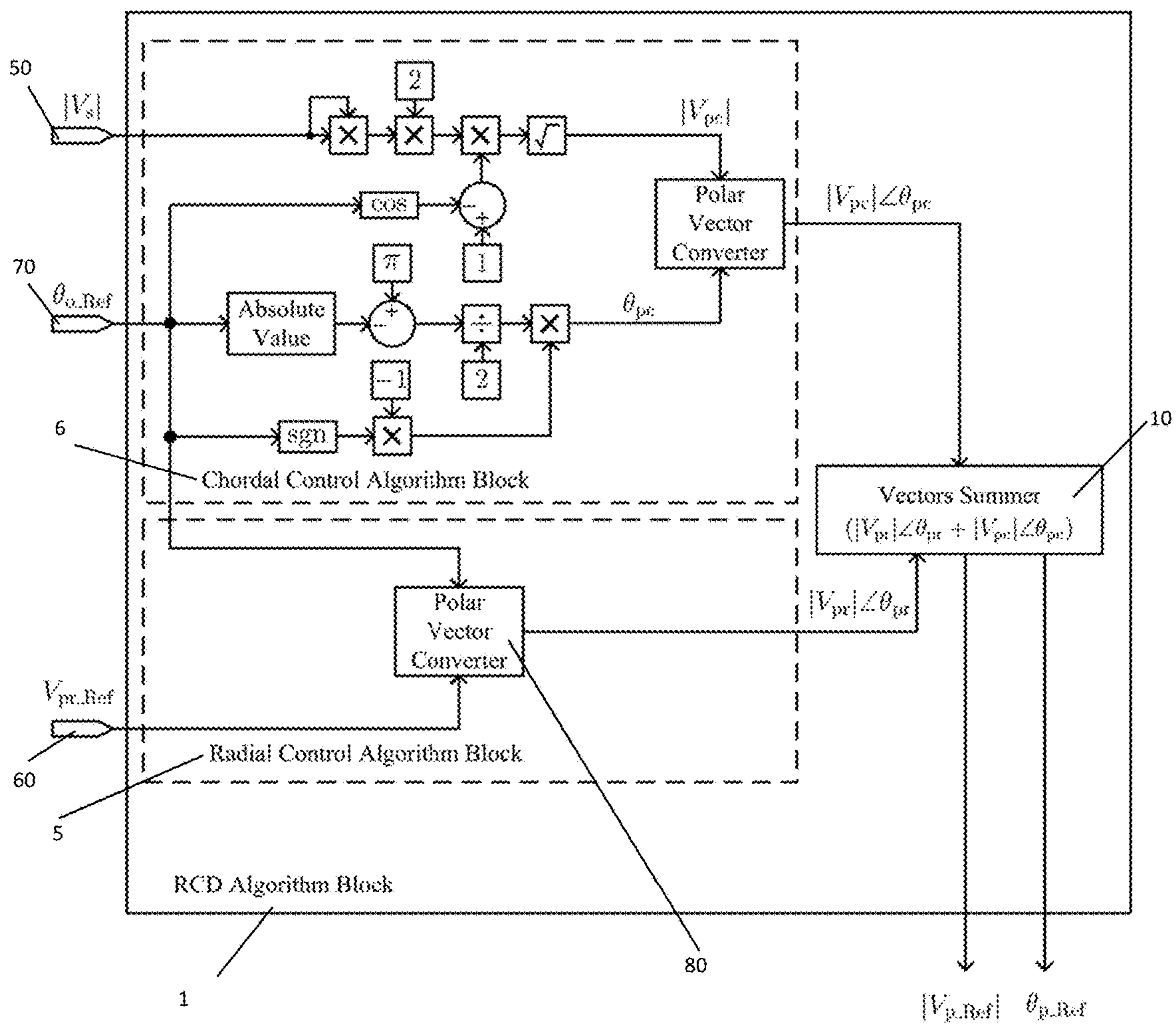
FIG. 10
