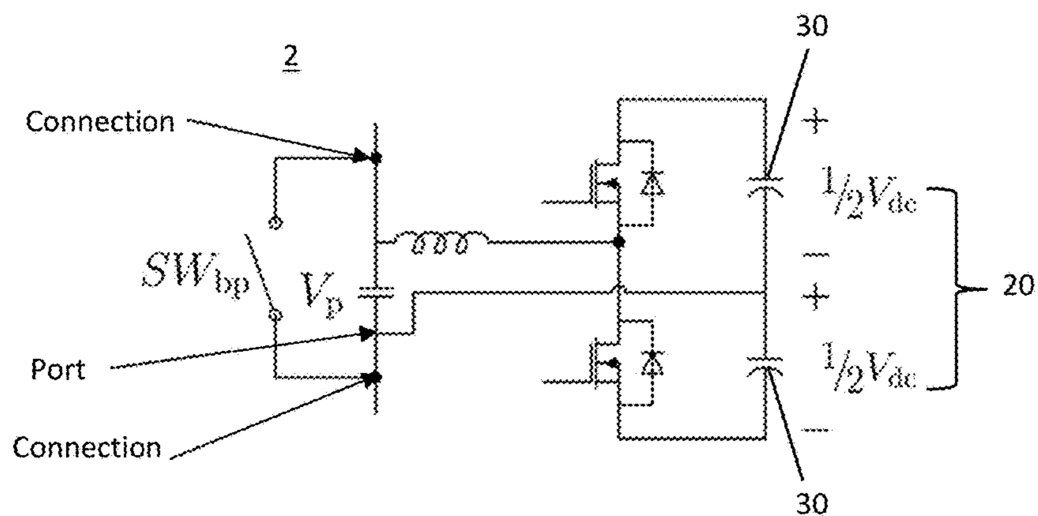
FIG. 7B
