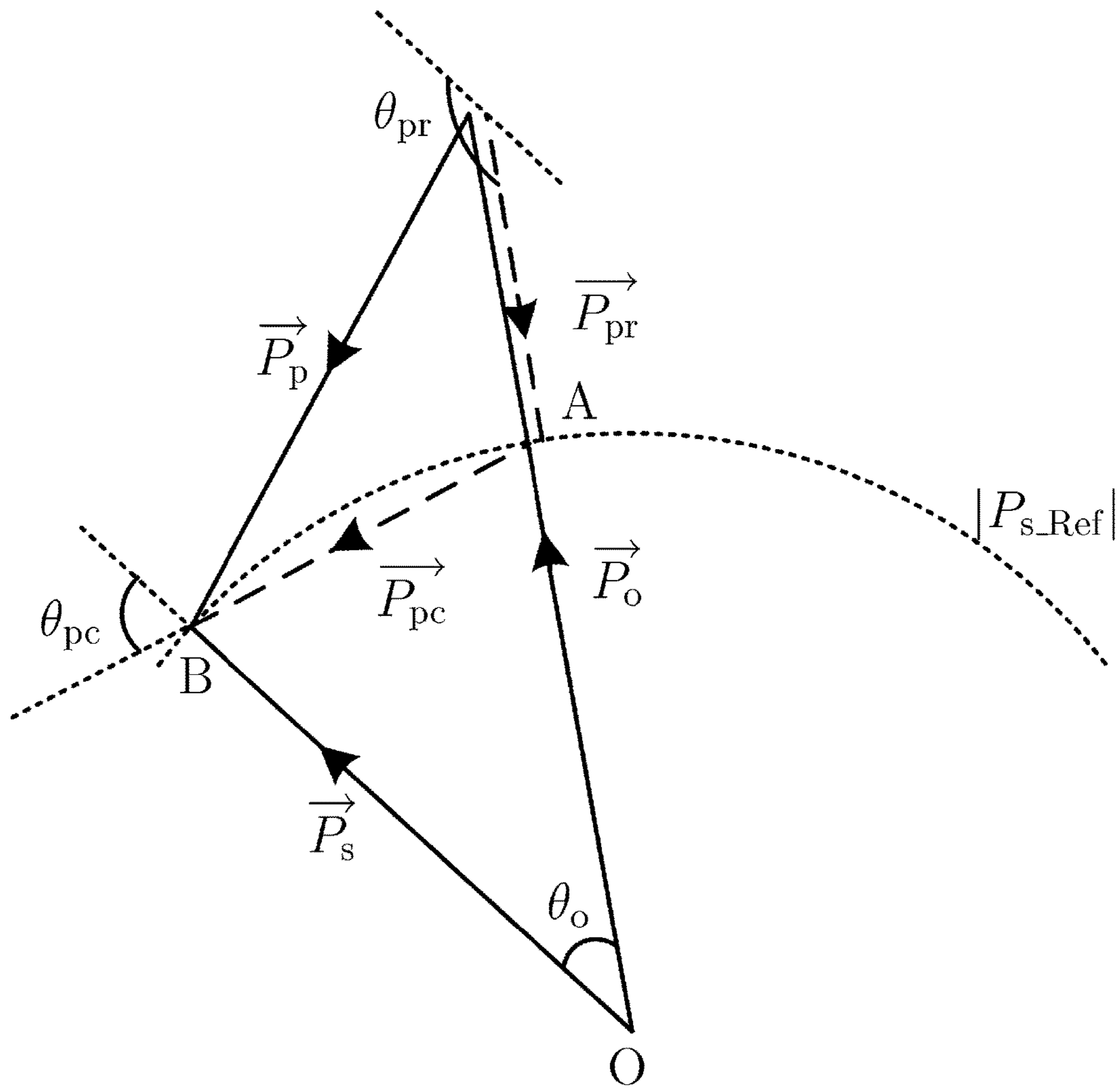
FIG. 21B
