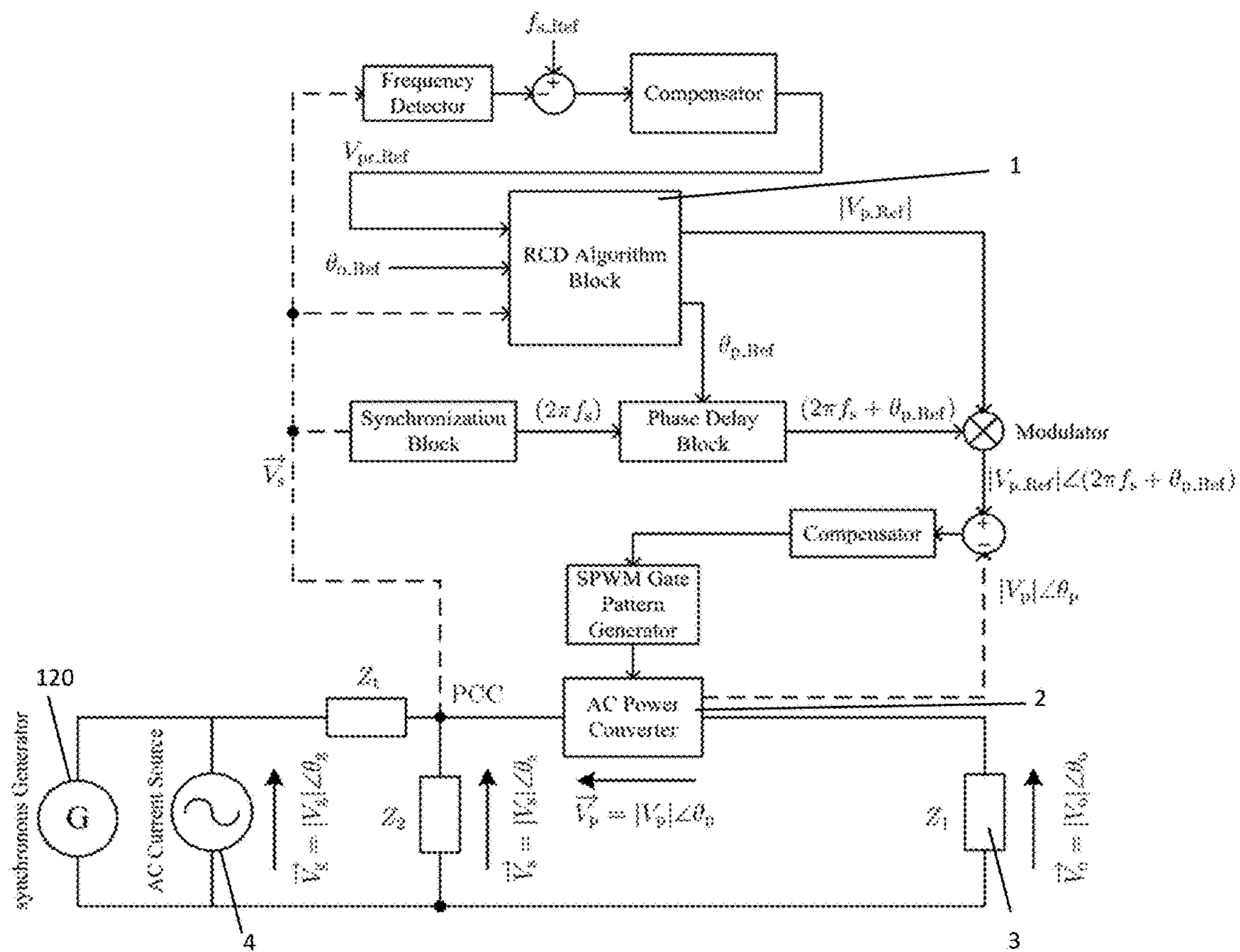
FIG. 18
