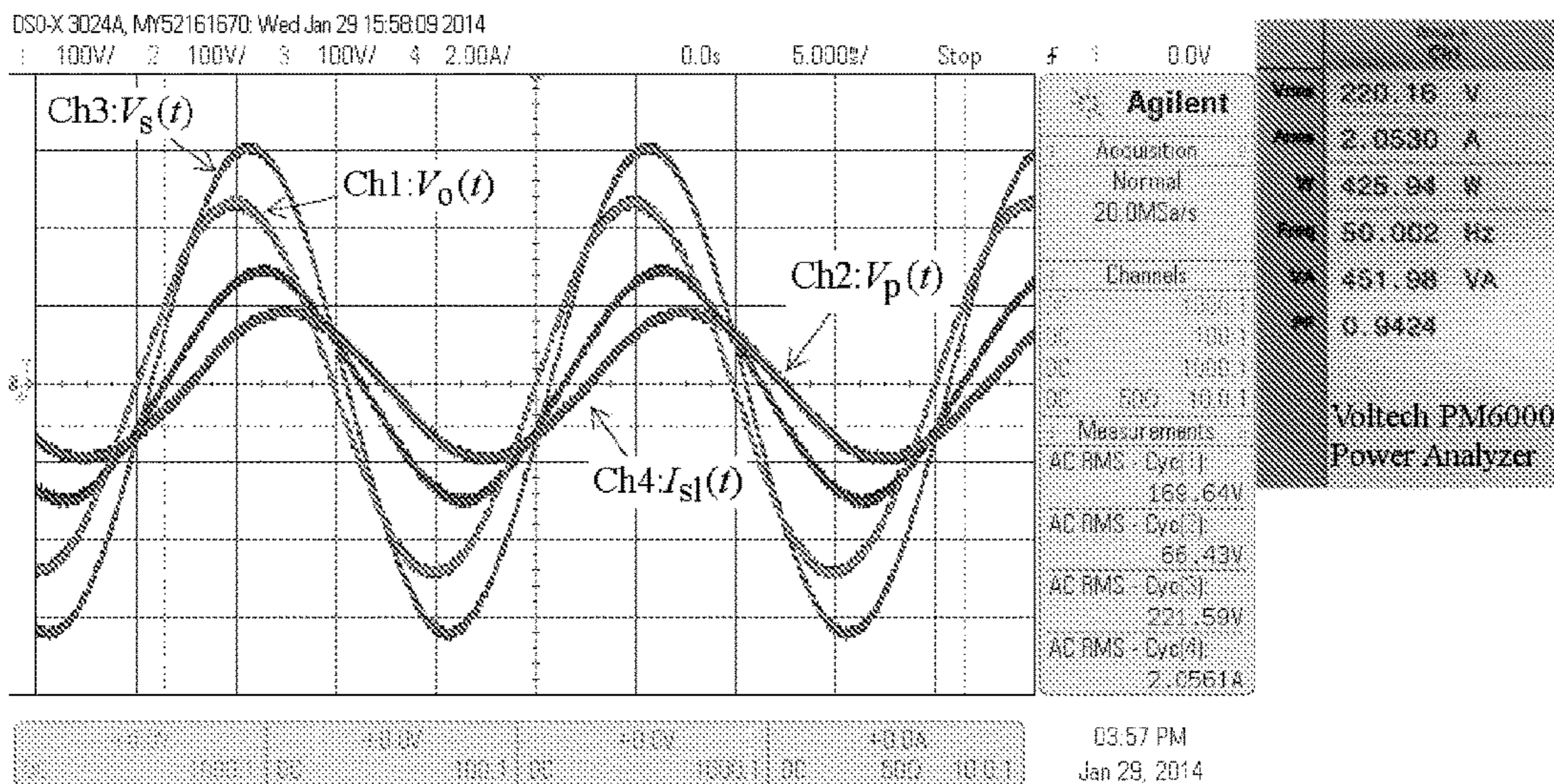
FIG. 13E
