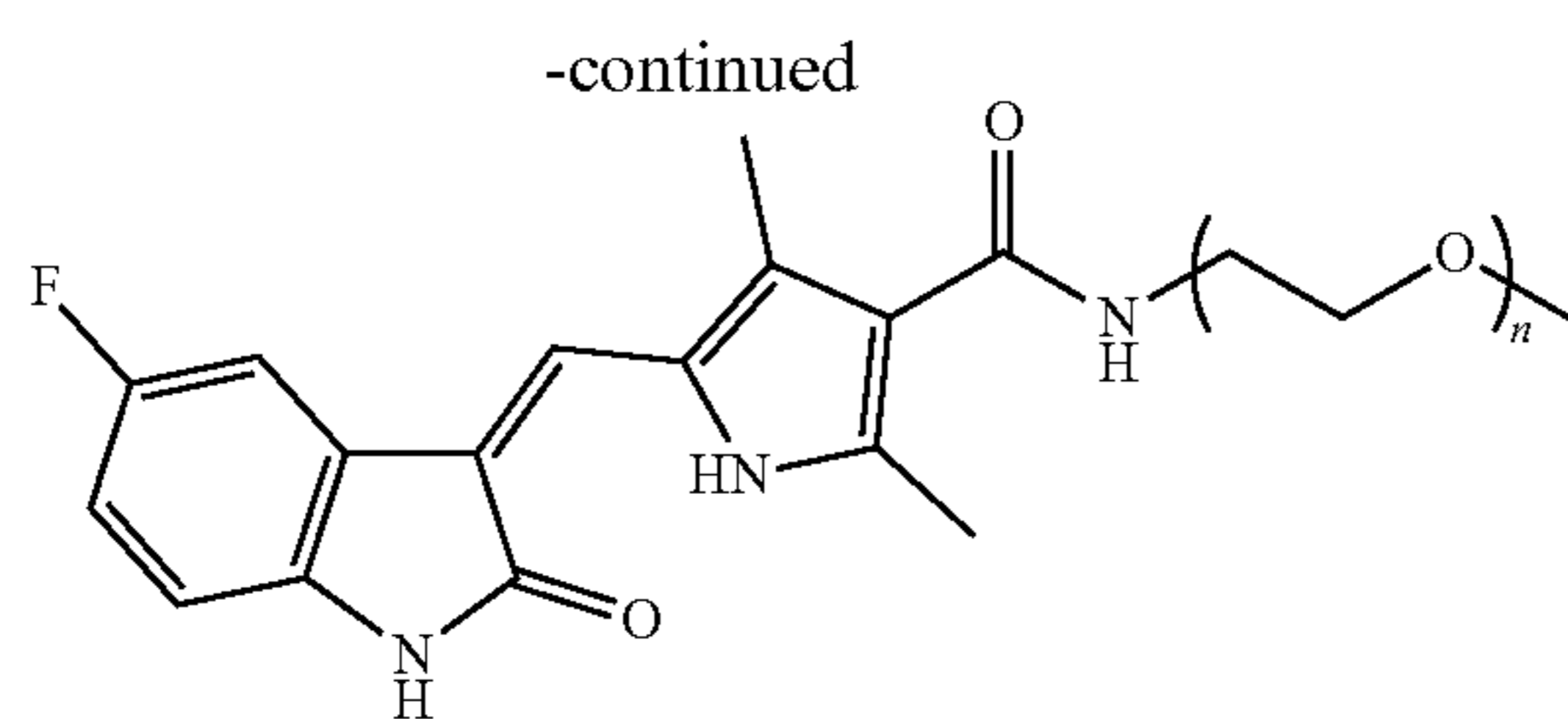
(Z)-5-((5-fluoro-2-oxoindolin-3-ylidene)methyl)- 2,4-dimethyl-1H-pyrrole-3-mPEG n -amide
