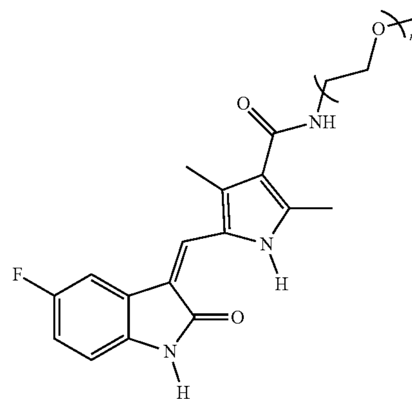
mPEG n -Semamaxanib (n = 3-9)
