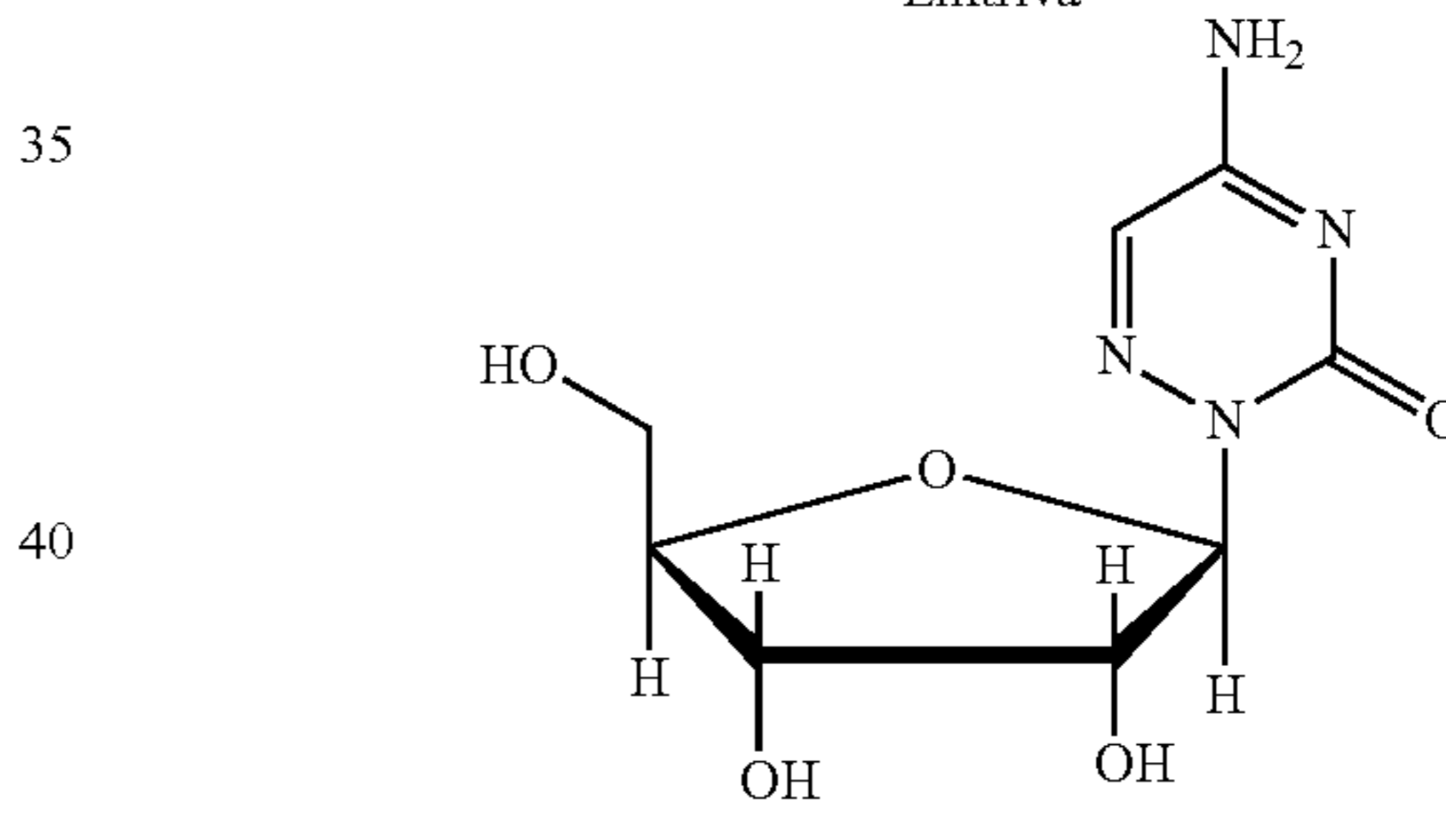
6-Azacytidine
