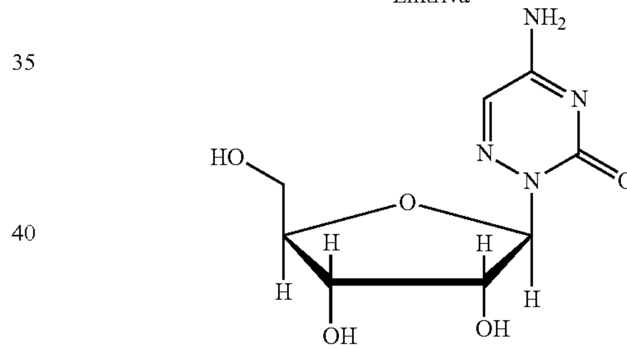
6-Azacytidine
