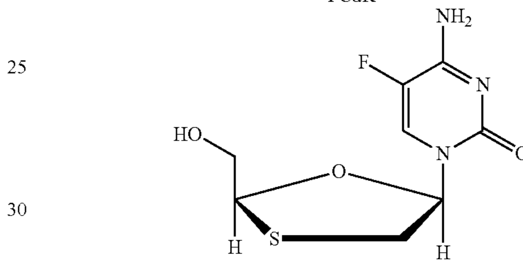
Emtriva
