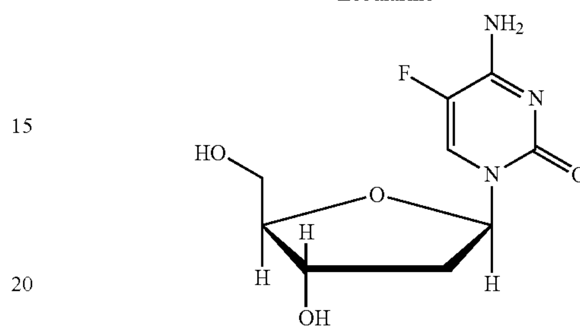
FCdR
