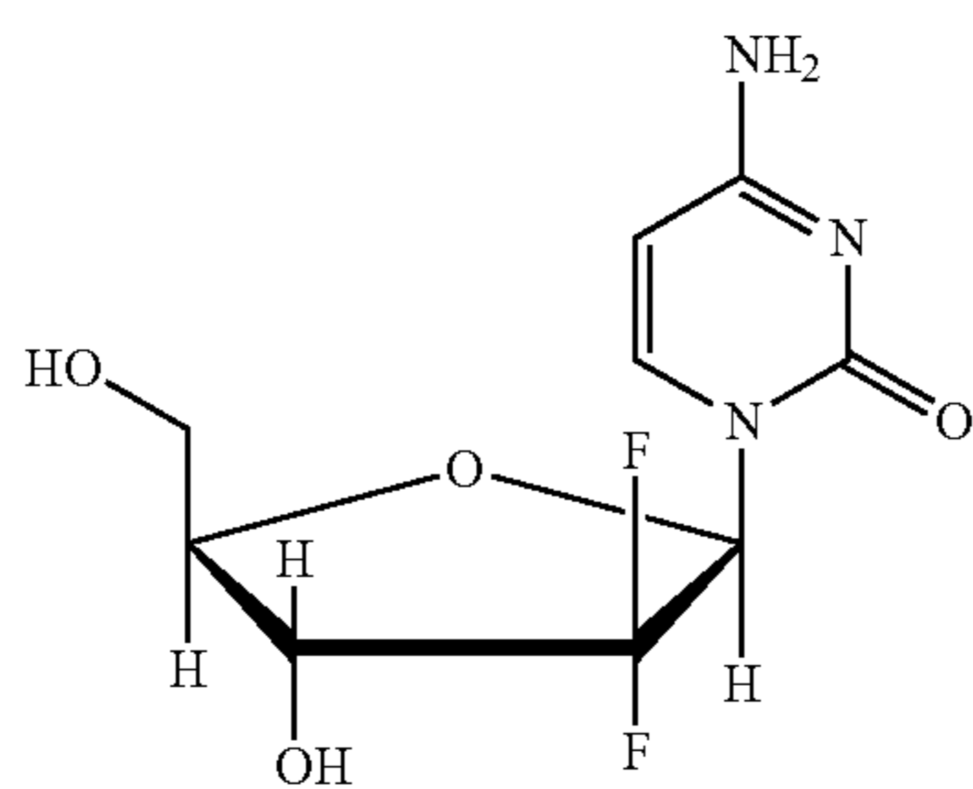
Gemcitabine
