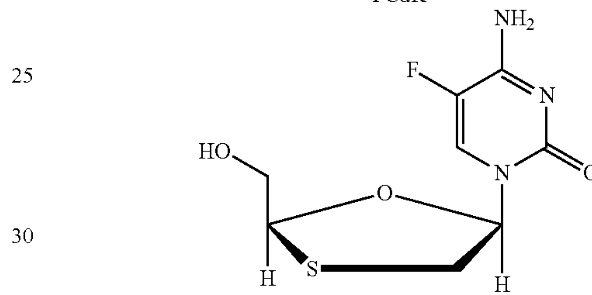
Emtriva
