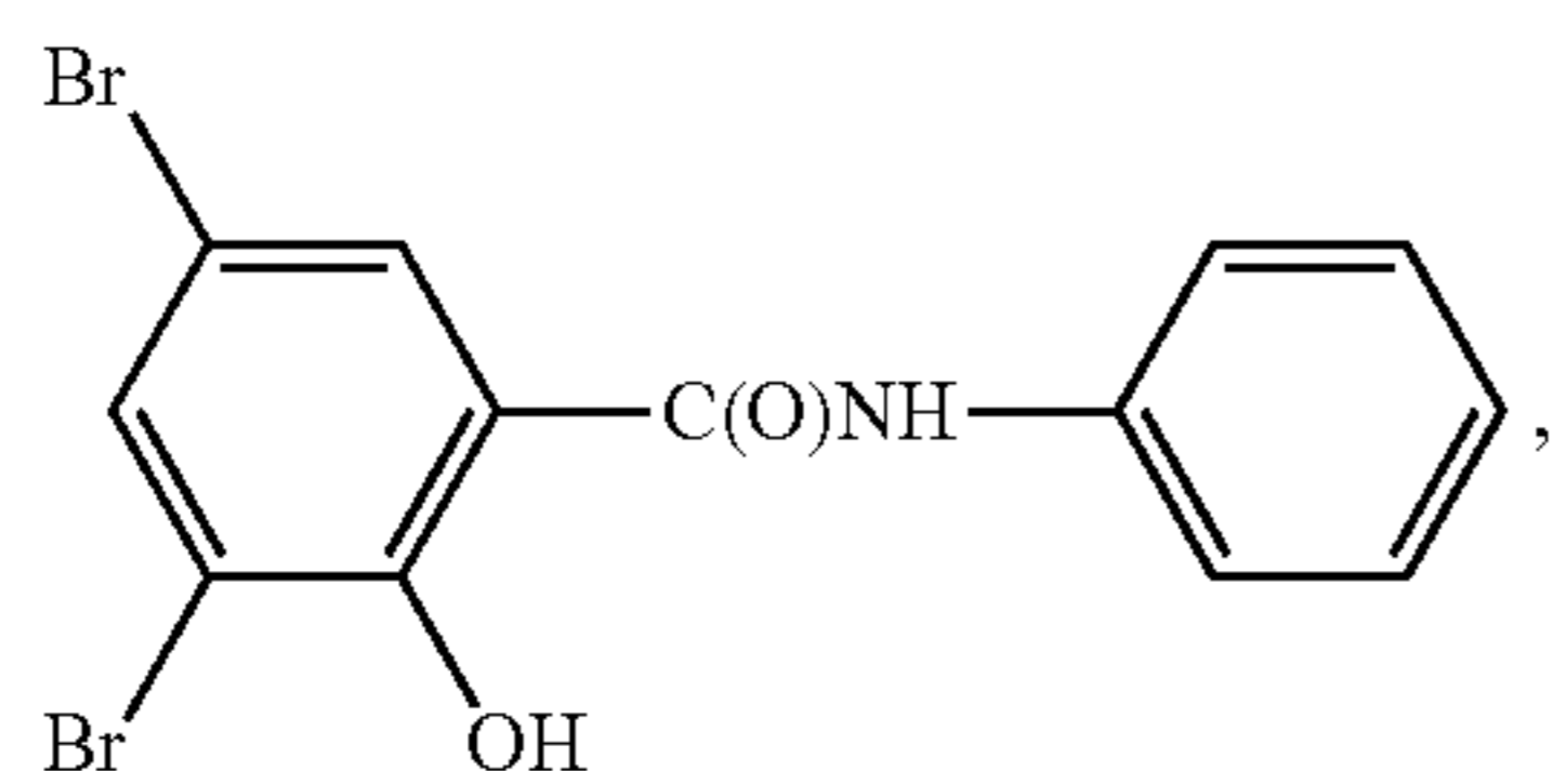
dibromosalalan
