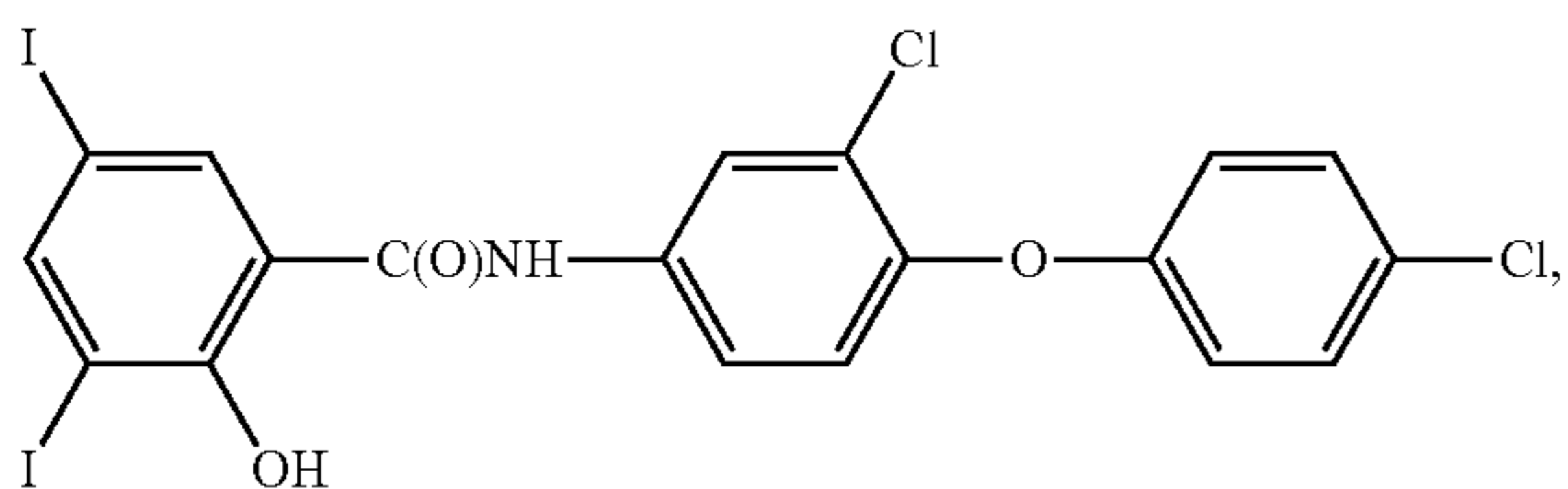
rafoxanide
