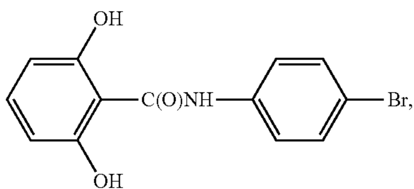
resorantel
