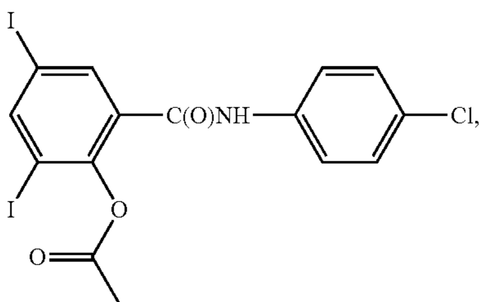
clioxanide
