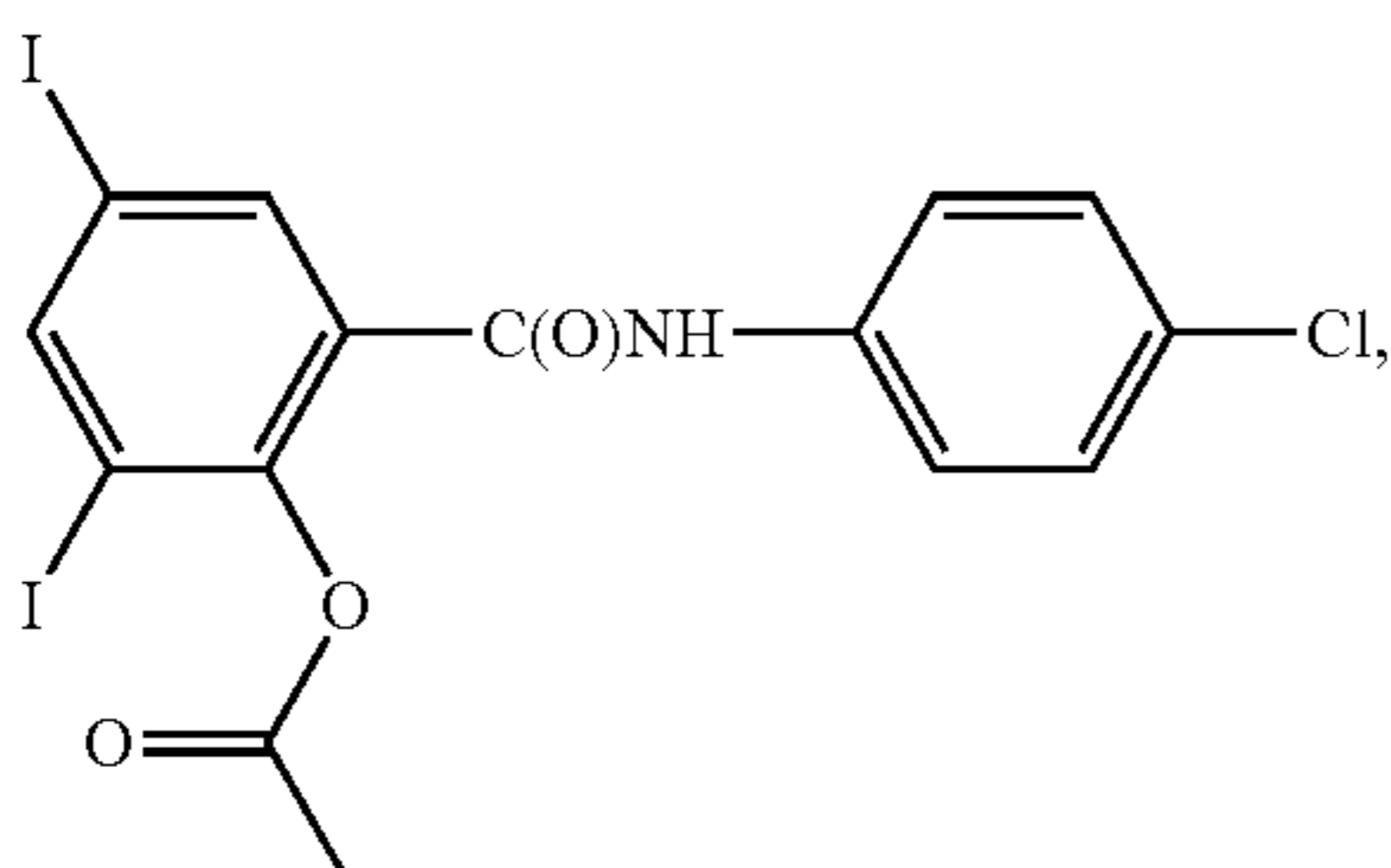
clioxanide
