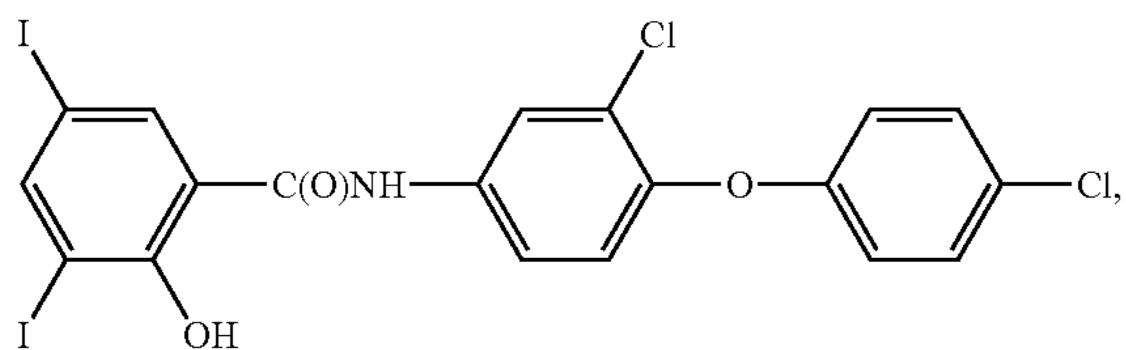
rafoxanide
