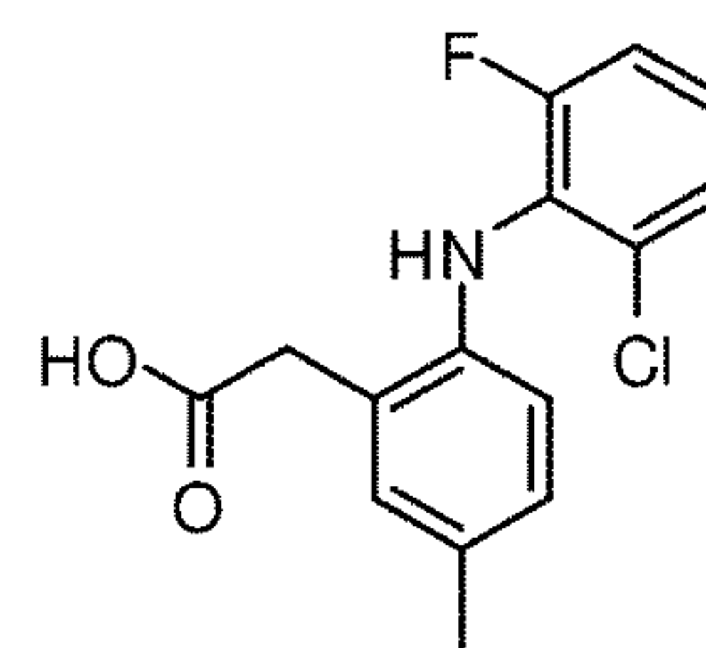
Lumiracoxib
