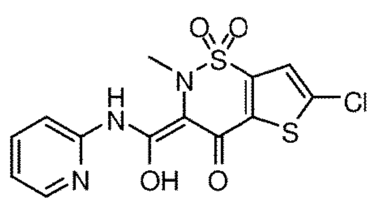
Lornoxicam
