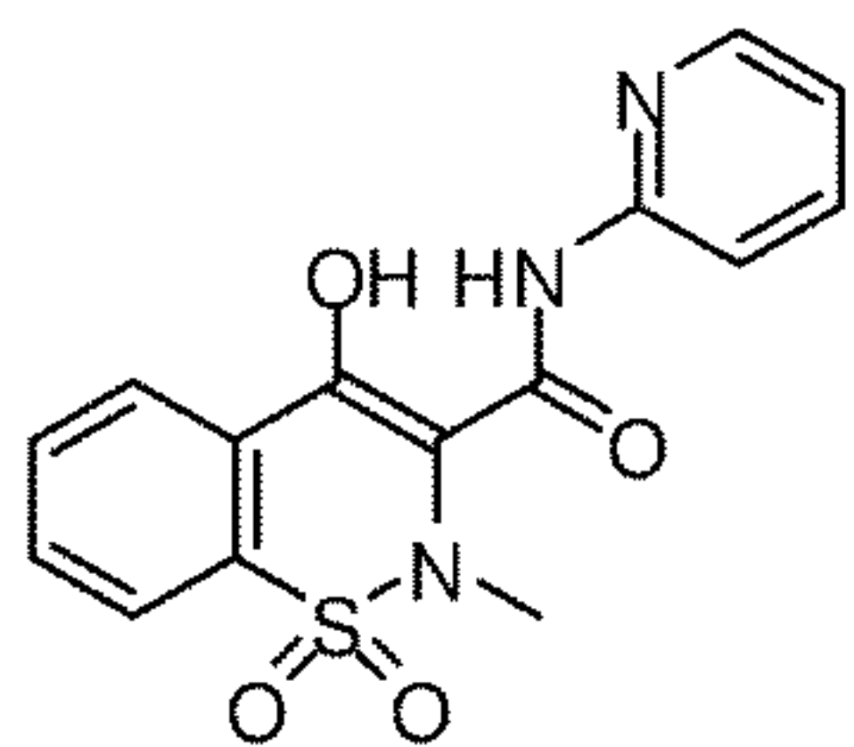
Piroxicam
