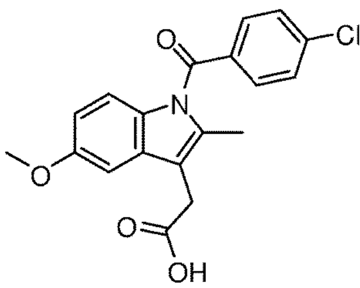
Indomethacin
