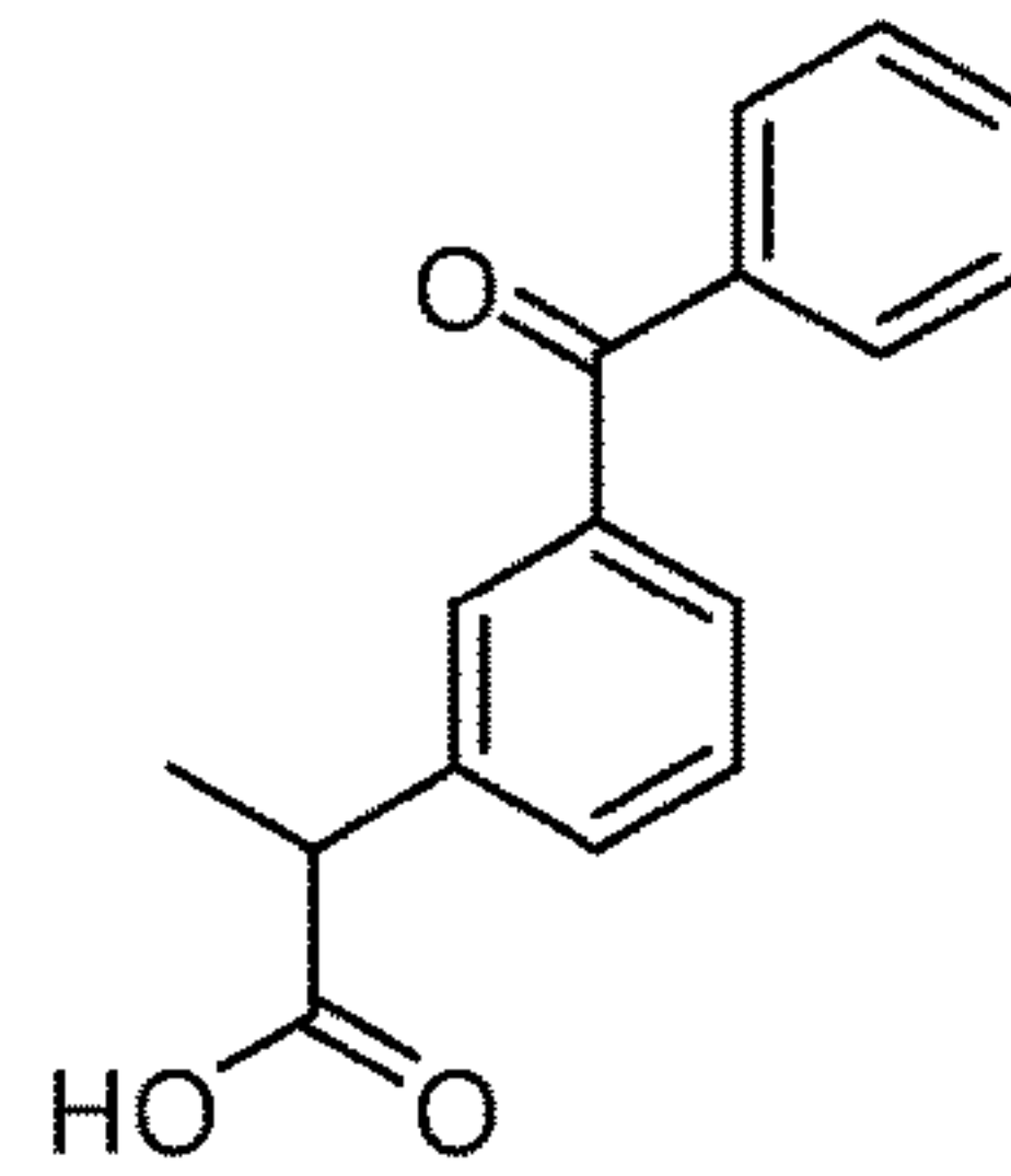
Ketoprofen
