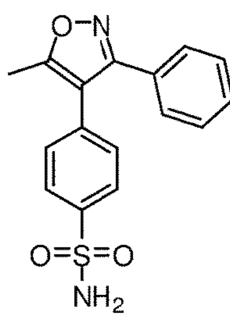
Valdecoxib
