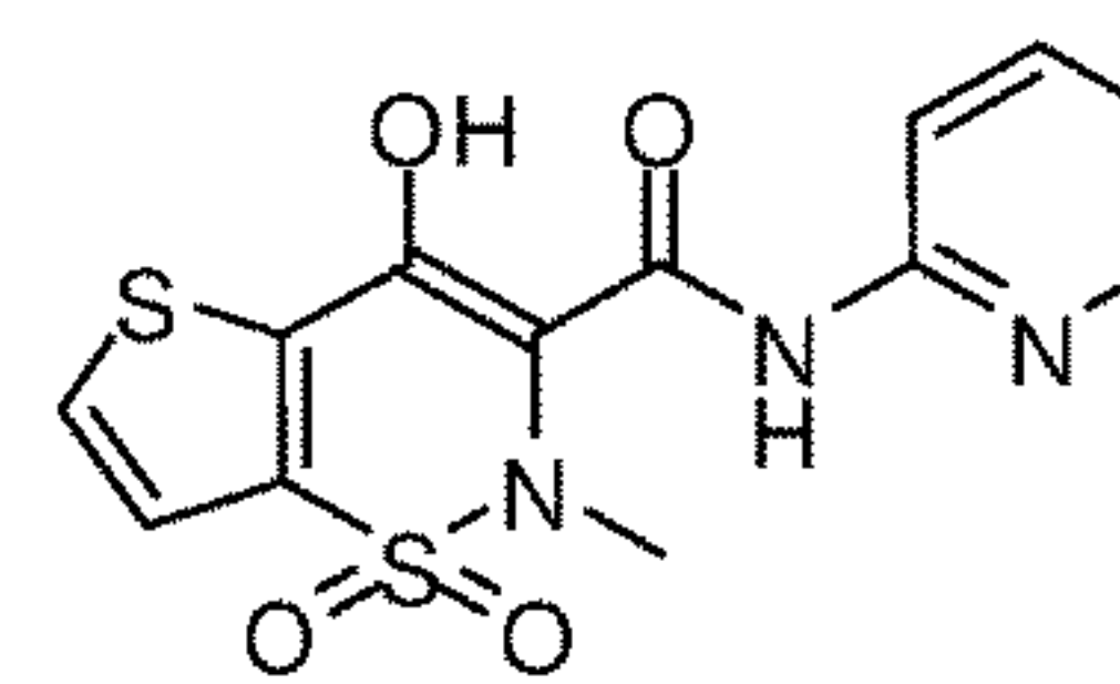
Tenoxicam
