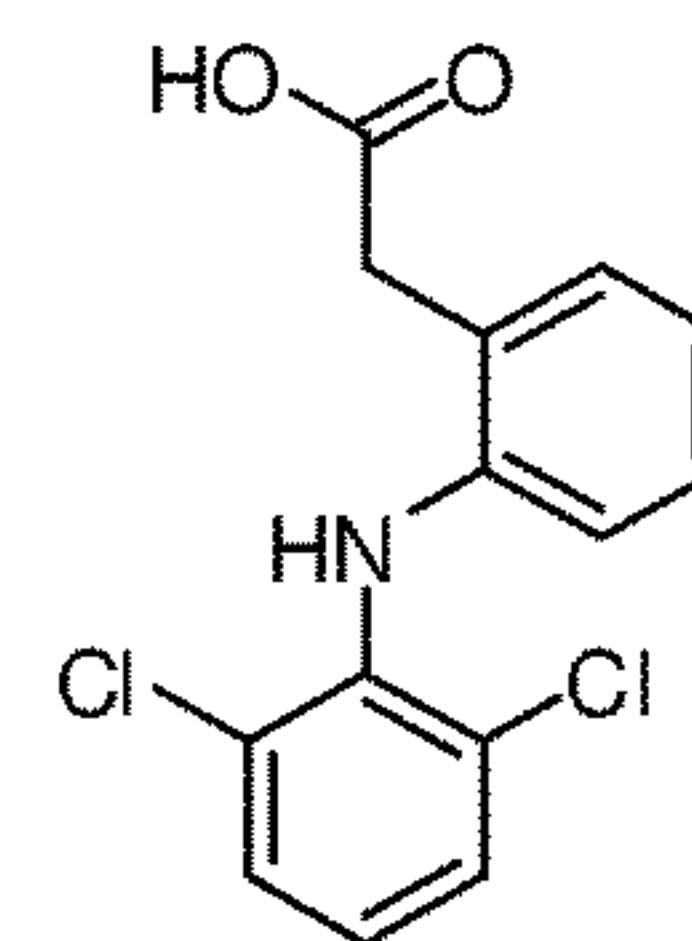
Diclofenac
