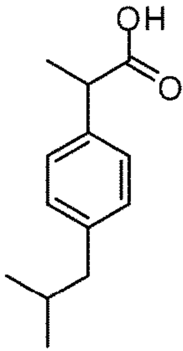
Ibuprofen
