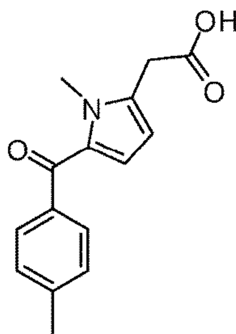
Tolmetin
