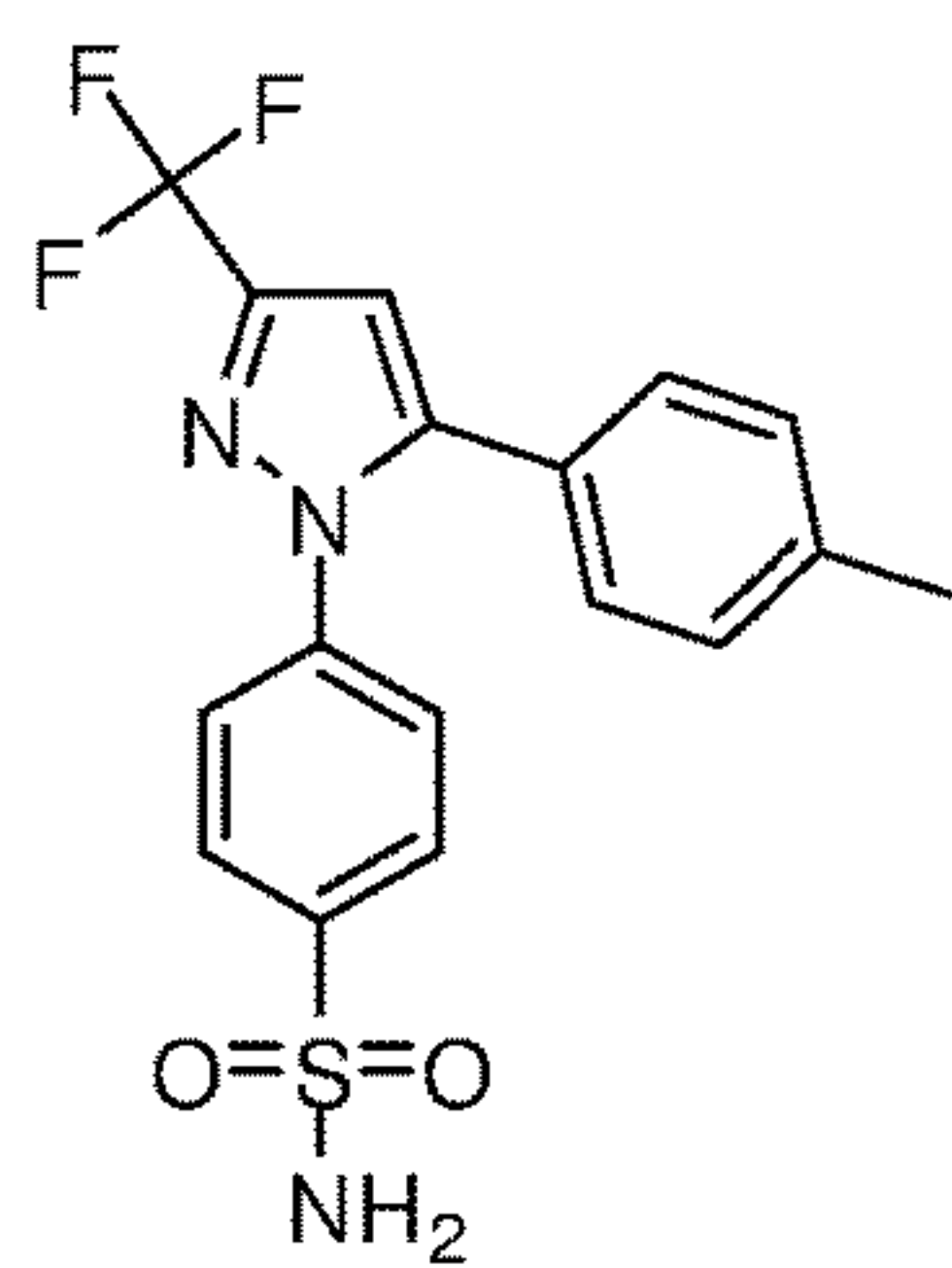
Celecoxib
