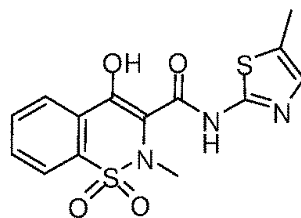
Meloxicam
