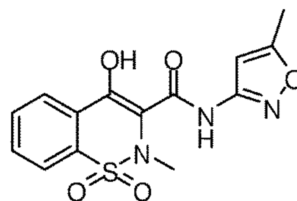
Isoxicam
