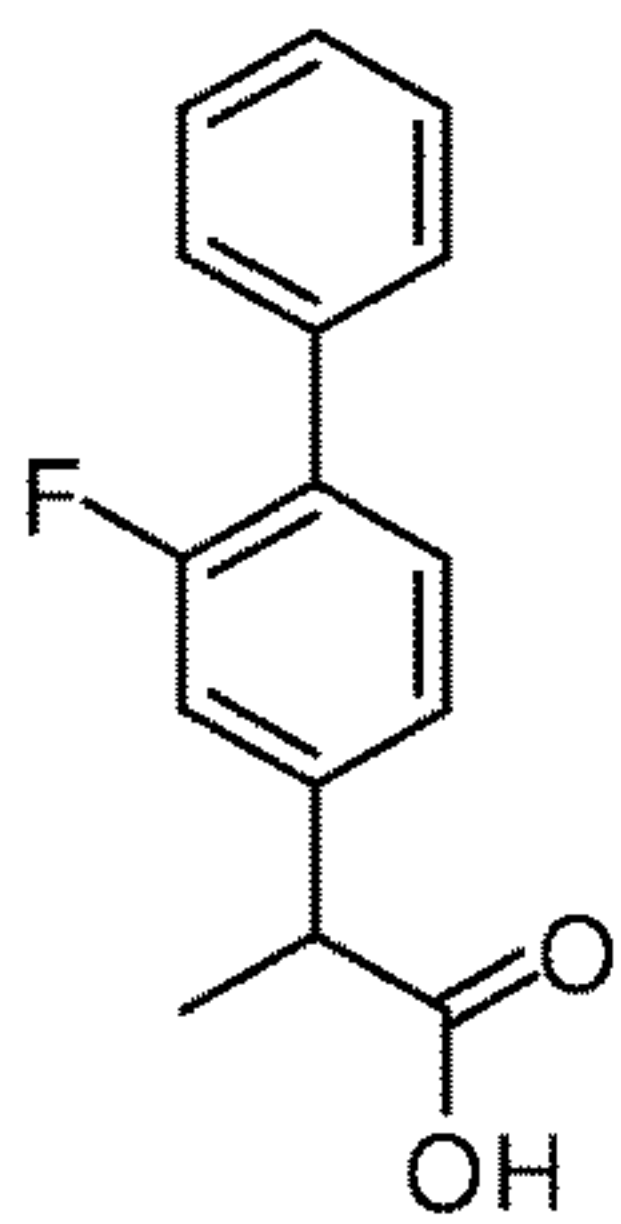
Flurbiprofen
