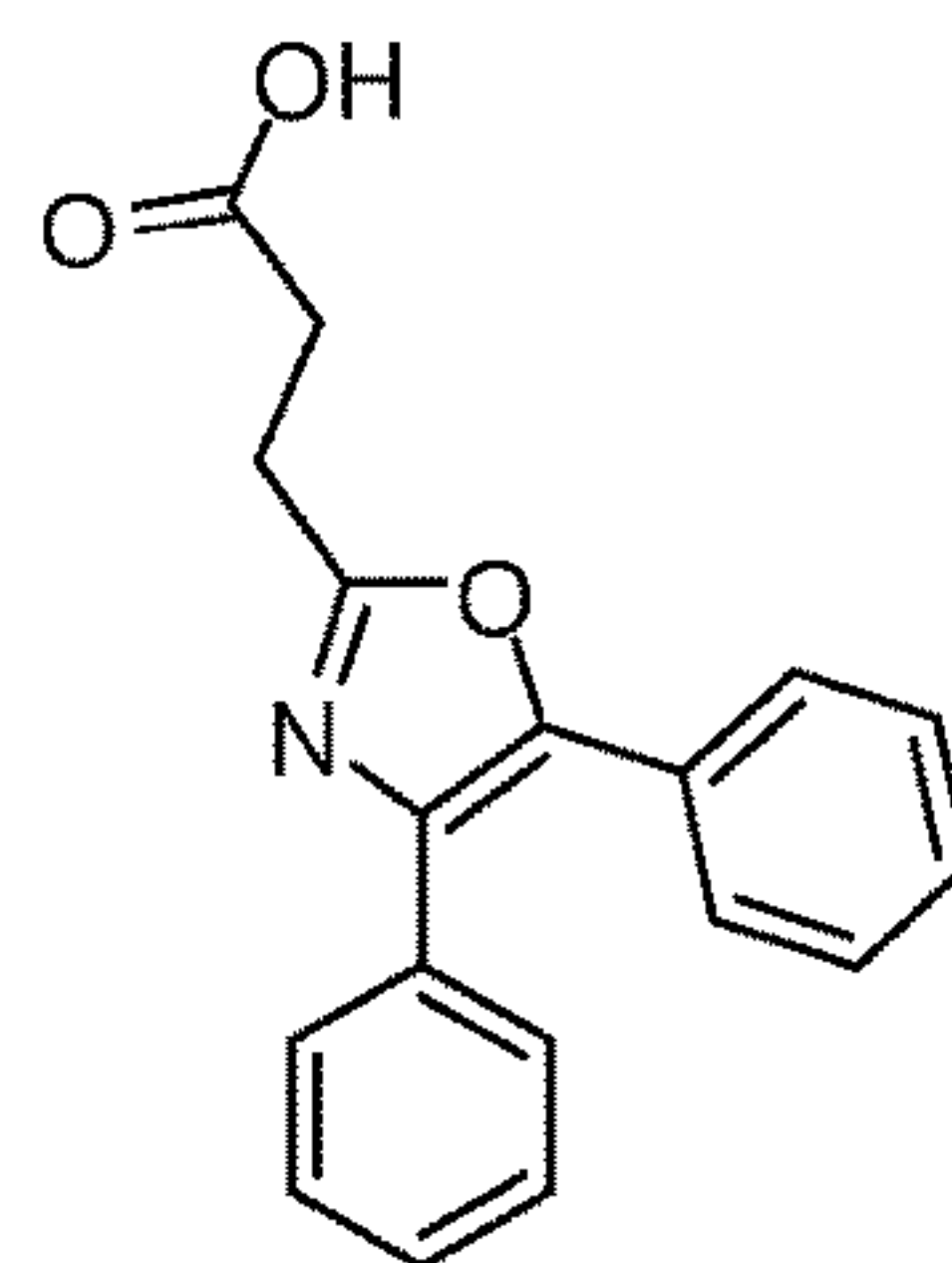
Oxaprozin
