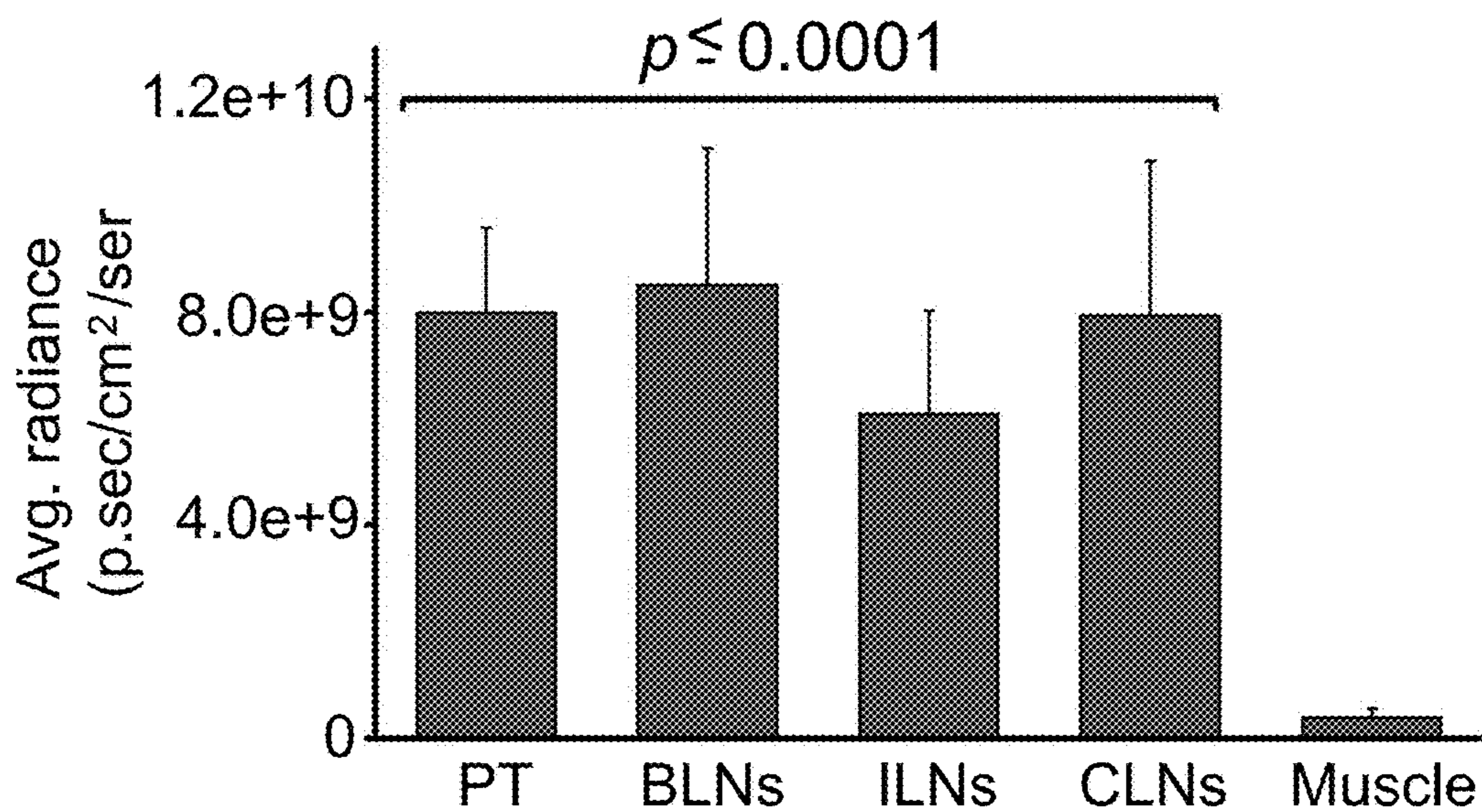
FIG. 10 MN-scr-miR
