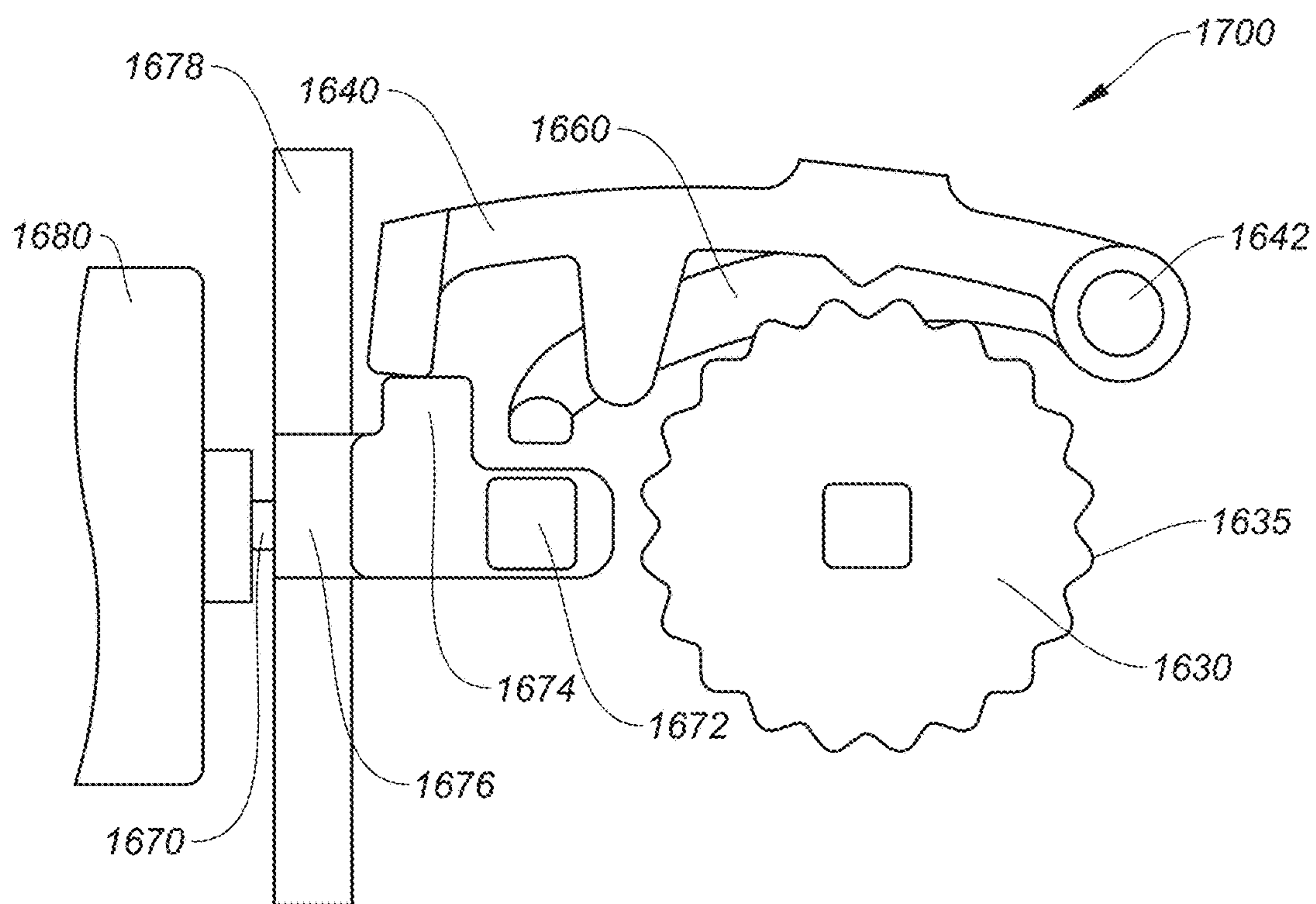
FIG. 17B
