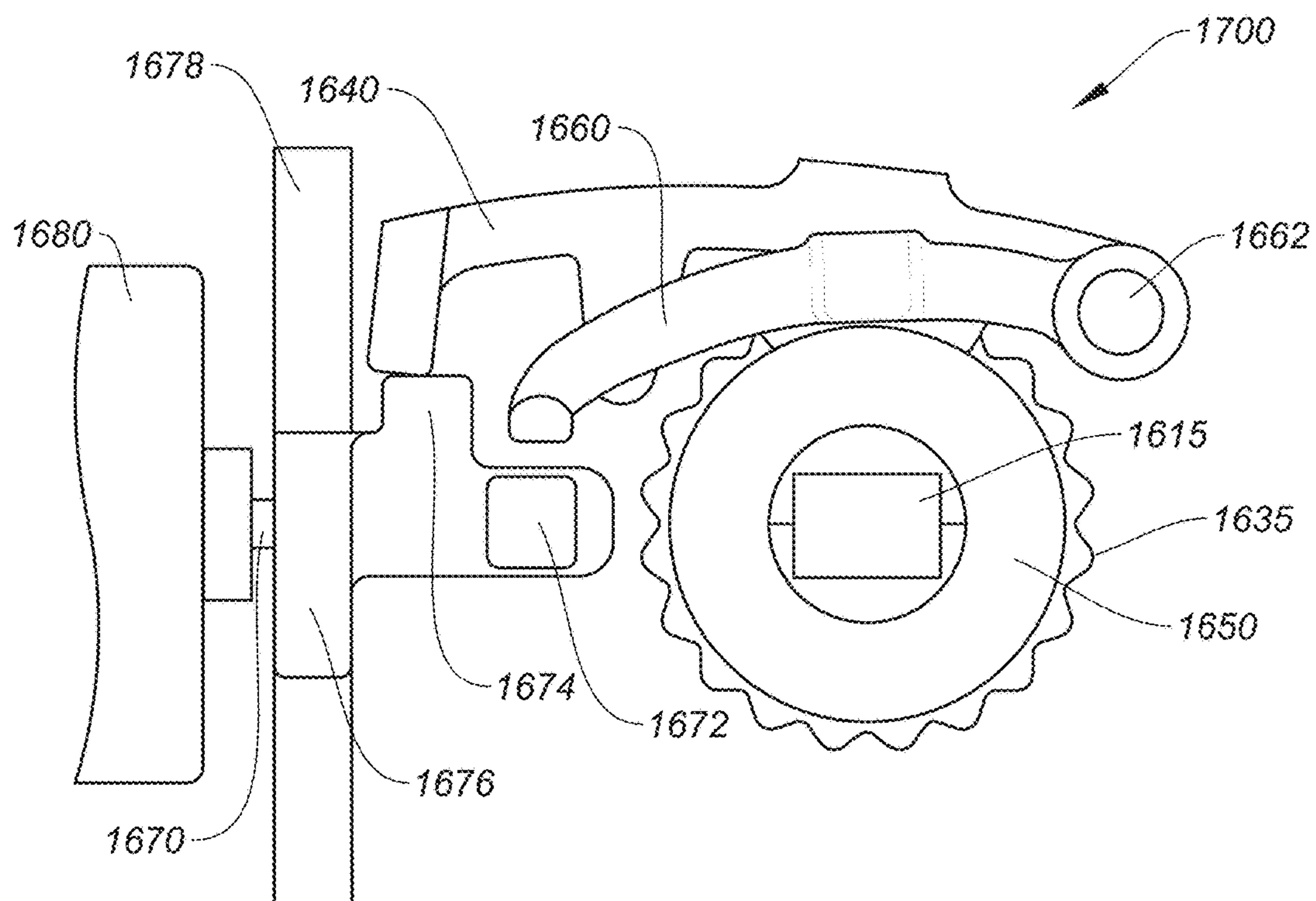
FIG. 17A
