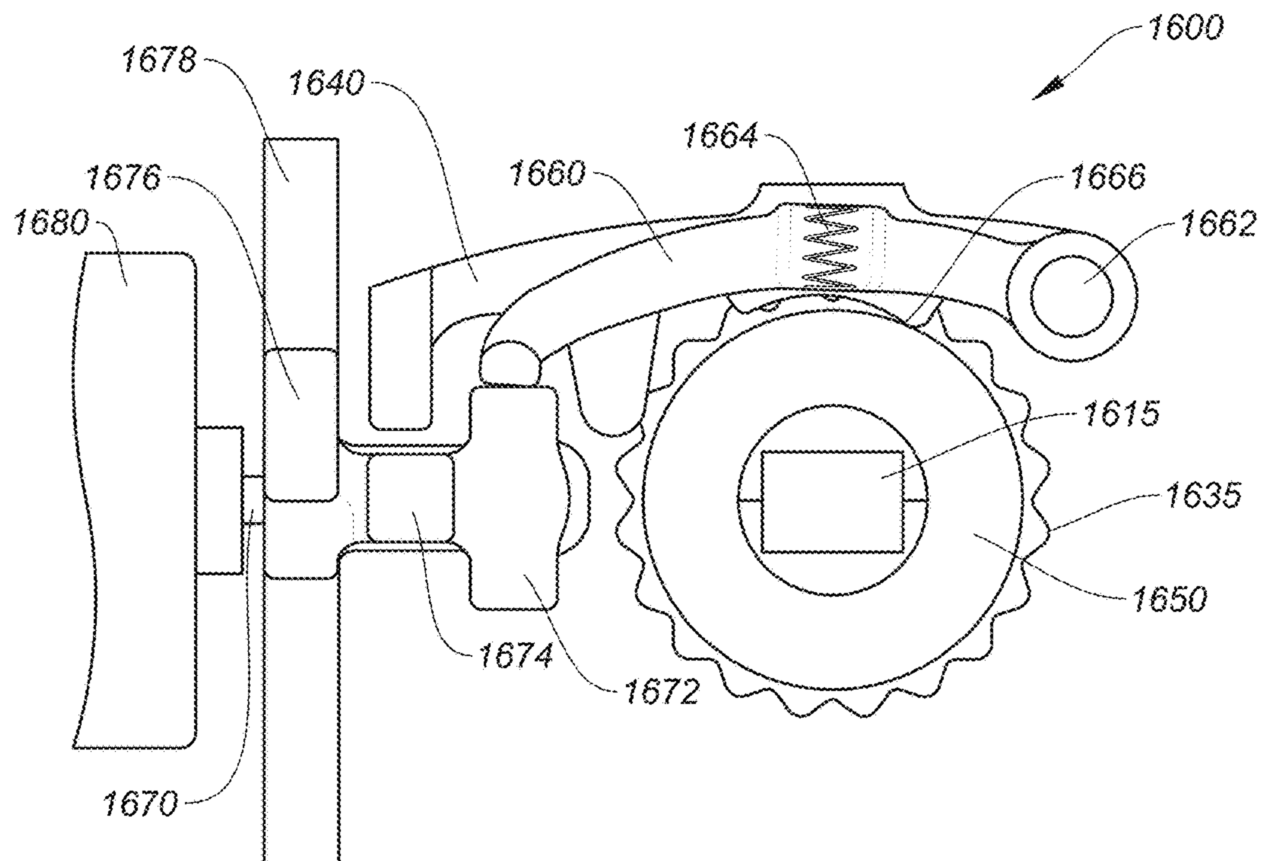
FIG. 16A
