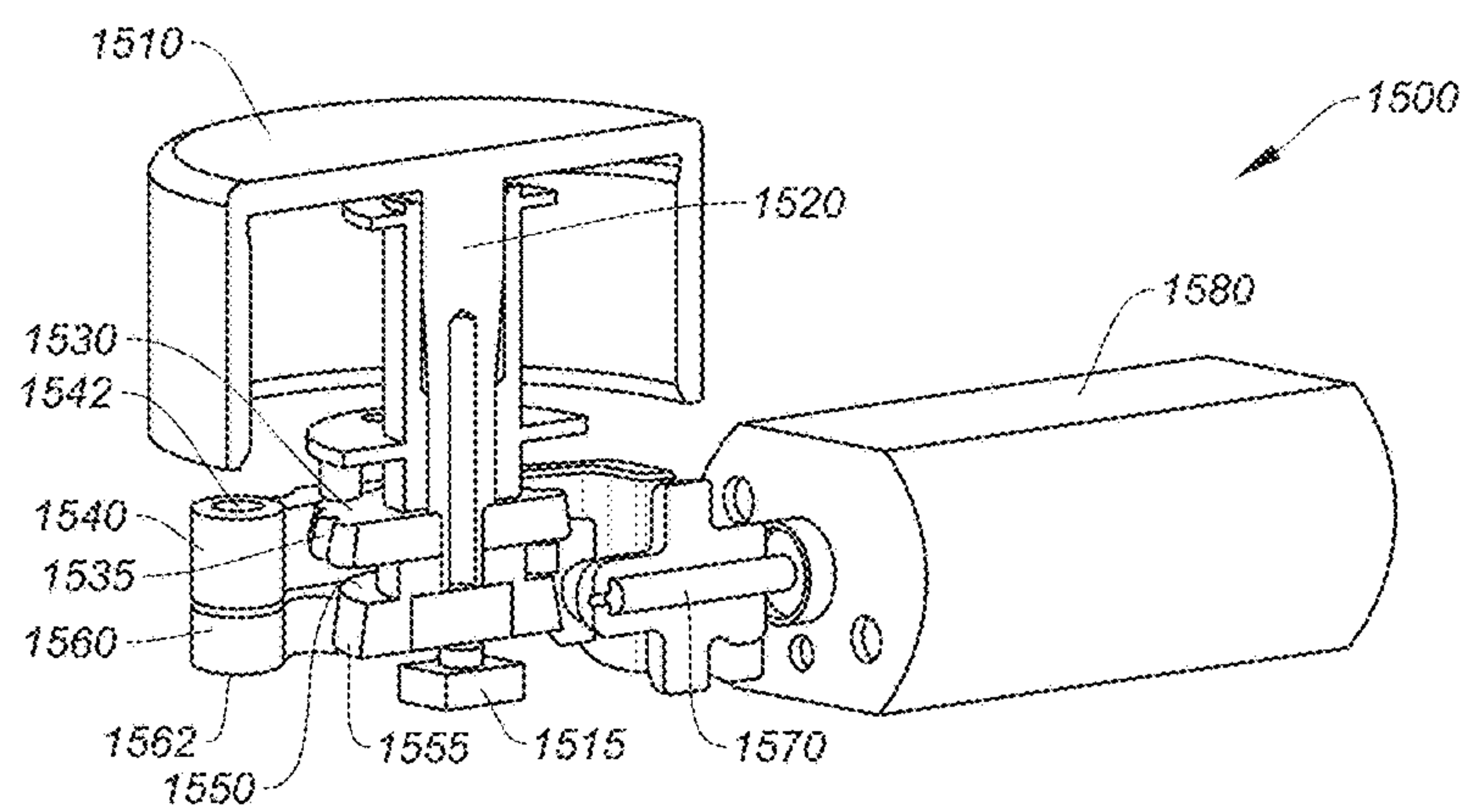
FIG. 15A
