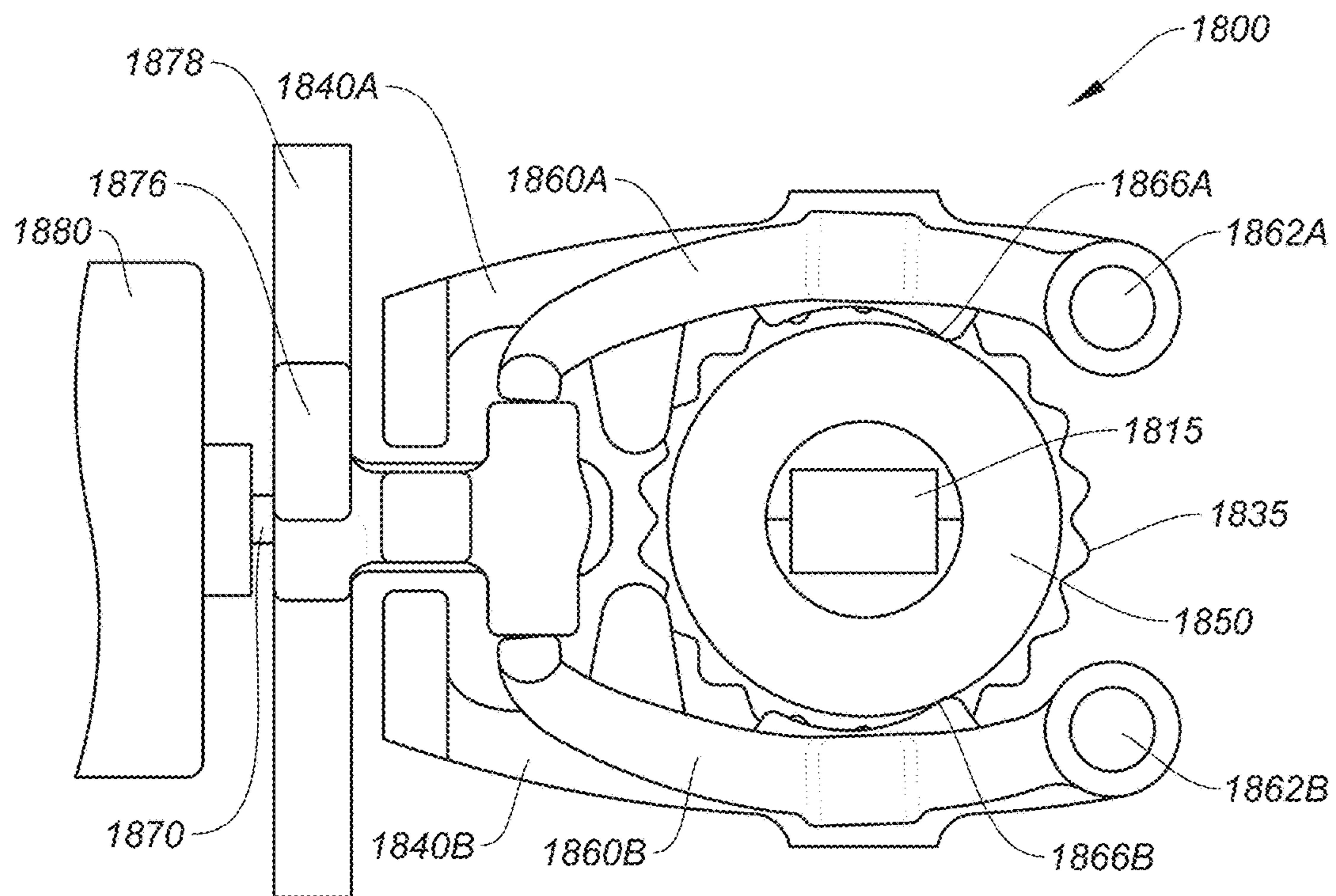
FIG. 18A
