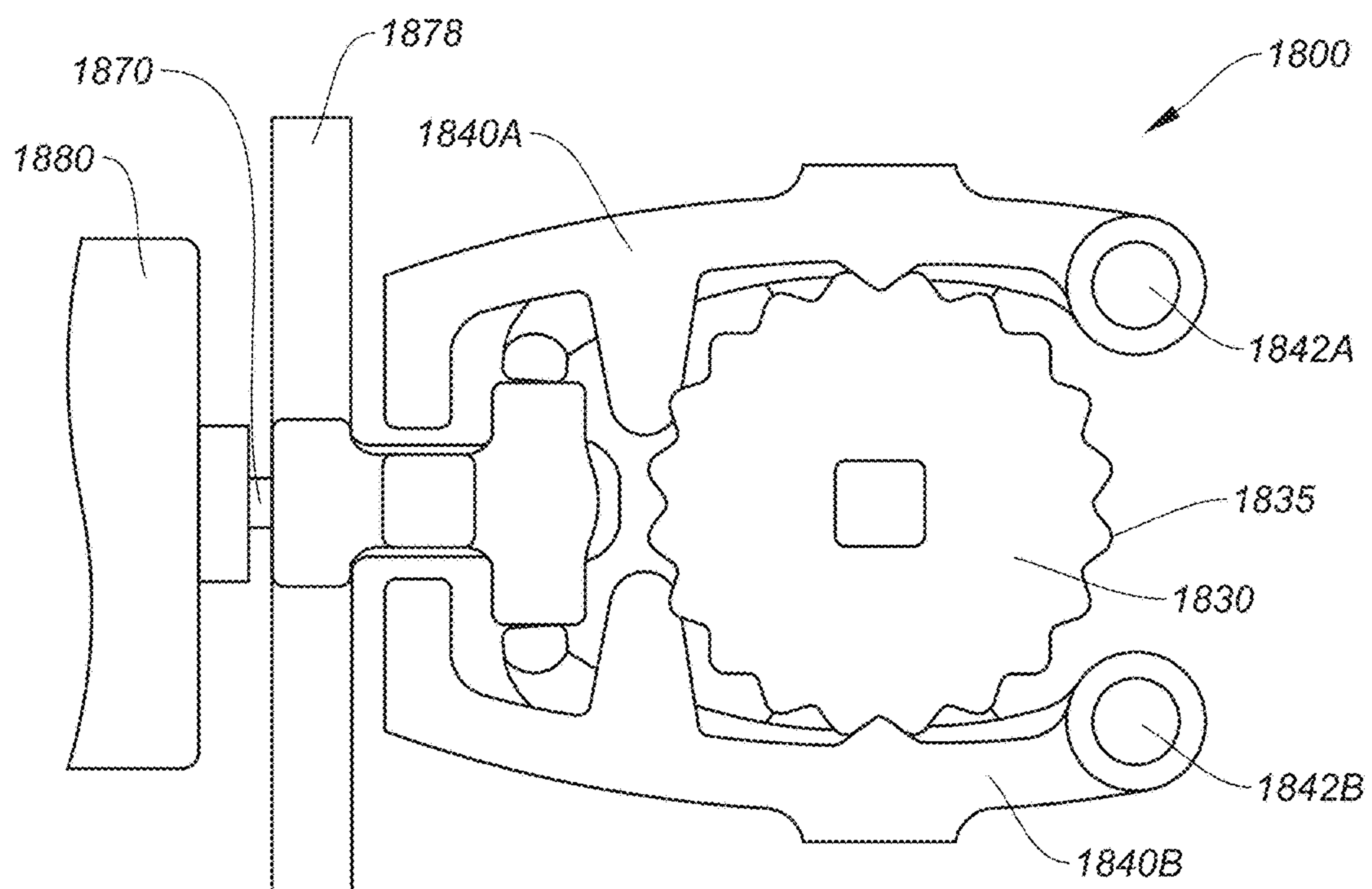
FIG. 18B
