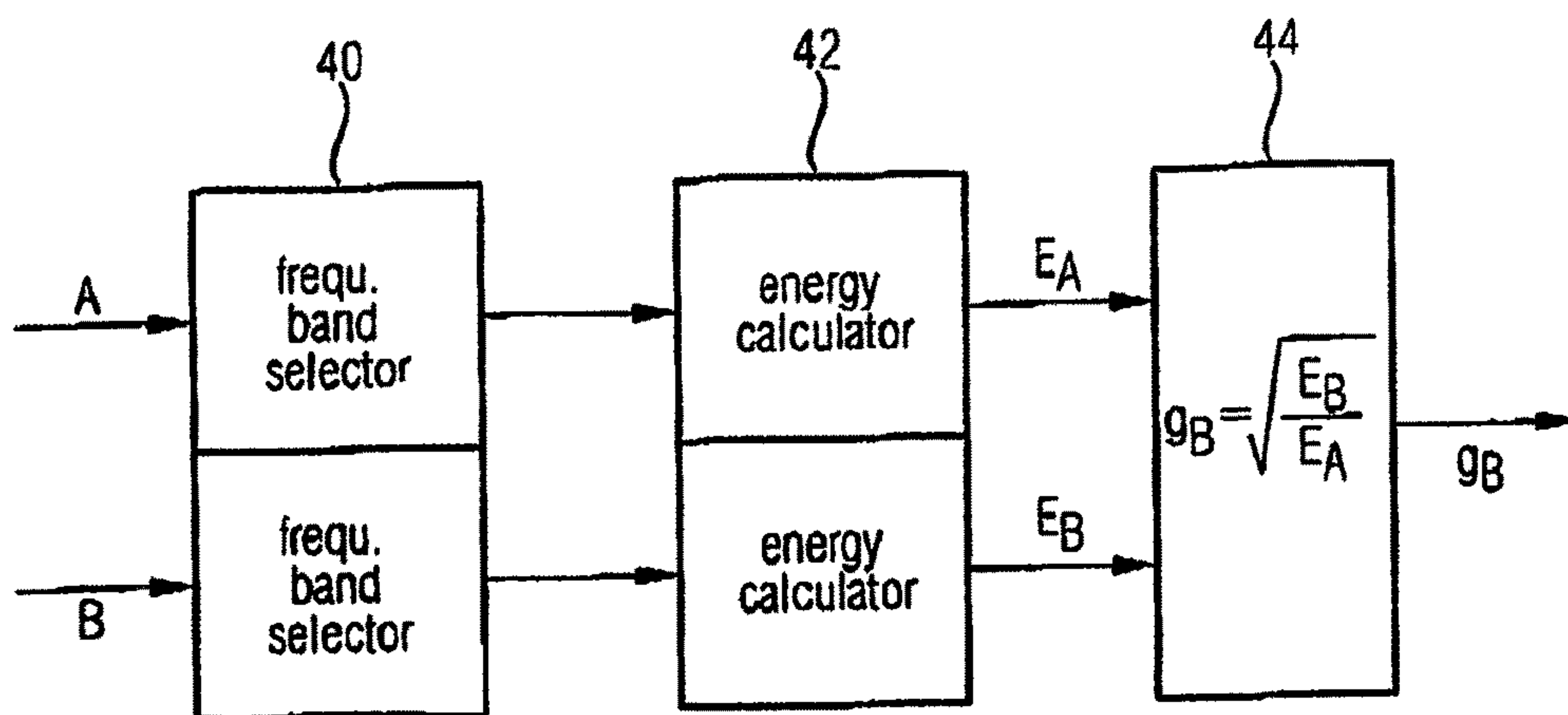
FIG 4 (encoder side)
