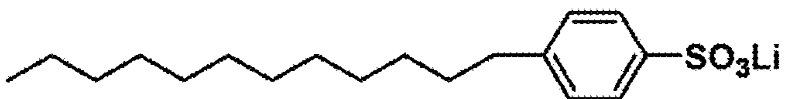
lithium 4-dodecylbenzenesulfonate
