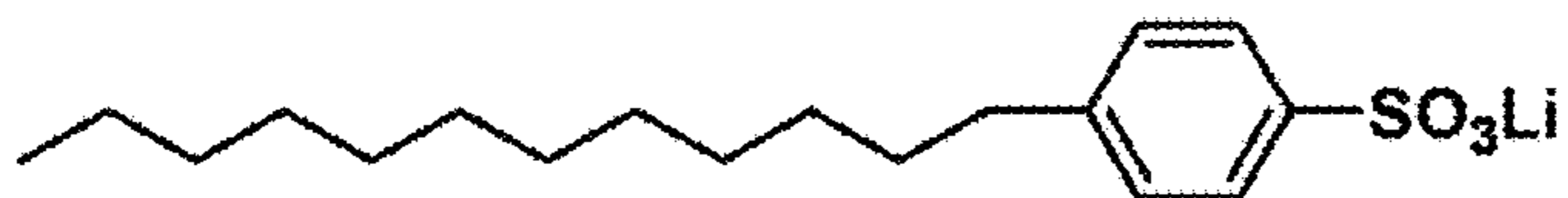
lithium 4-dodecylbenzenesulfonate
