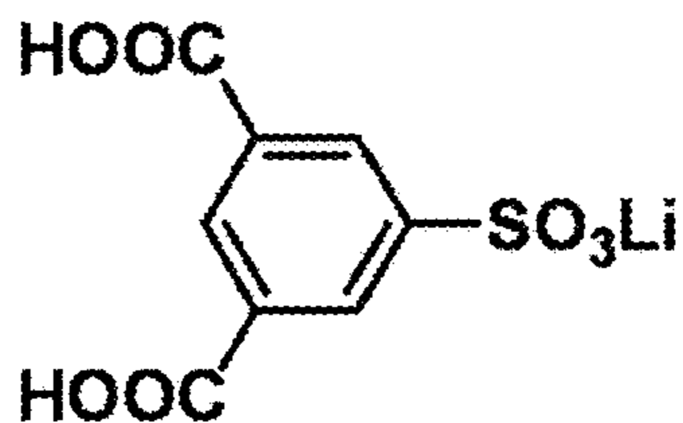
lithium 3,5-dicarboxybenzenesulfonate
