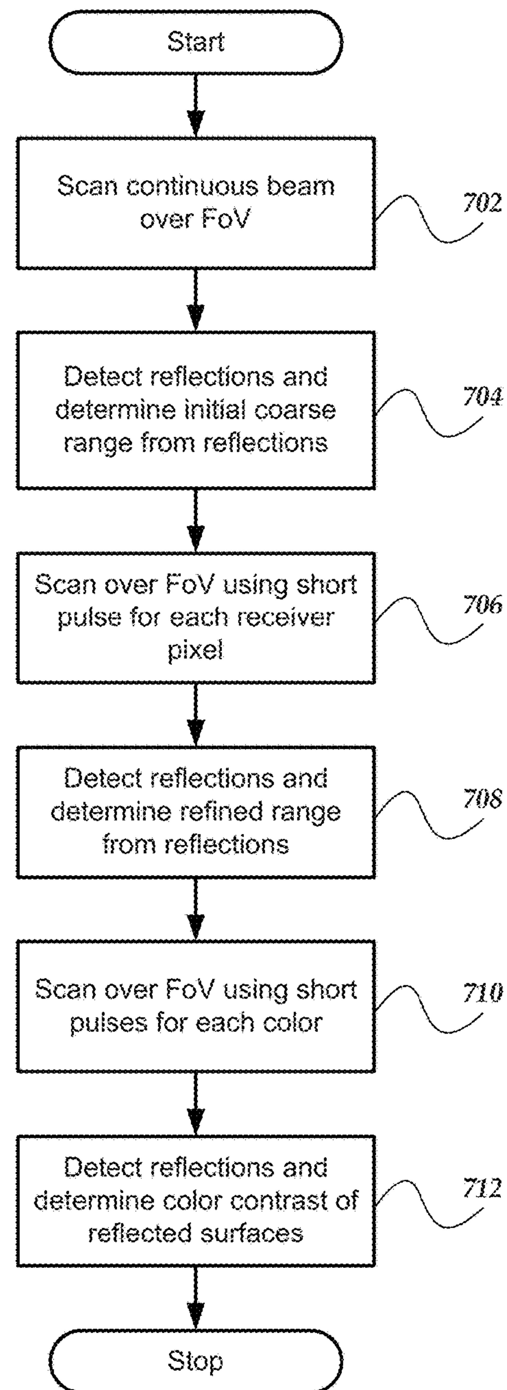
FIG. 7
