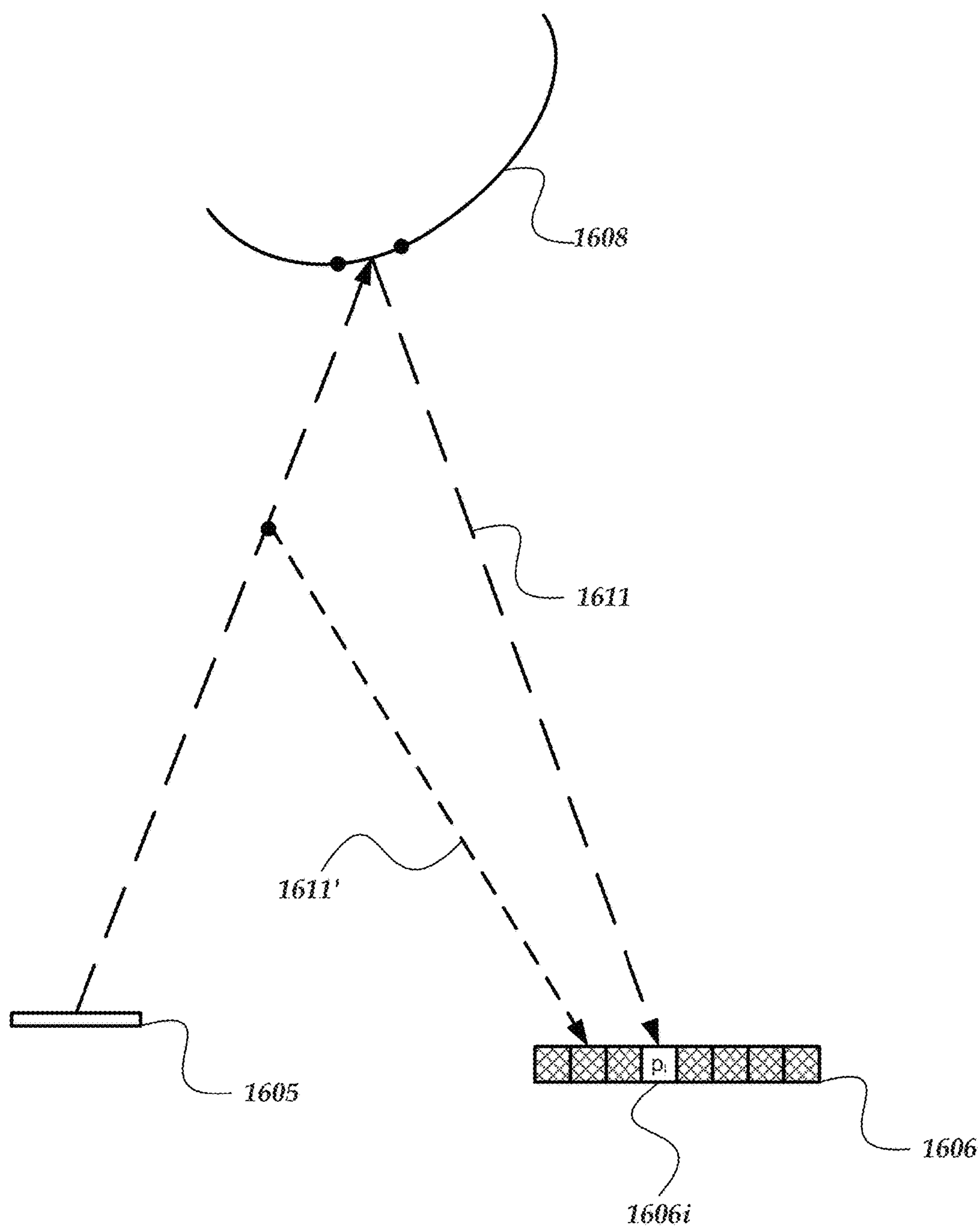
FIG. 16B
