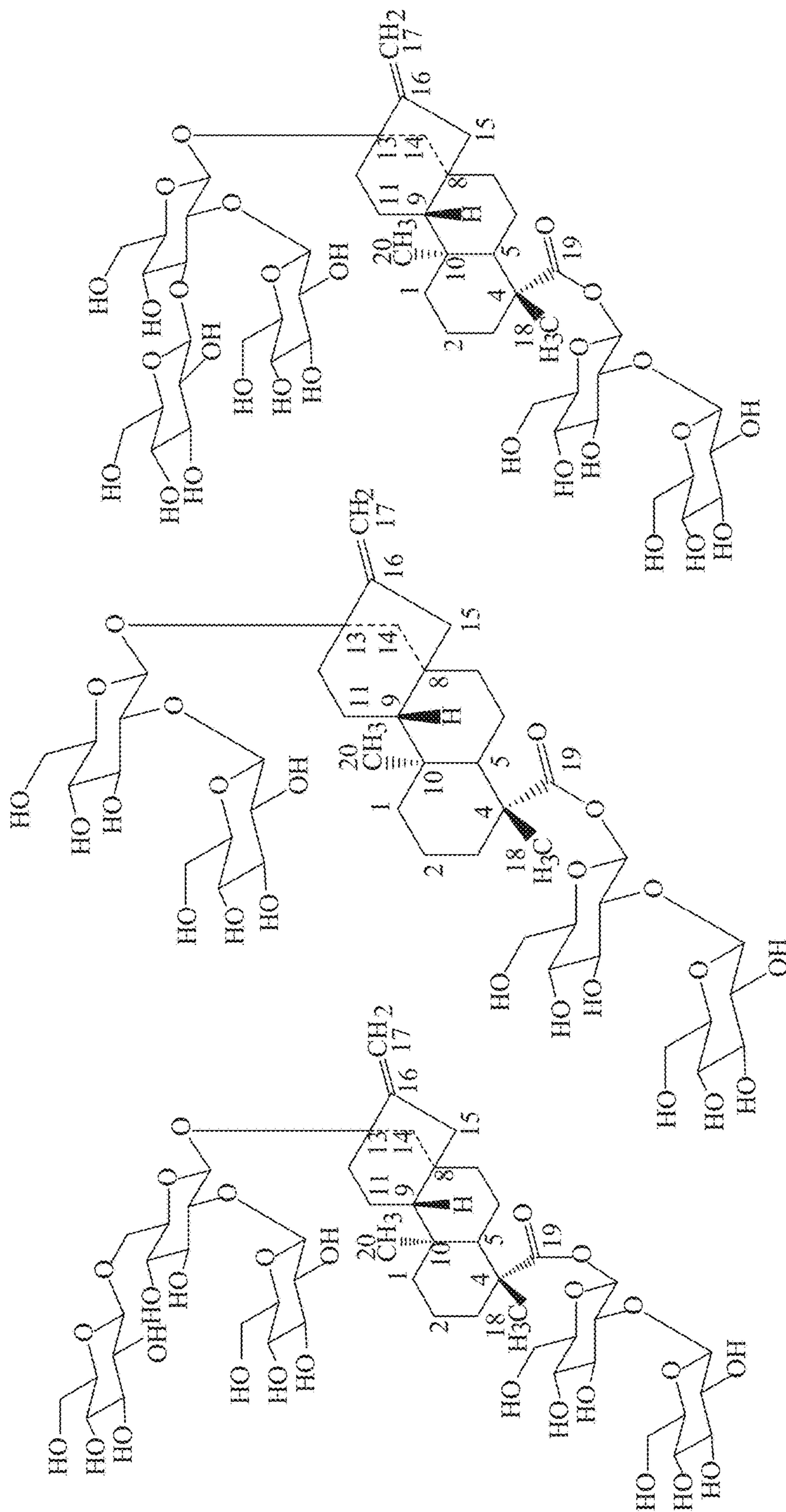
Rebaudioside D
