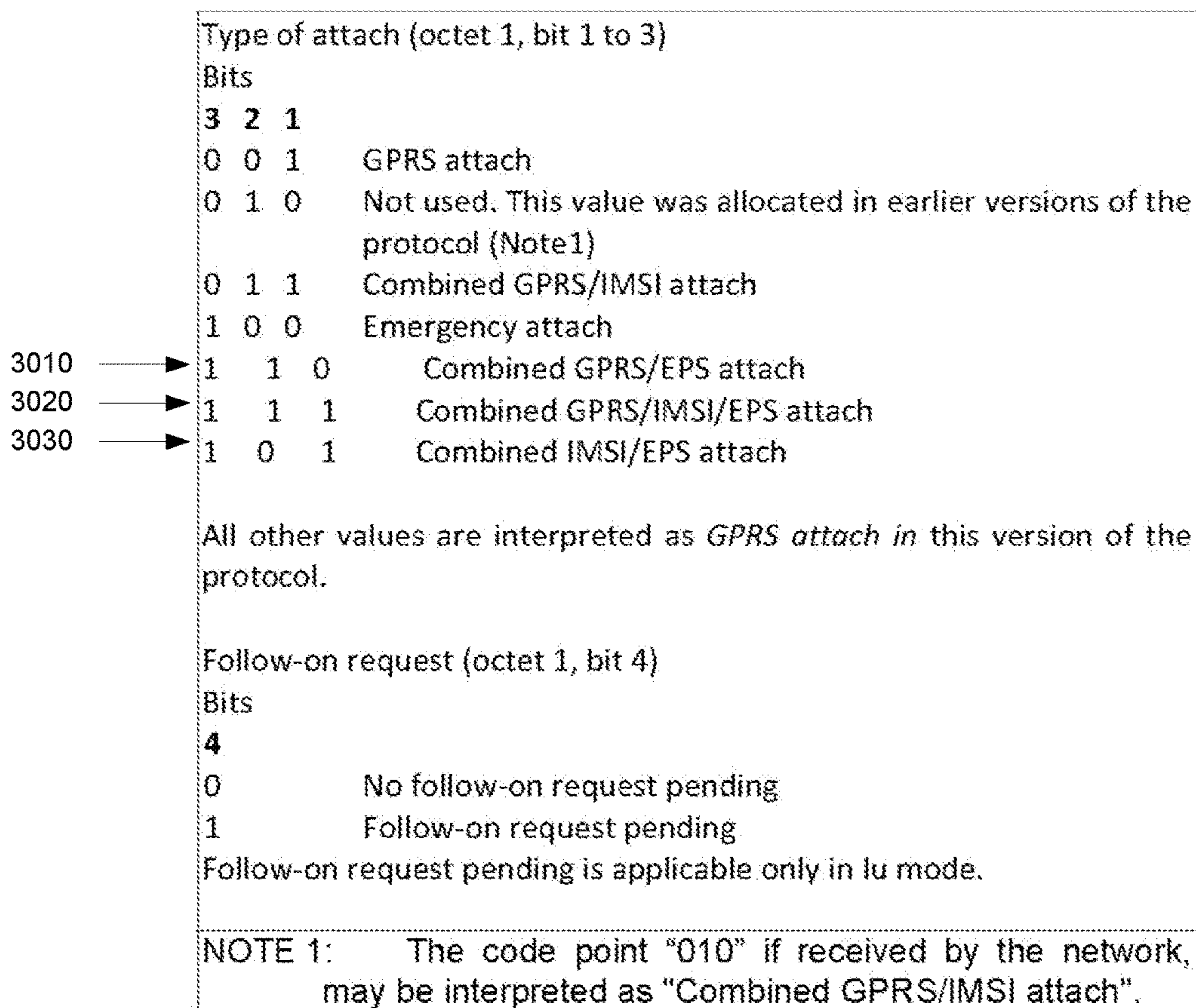
FIG. 30
