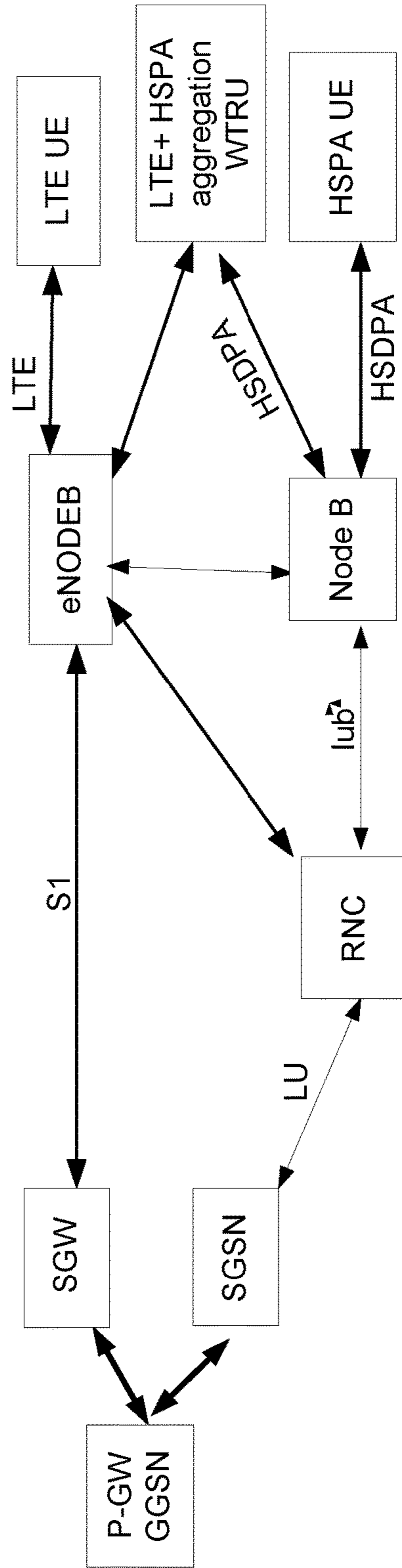
FIG. 3H
