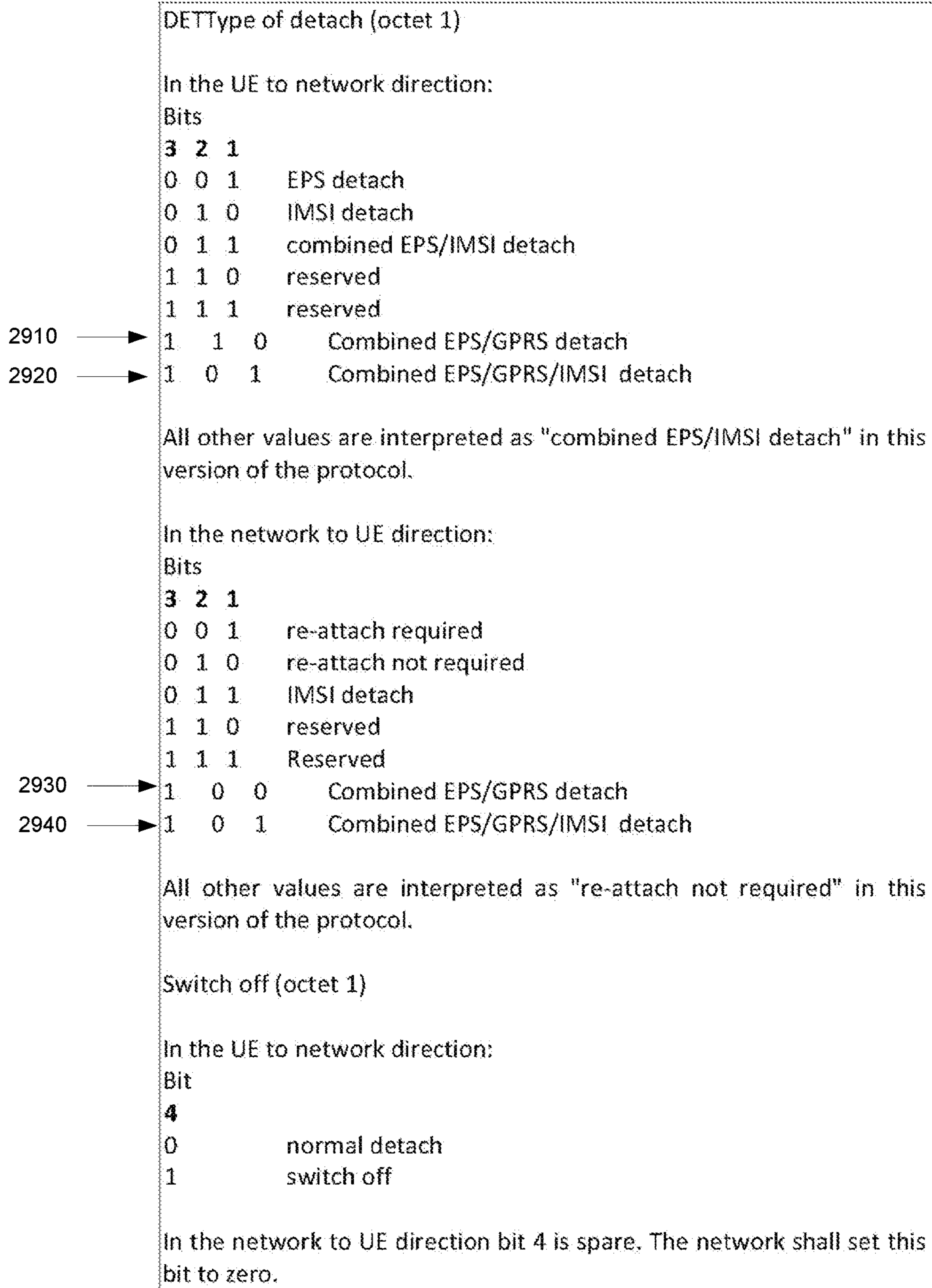
FIG. 29
