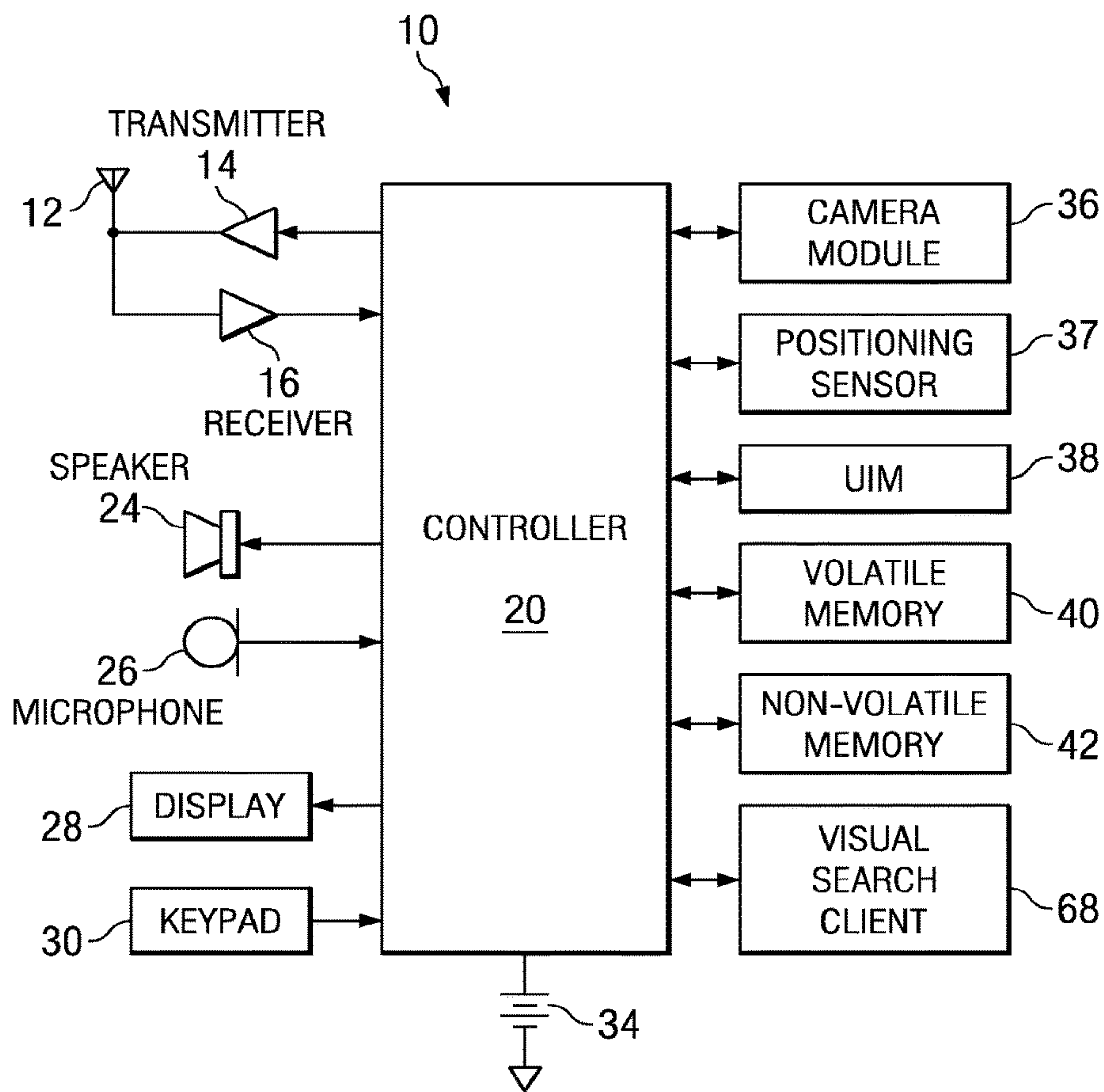
FIG. 12
