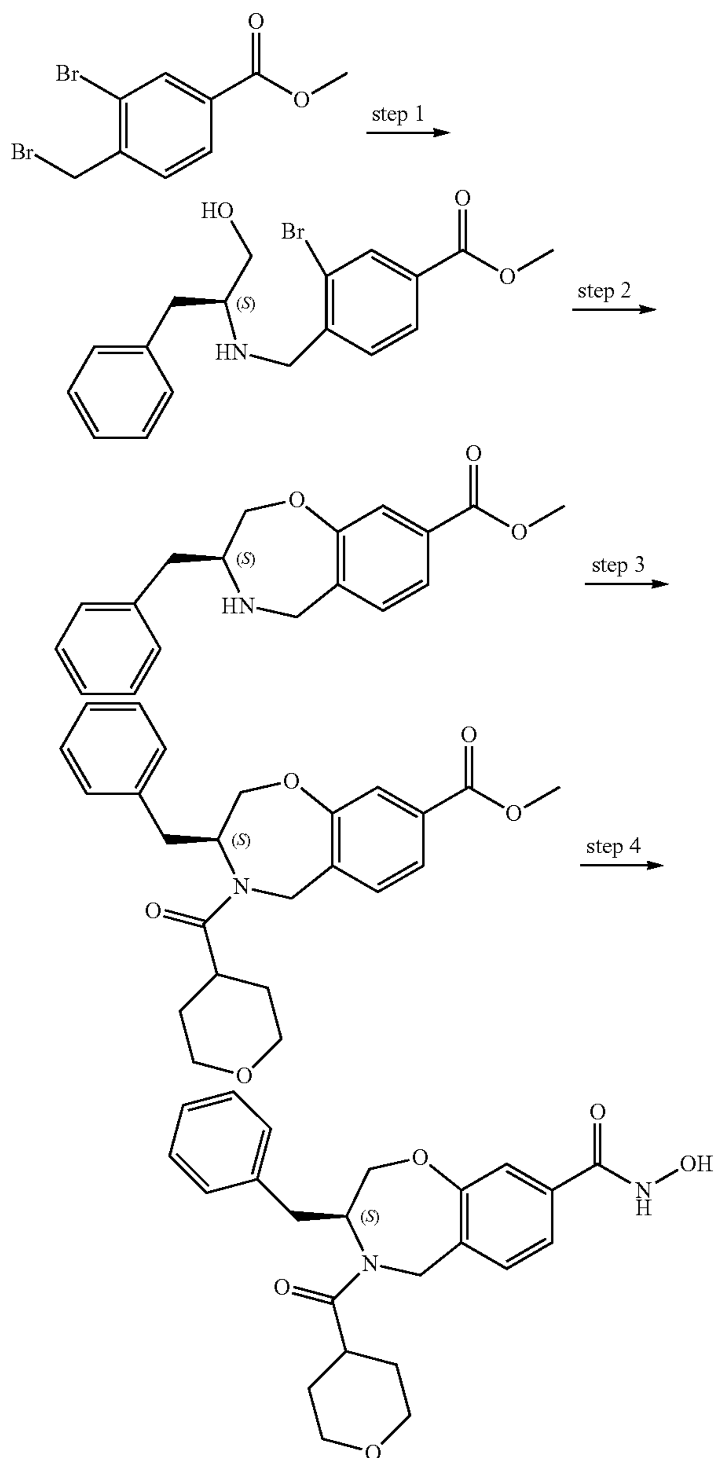
Step-1: Methyl (S)-3-bromo-4-(((1-hydroxy-3-phenylpropan-2-yl)amino)methyl)benzoate
