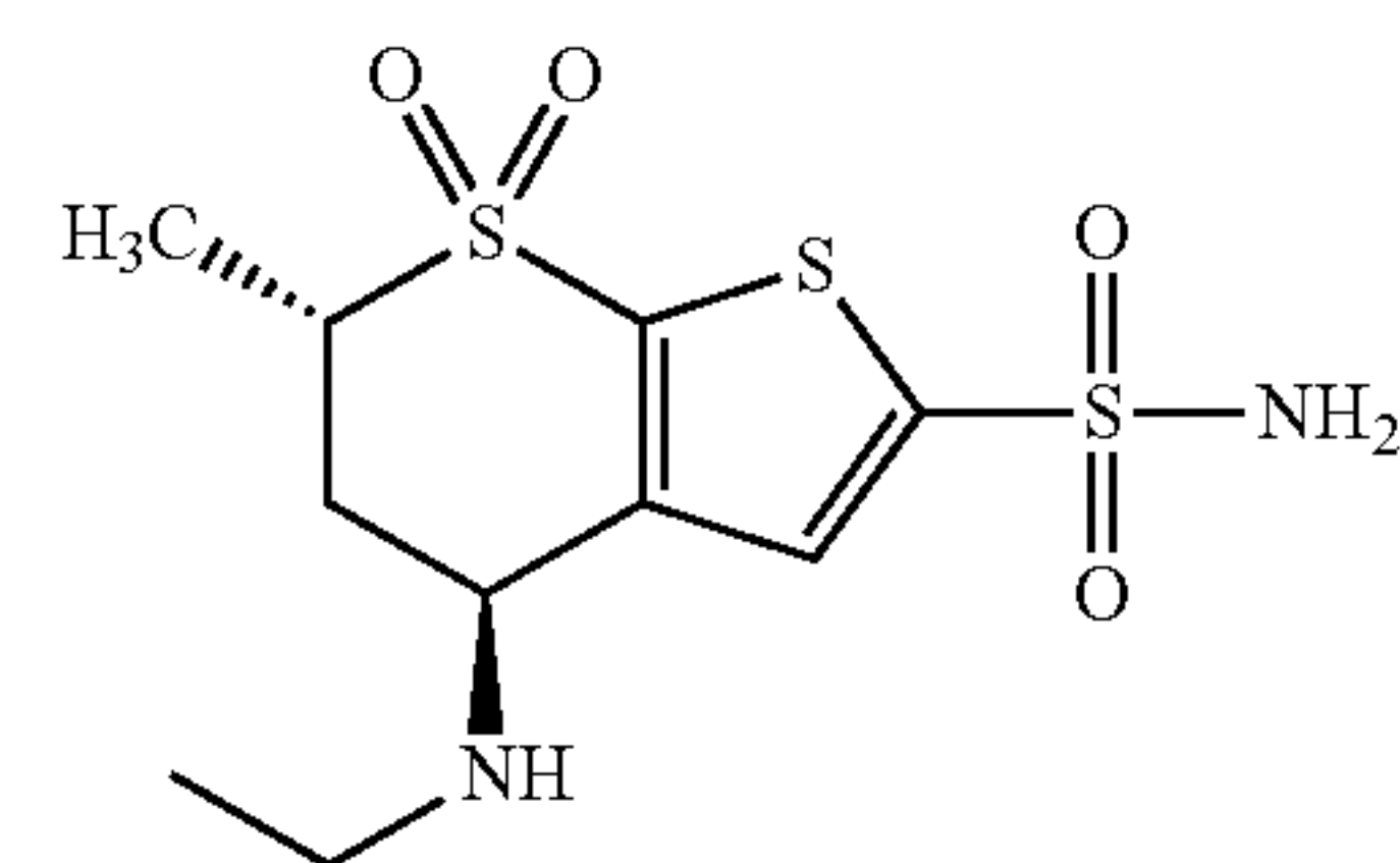
dorzolamide
