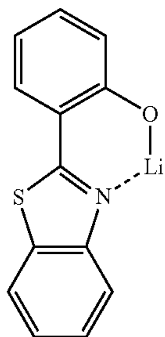
ET-D2
