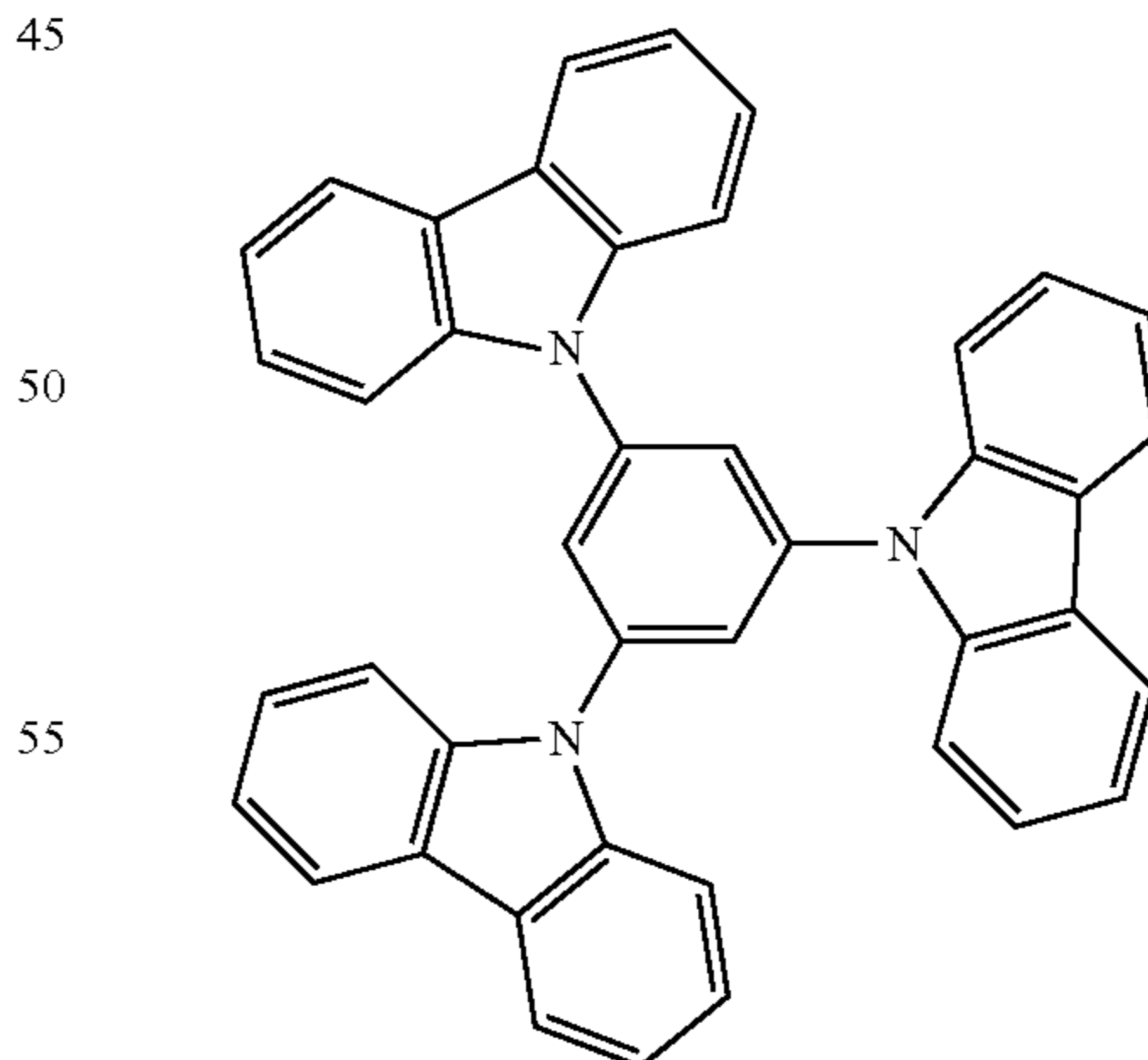
TCP
