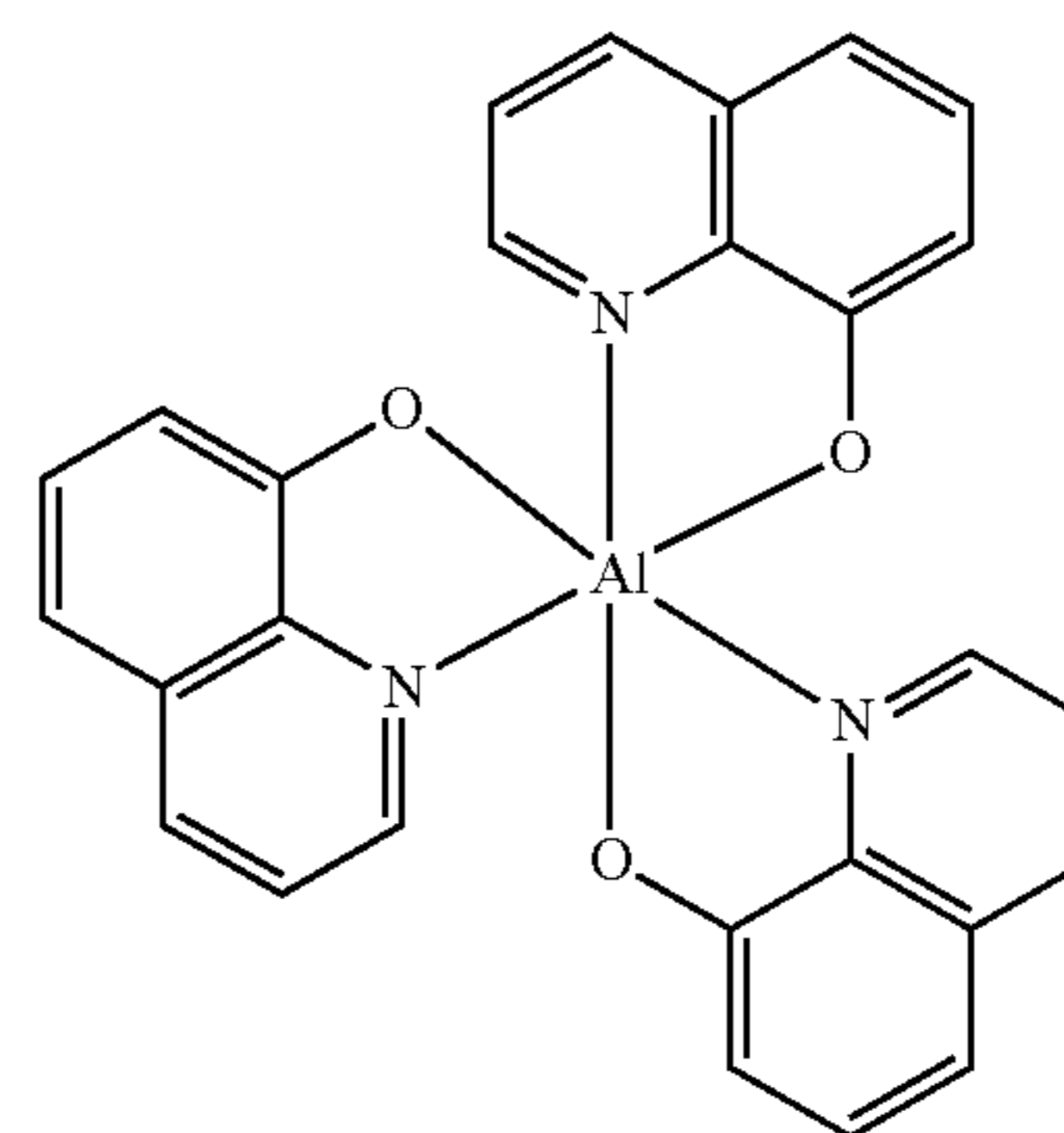
Alq 3
