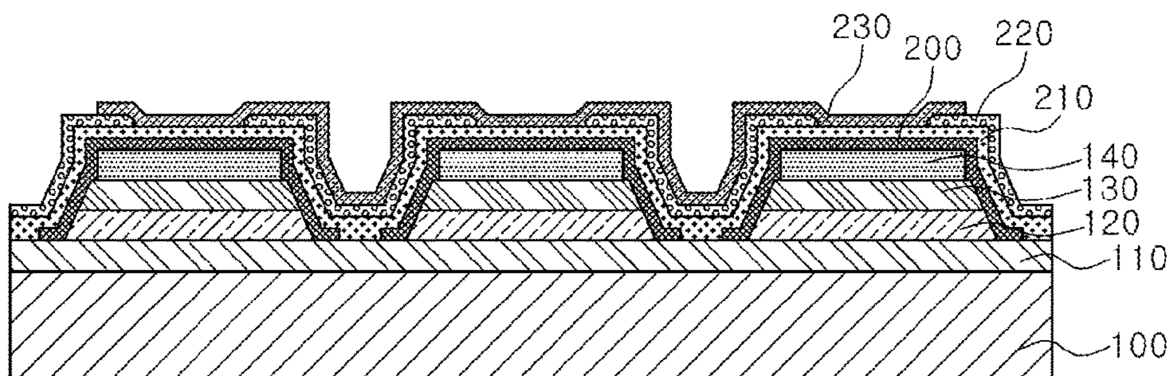
B - B'
