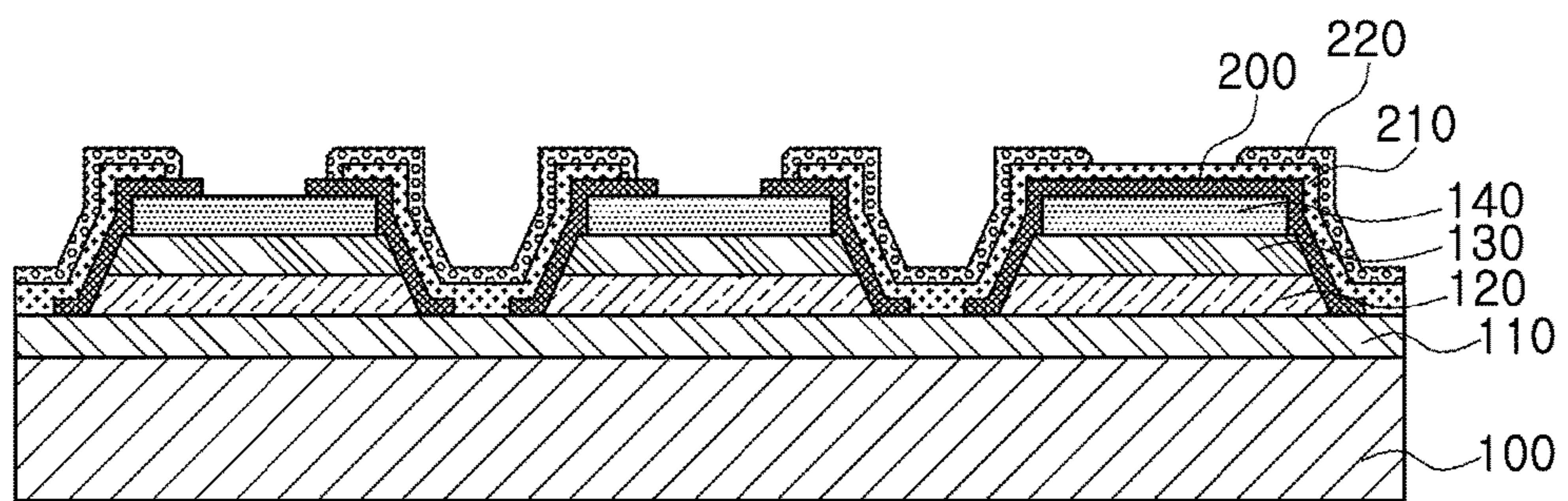
A - A'
