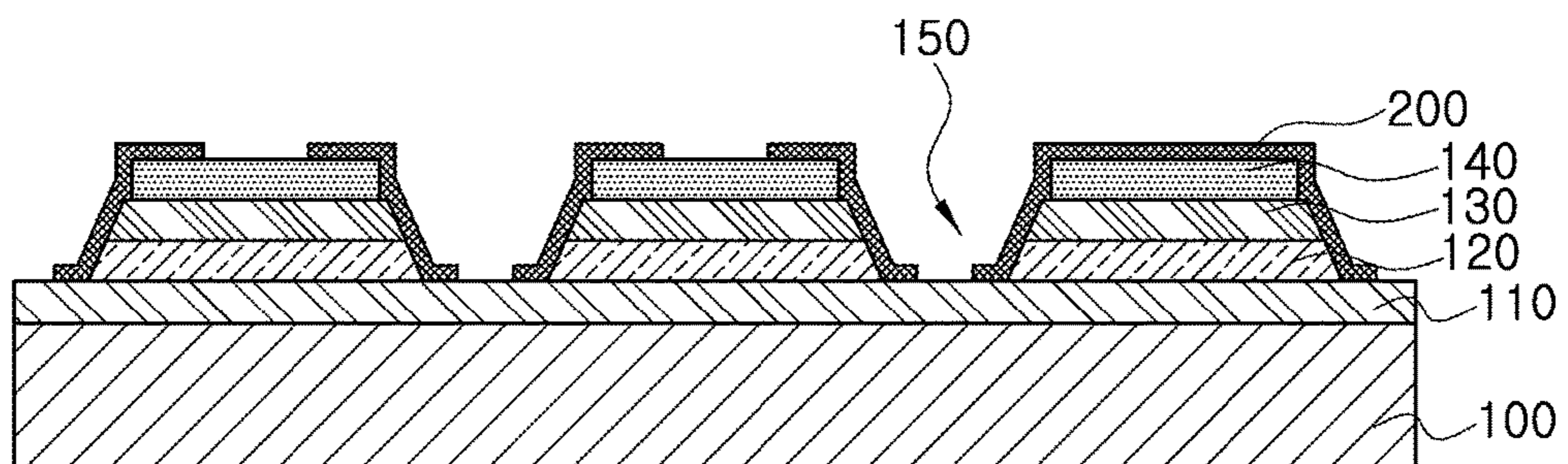
A - A'
