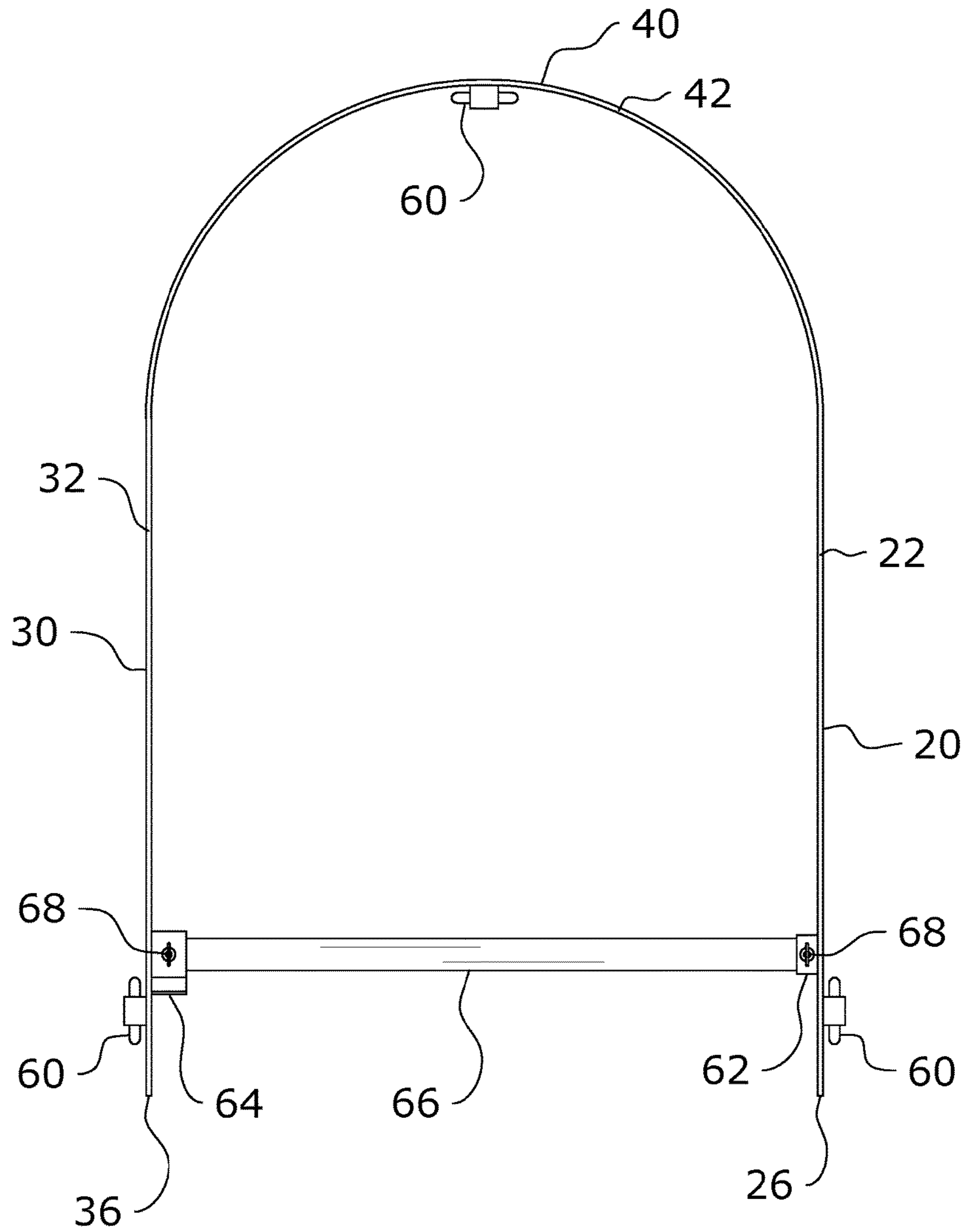
FIG. 15
