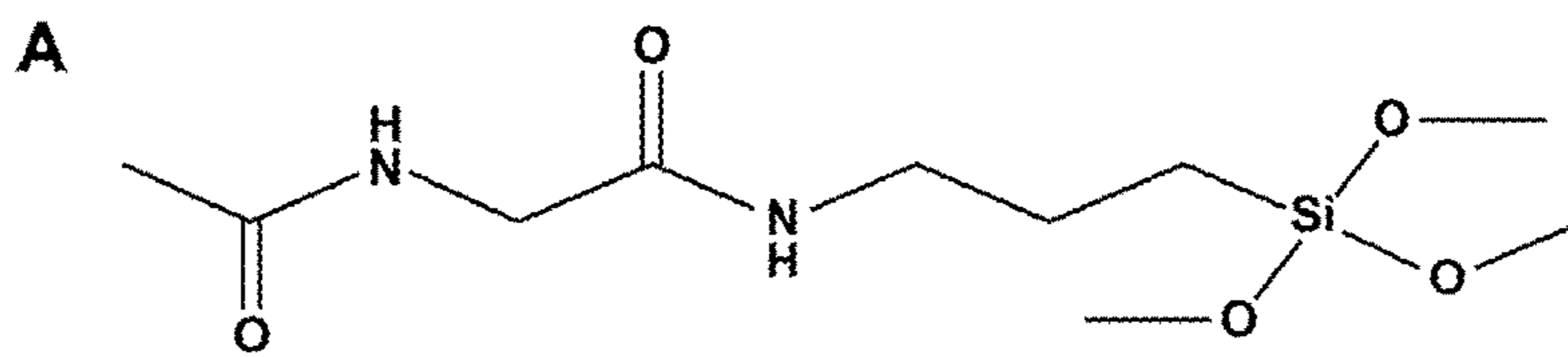
N-(Acetylglycyl)-3-aminopropyltrimethoxysilane
