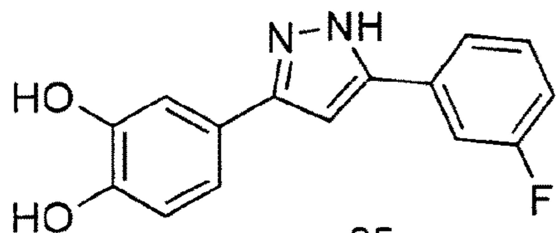
sery85 C_{15}H_{11}FN_2O_2 Mol. Wt.: 270,26
