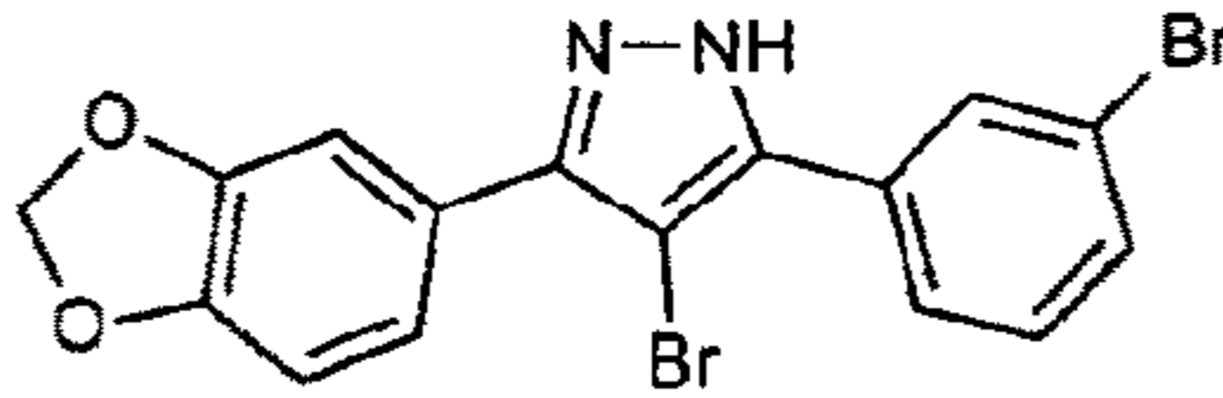
sery330 C_{16}H_{10}Br_2N_2O_2 Mol. Wt.: 422,07
