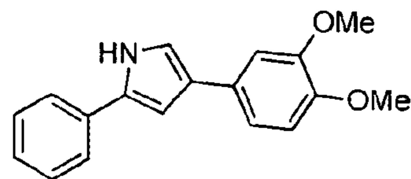
sery160 C_{18}H_{17}NO_2 Mol. Wt.: 279,33
