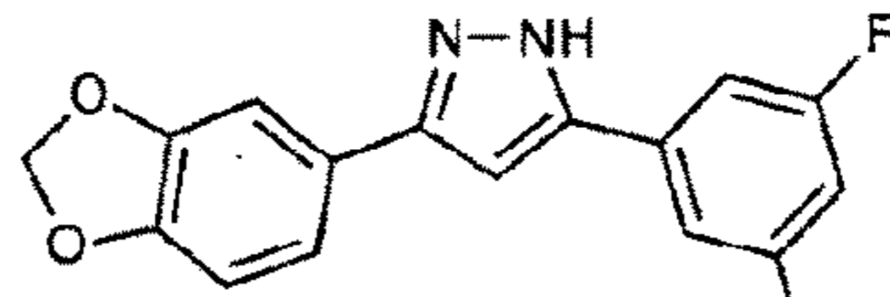
sery294b C_{15}H_{10}F_2N_2O_2 Mol. Wt.: 300,26
