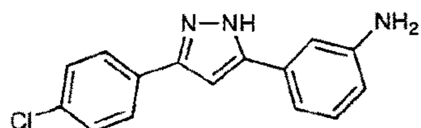
sery280a C_{15}H_{12}ClN_3 Mol. Wt.: 269,73
