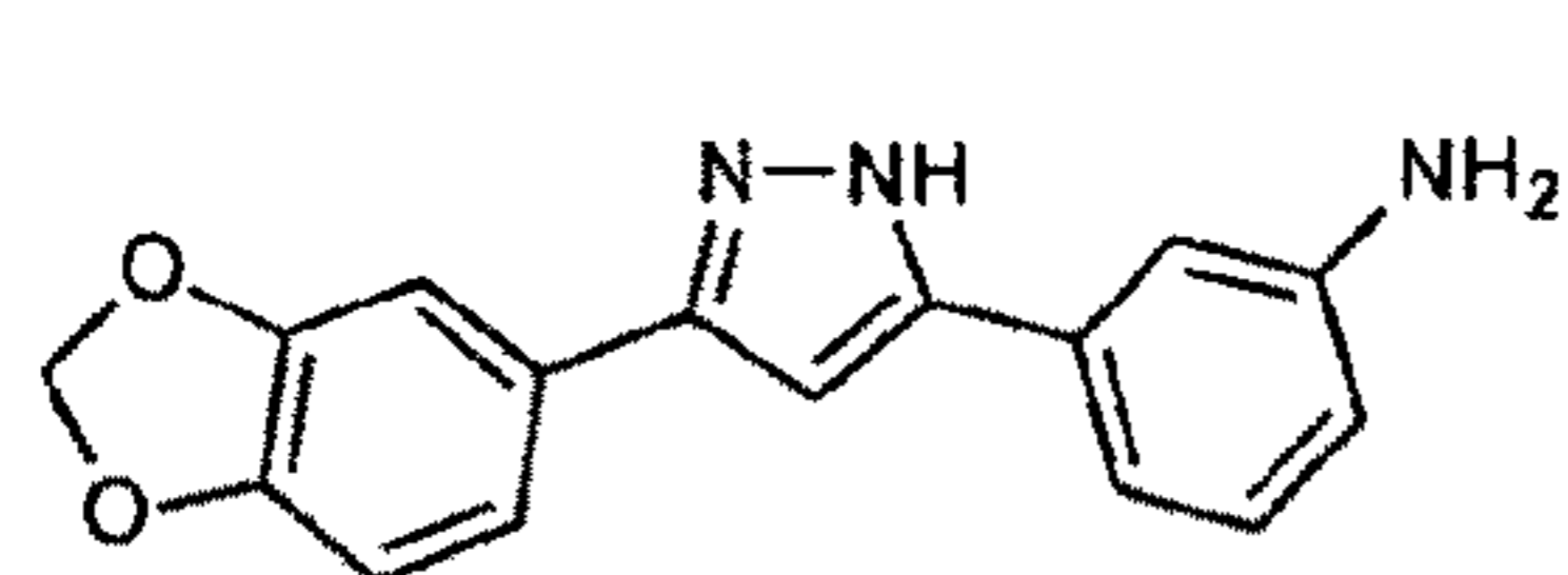
sery308 C_{16}H_{13}N_3O_2 Mol. Wt.: 279,29
