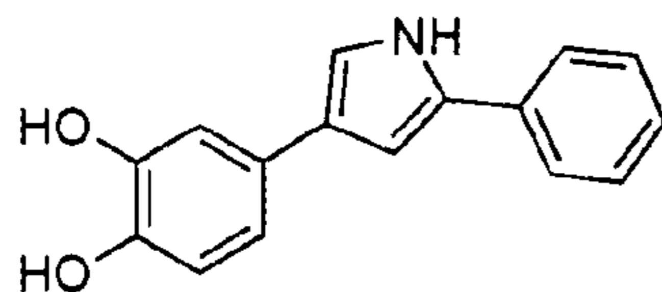
sery166b C_{16}H_{13}NO_2 Mol. Wt.: 251,28
