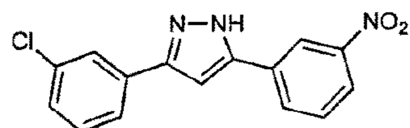
sery275a C_{15}H_{10}ClN_3O_2 Mol. Wt.: 299,71
