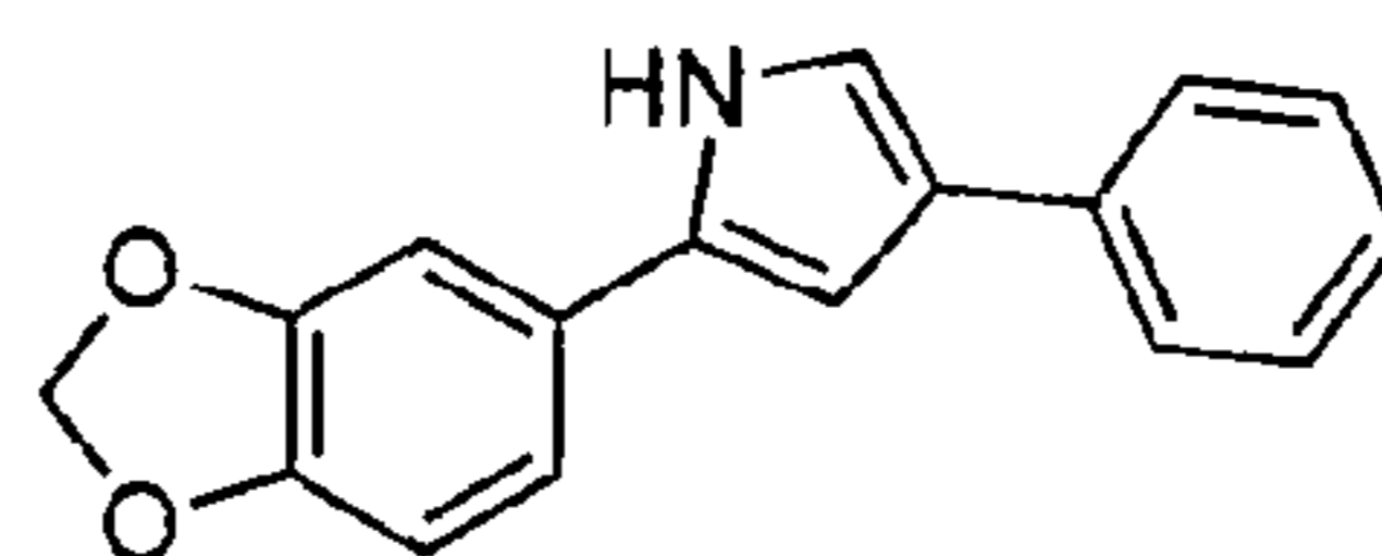
anle130b C_{17}H_{13}NO_2 Mol. Wt.: 263,29
