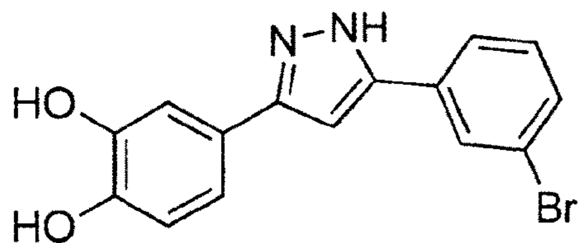
anle138c C_{15}H_{11}BrN_2O_2 Mol. Wt.: 331,16
