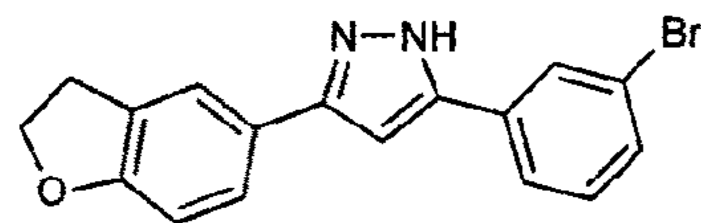
sery312b C_{17}H_{13}BrN_2O Mol. Wt.: 341,2
