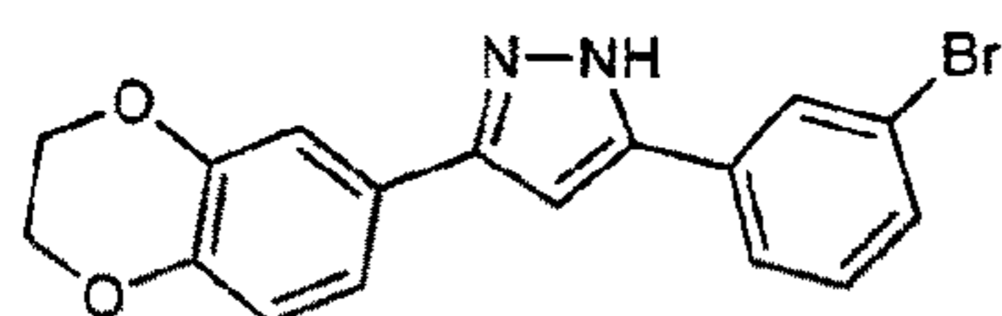
sery315b C_{17}H_{13}BrN_2O_2 Mol. Wt.: 357,2
