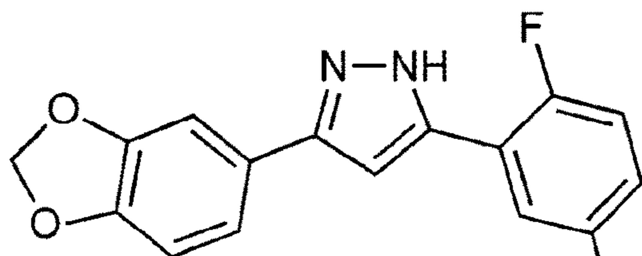
sery316b C_{16}H_{10}F_2N_2O_2 Mol. Wt.: 300,26
