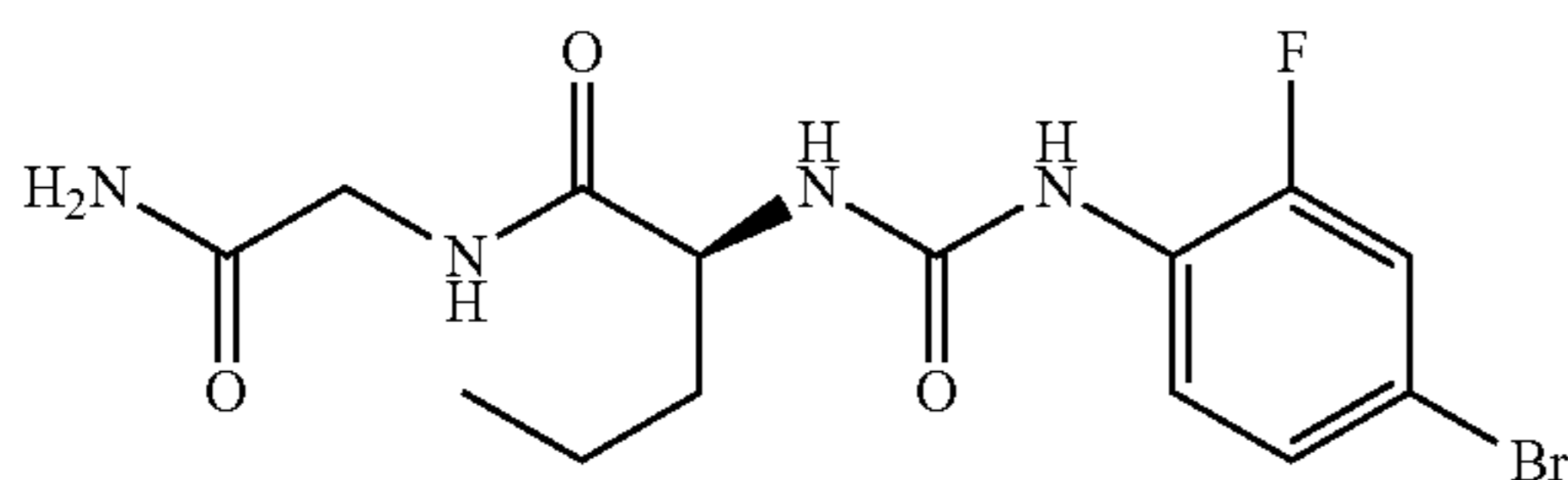
(2S)-N-(2-amino-2-oxoethyl)-2-[[4-bromo-2-fluorophenyl]carbamoyl]amino pentanamide
