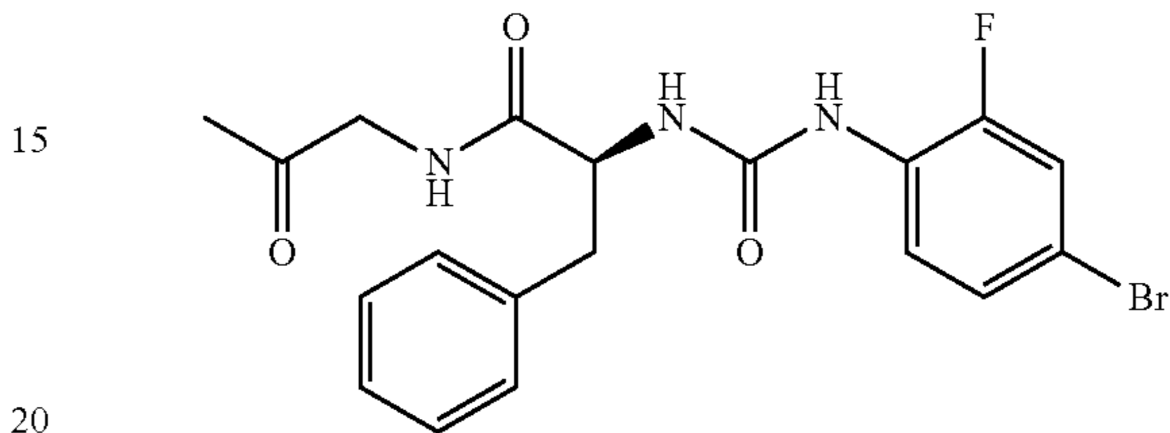
(2S)-2-{{(4-bromo-2-fluorophenyl)carbamoyl}amino}-N-(2-oxopropyl)-3-phenylpropanamide
