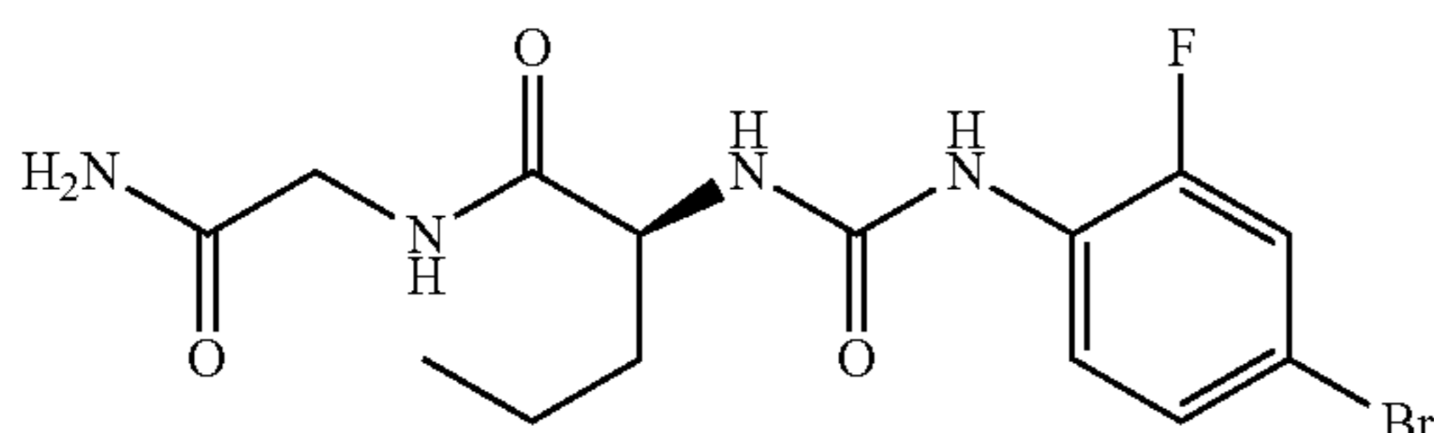
(2S)-N-(2-amino-2-oxoethyl)-2-[[4-bromo-2-fluorophenyl]carbamoyl]amino pentanamide
