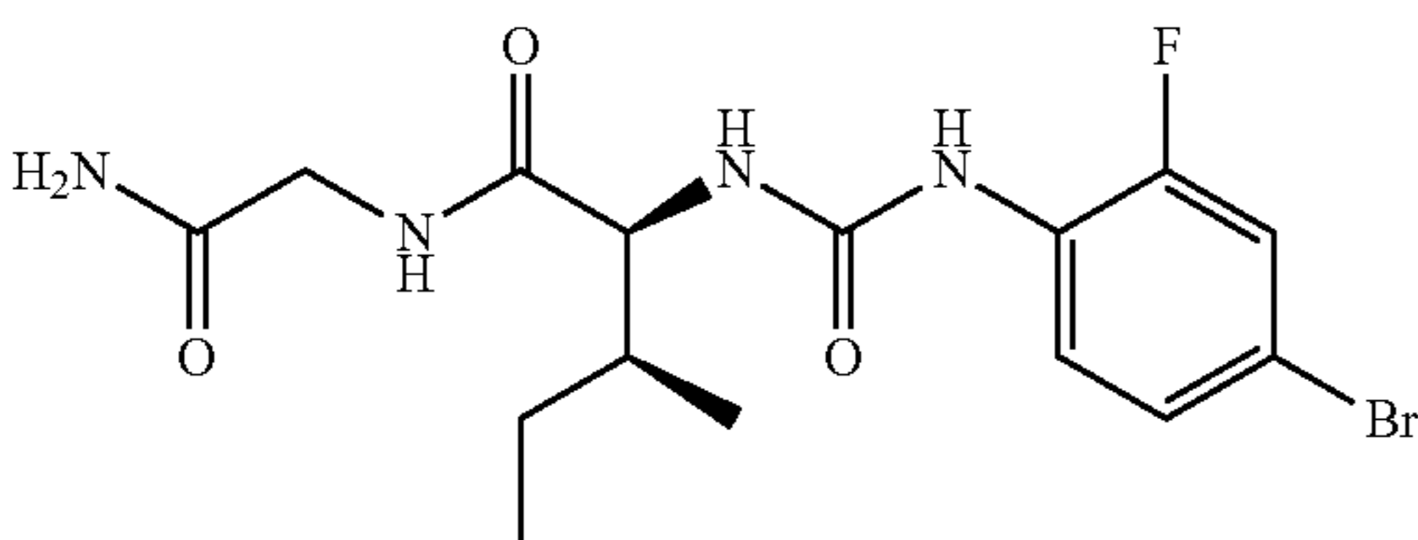
(2S,3S)-N-(2-amino-2-oxoethyl)-2-{{(4-bromo-2-fluorophenyl)carbamoyl}amino}-3-methylpentanamide
