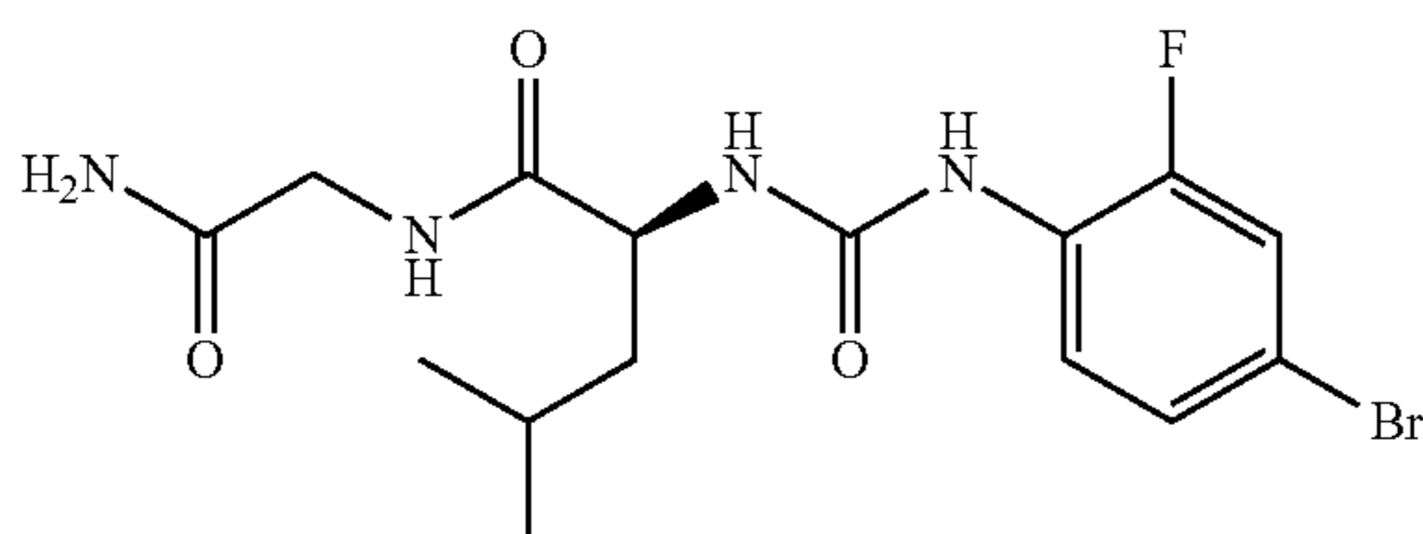
(2S)-N-(2-amino-2-oxoethyl)-2-[[4-bromo-2-fluorophenyl]carbamoyl]amino-4-methylpentanamide
