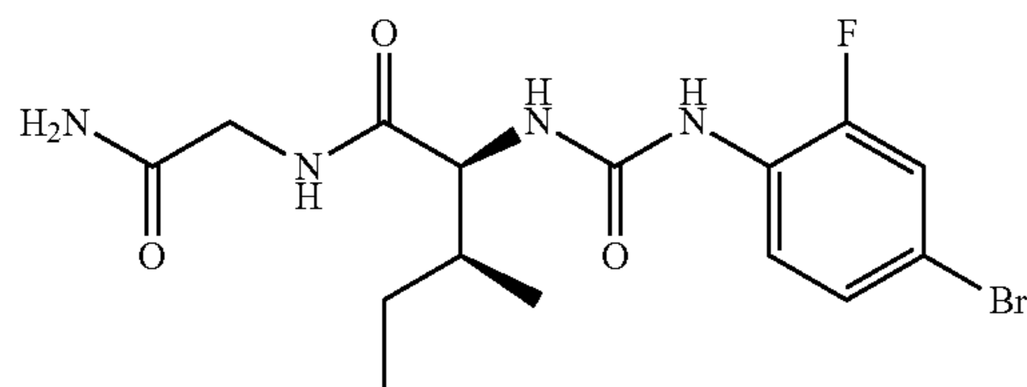
(2S,3S)-N-(2-amino-2-oxoethyl)-2-{{(4-bromo-2-fluorophenyl)carbamoyl}amino}-3-methylpentanamide
