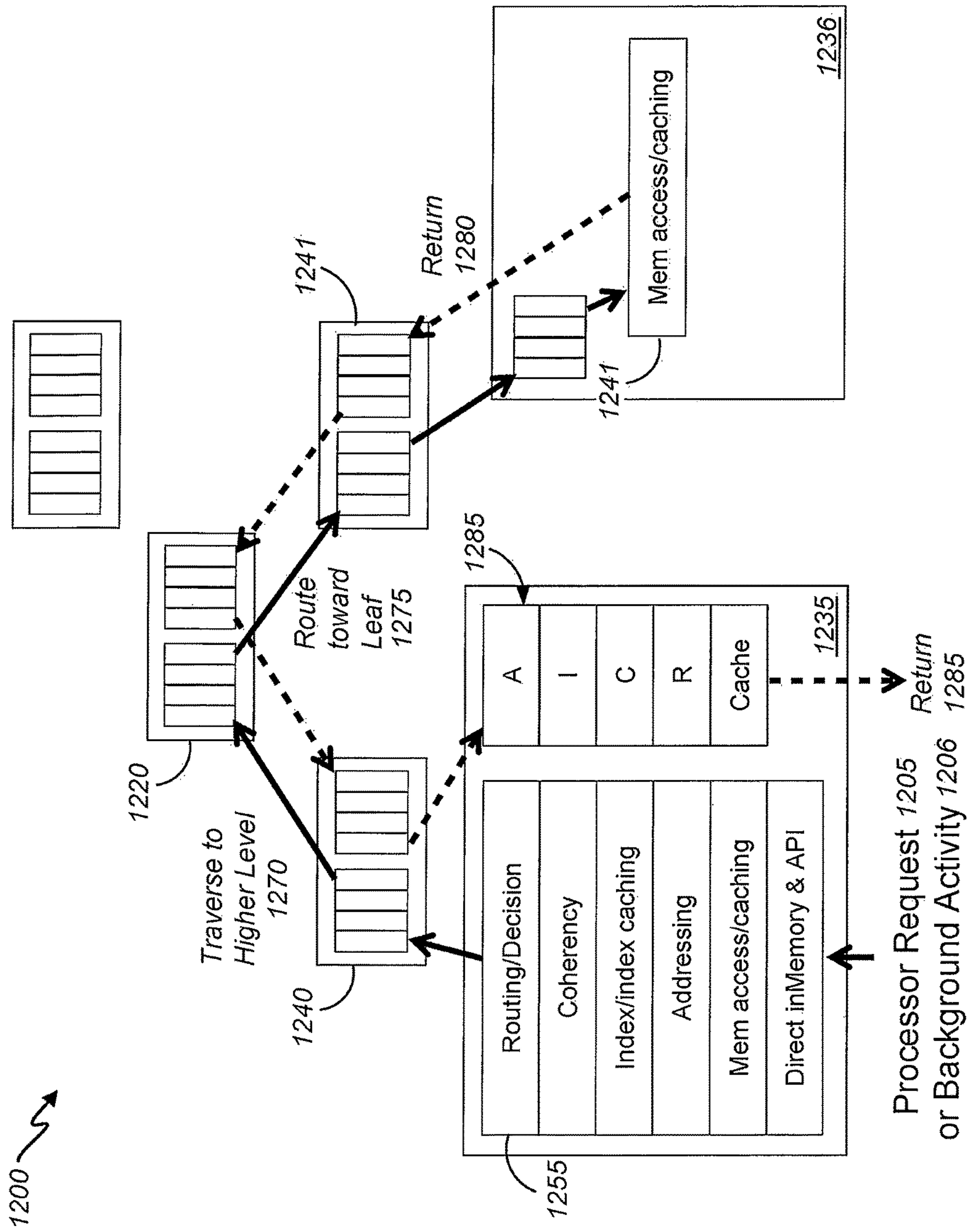
FIG. 12
