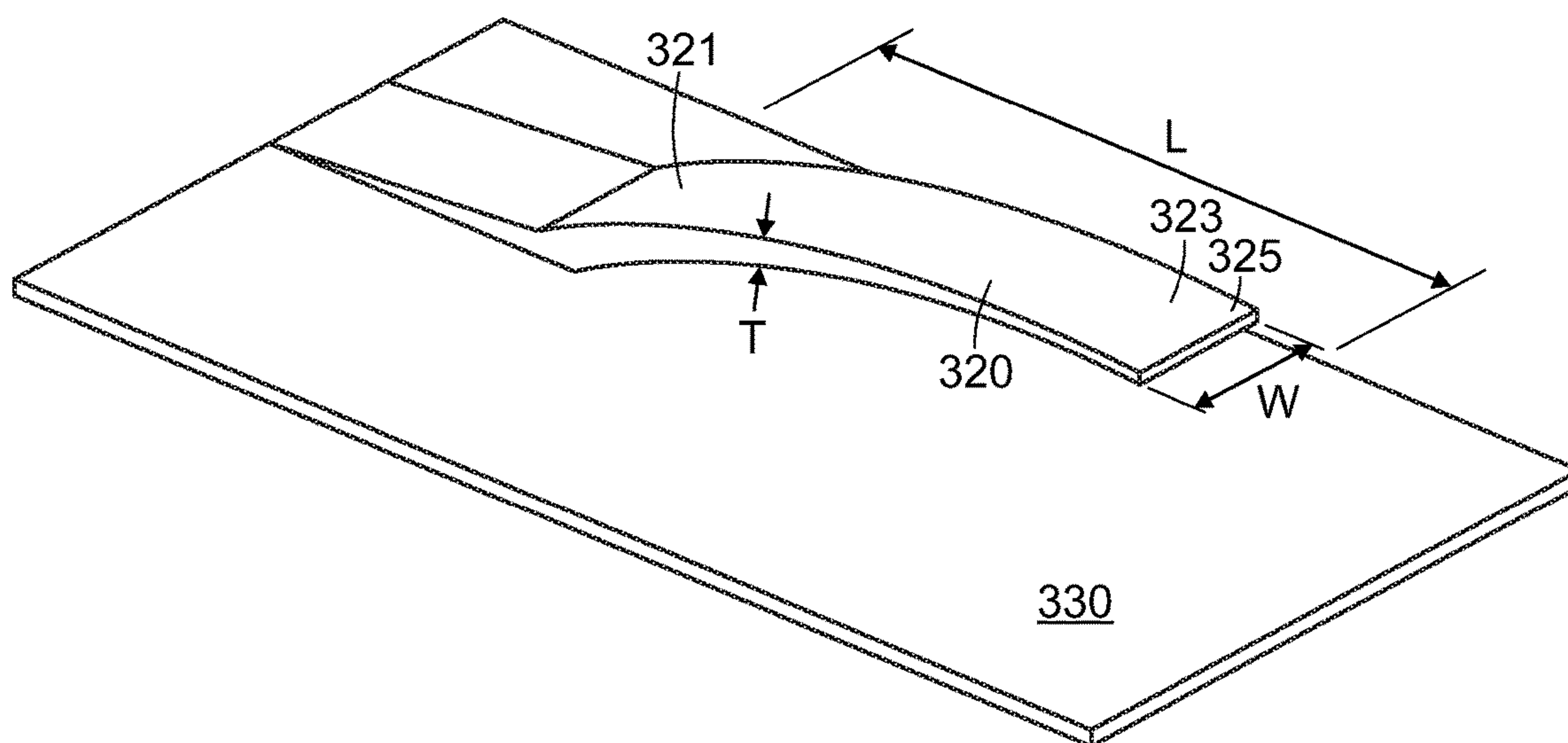
FIG. 7A
