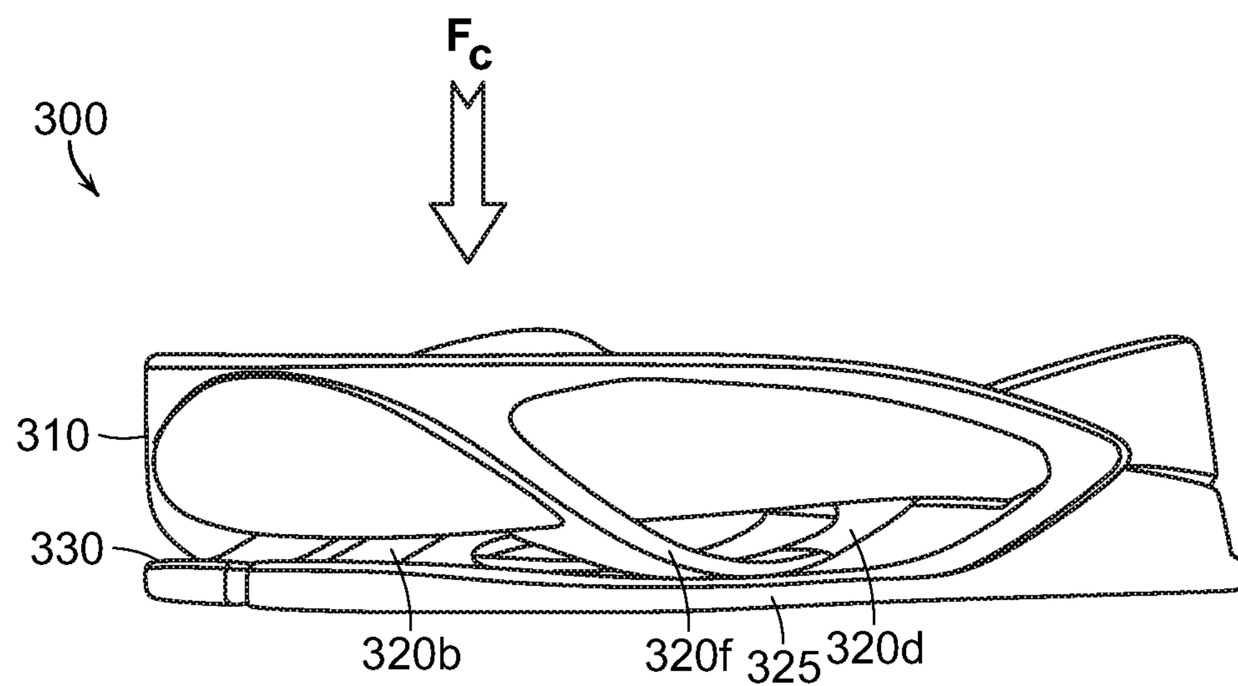
FIG. 9A
