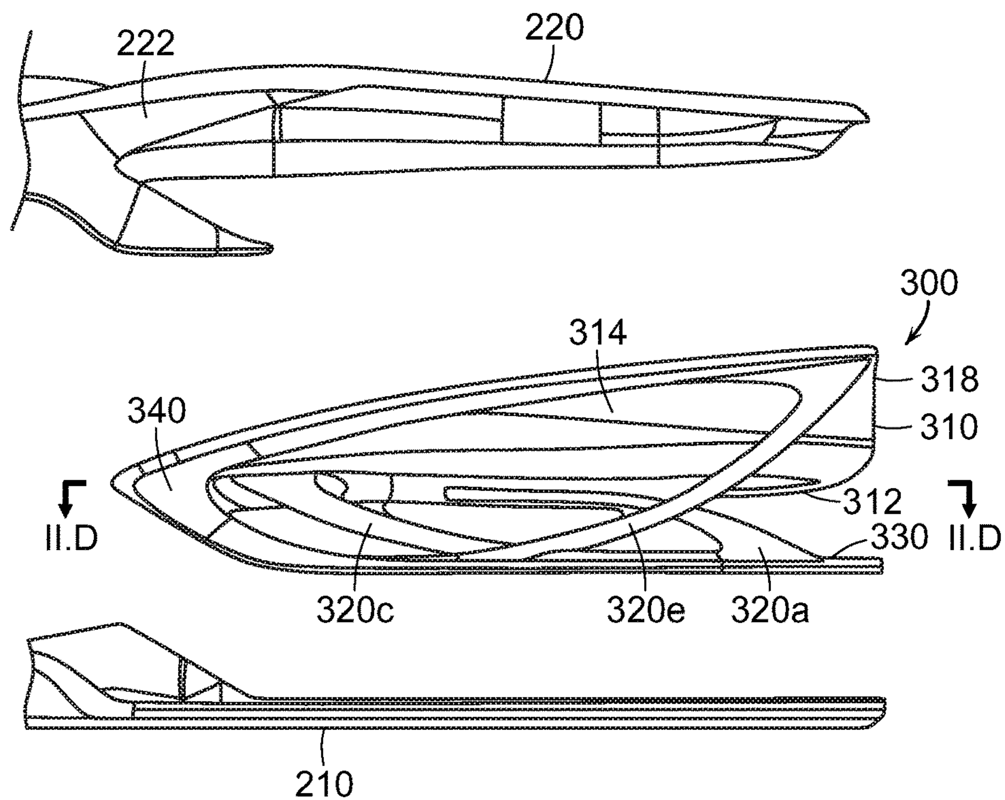
FIG. 2C
