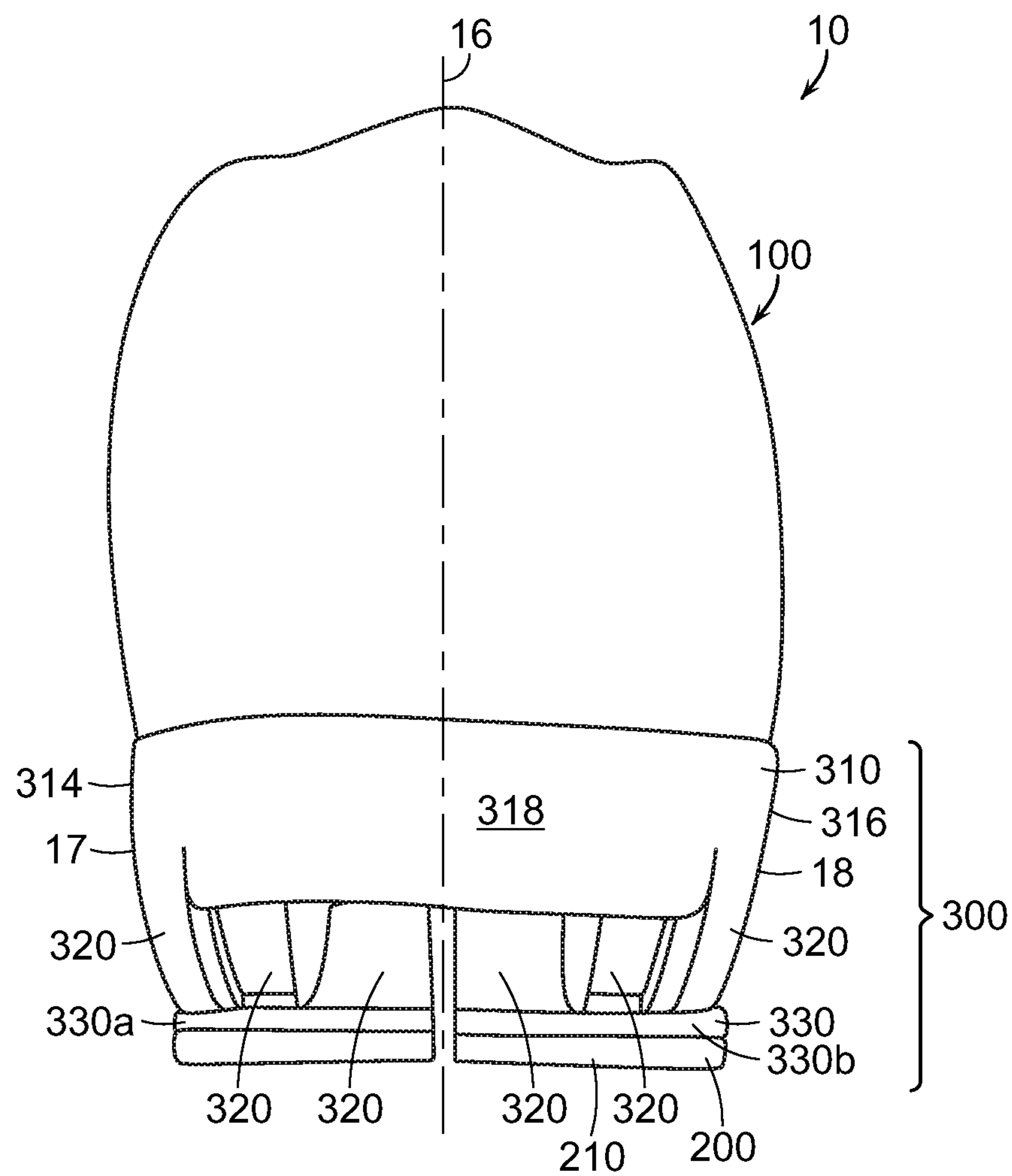
FIG. 1B
