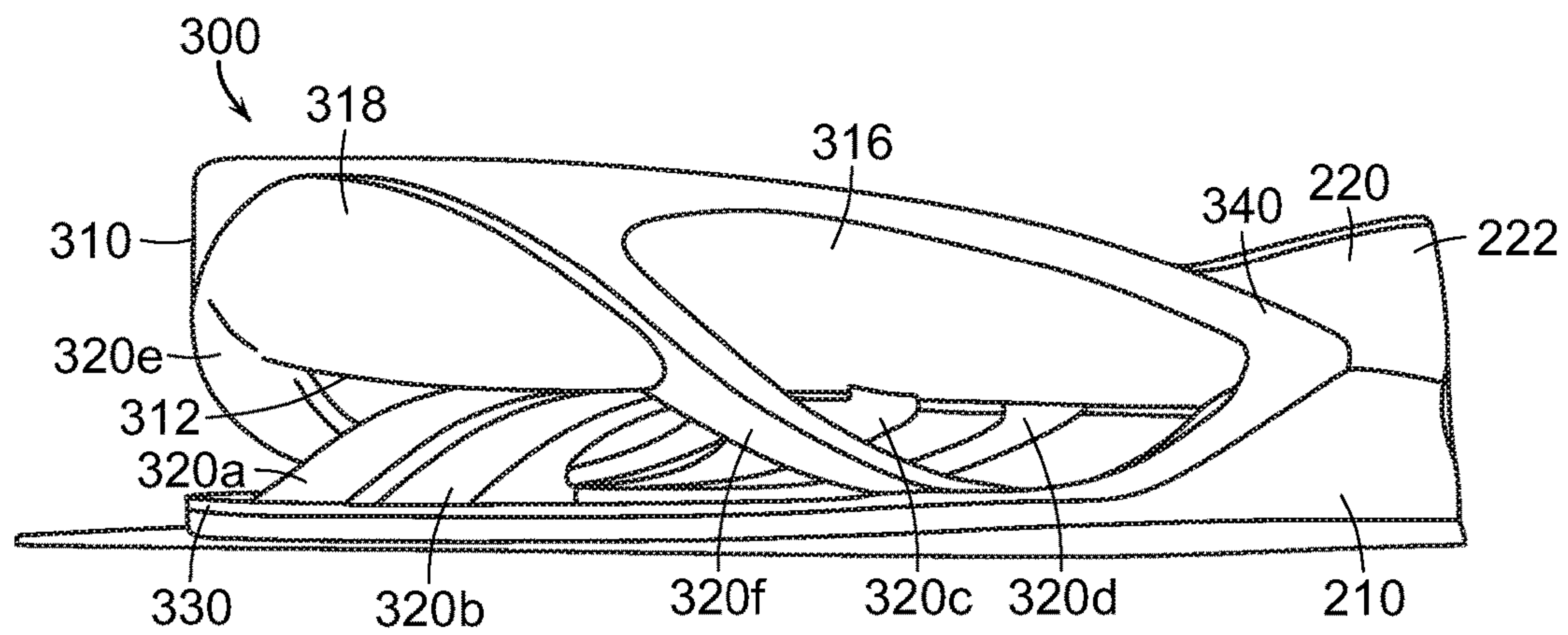
FIG. 2A
