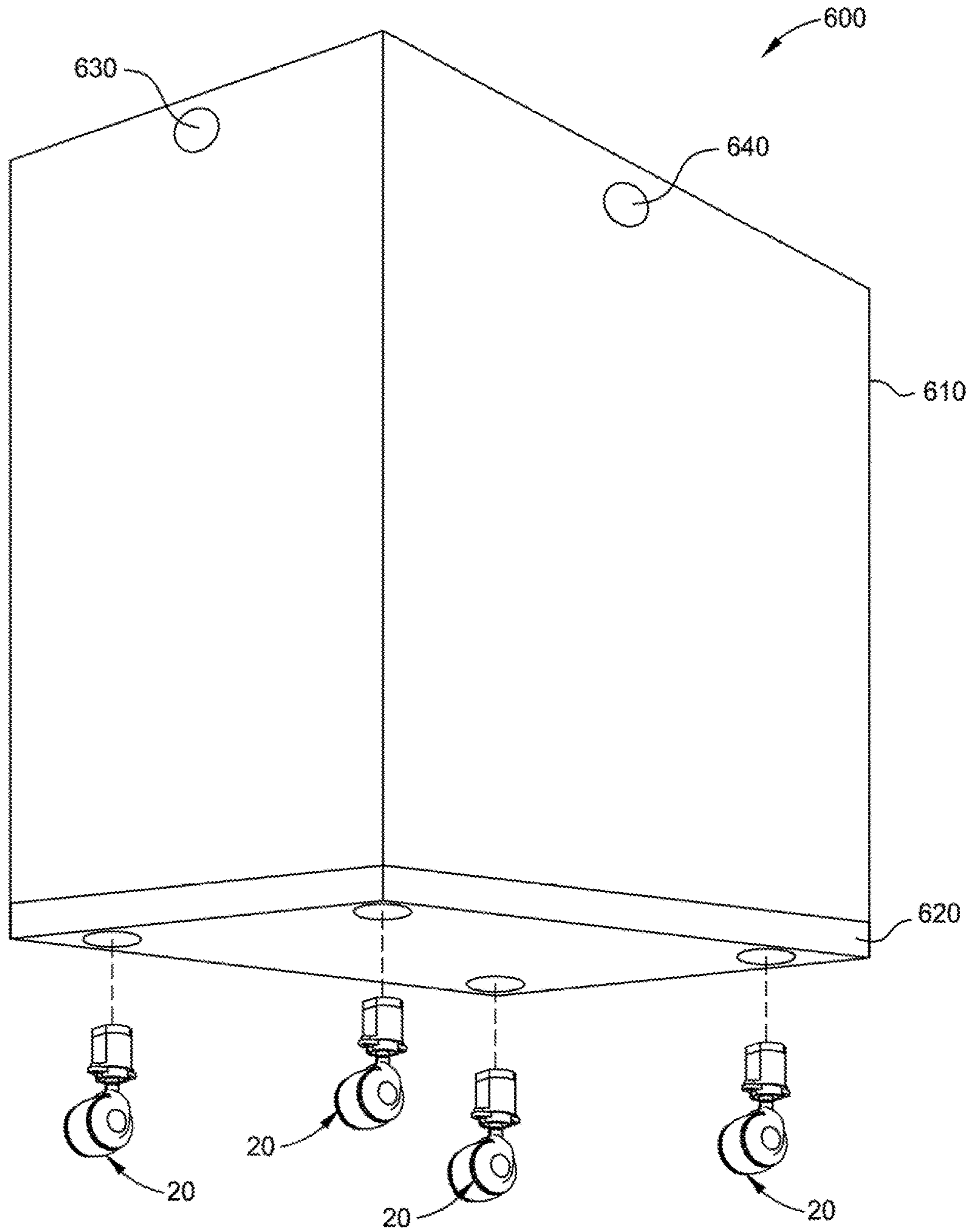
FIG. 10
