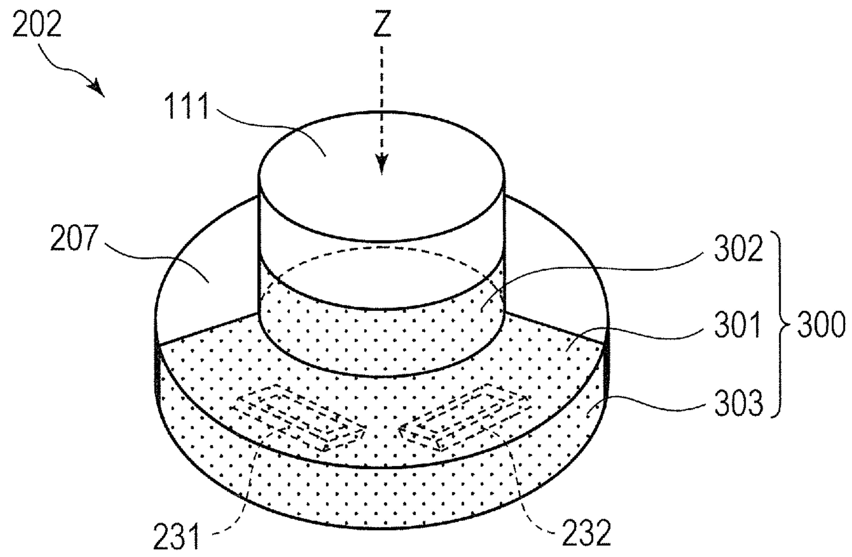
FIG. 4A
