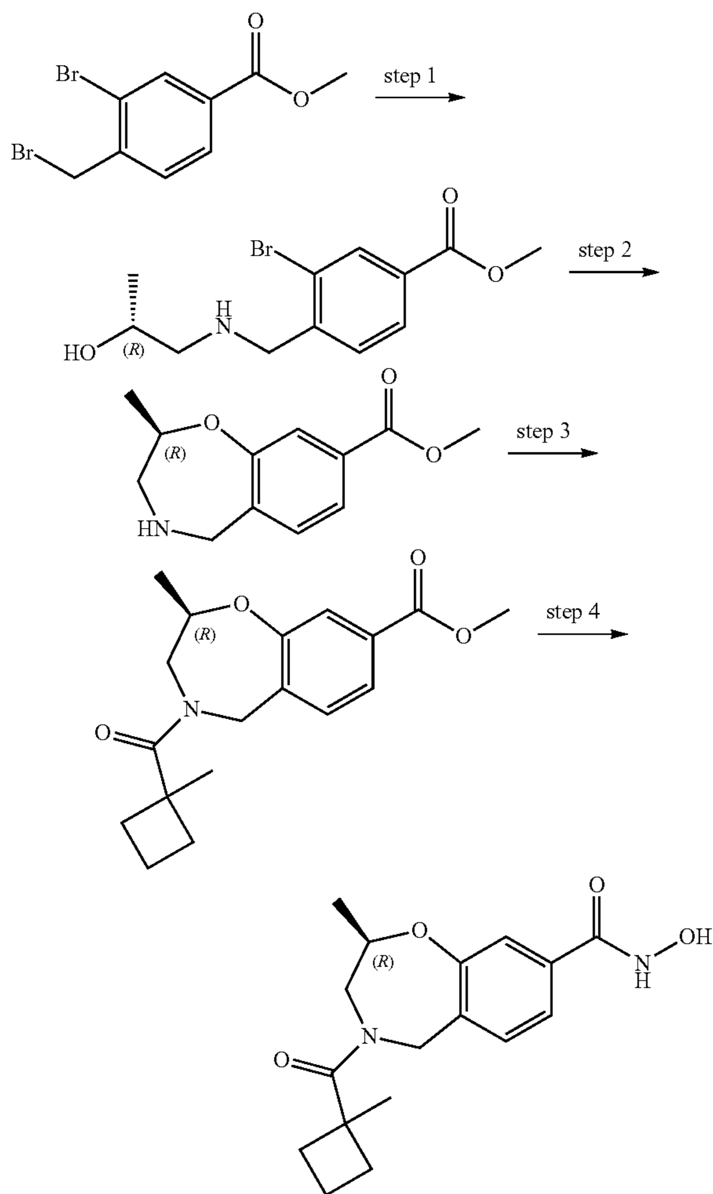
Step-1: Methyl (R)-3-bromo-4-(((2-hydroxypropyl)amino)methyl)benzoate
