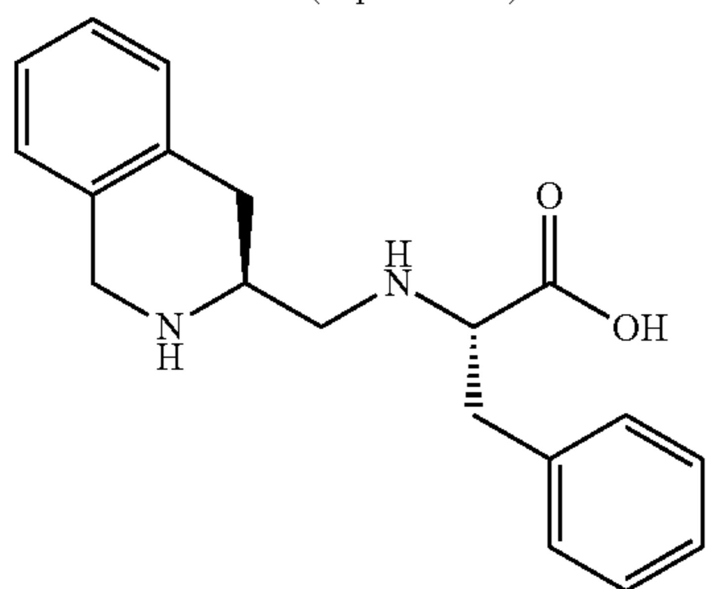
(Tic-Ψ[CH2—NH]-Ψ-Phe)
