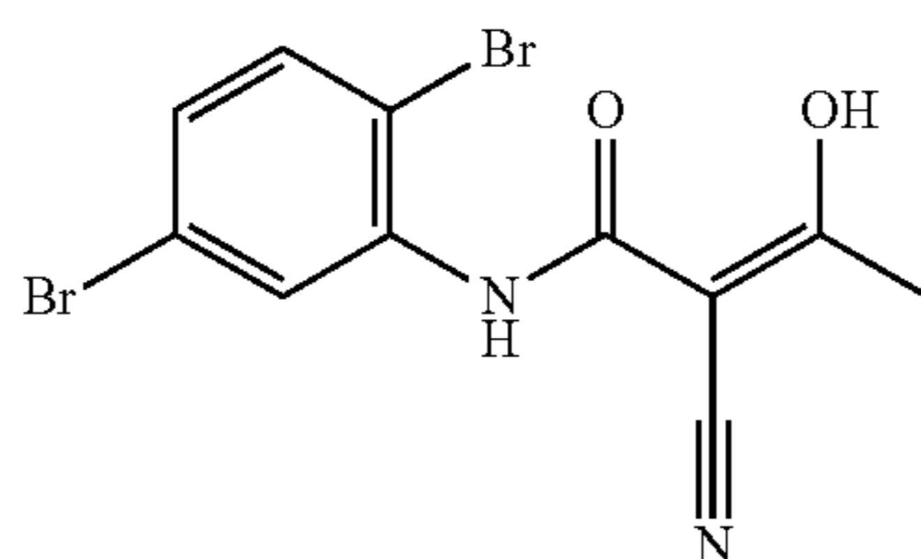
LFM-A13
