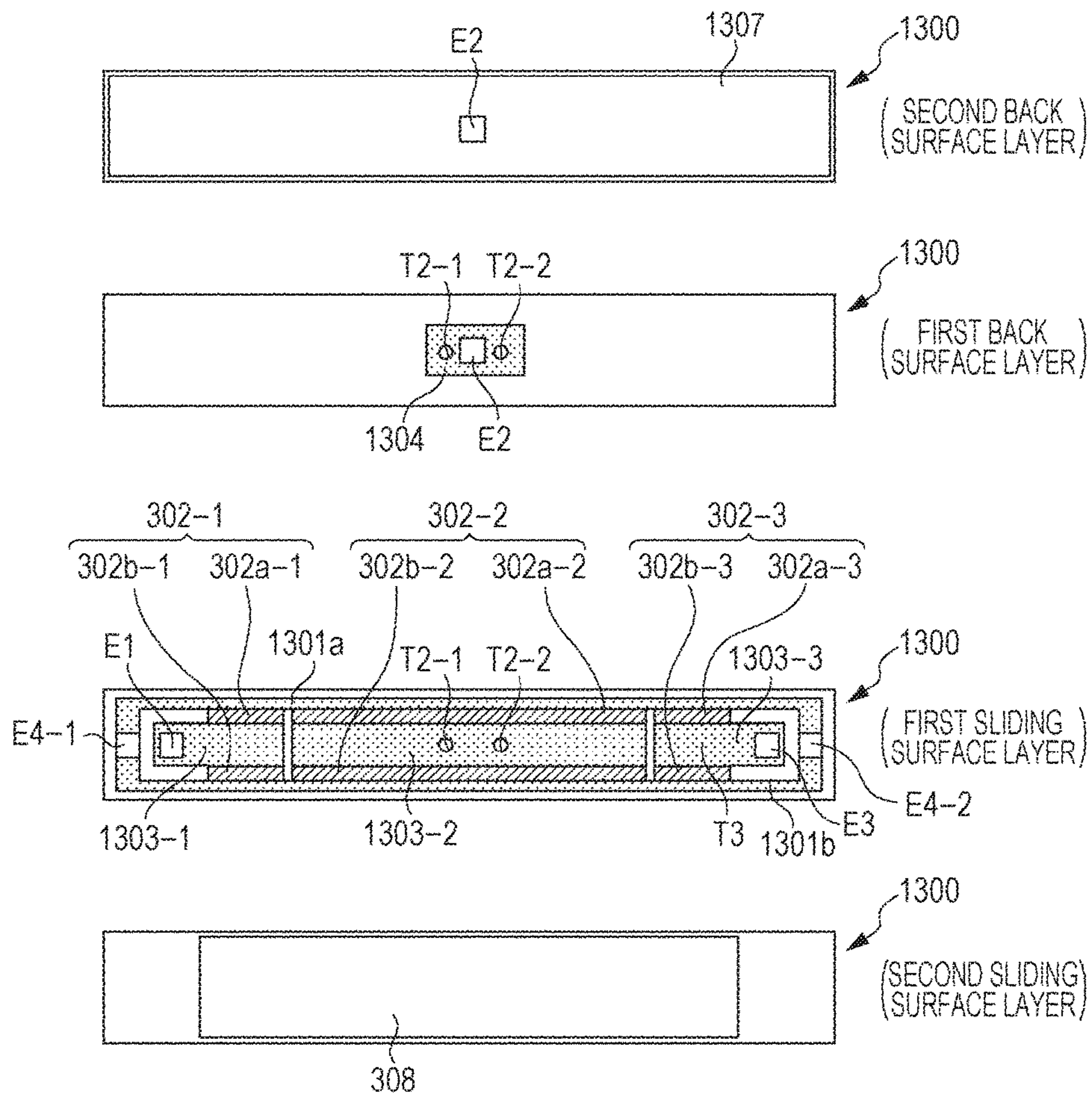
FIG. 13B
