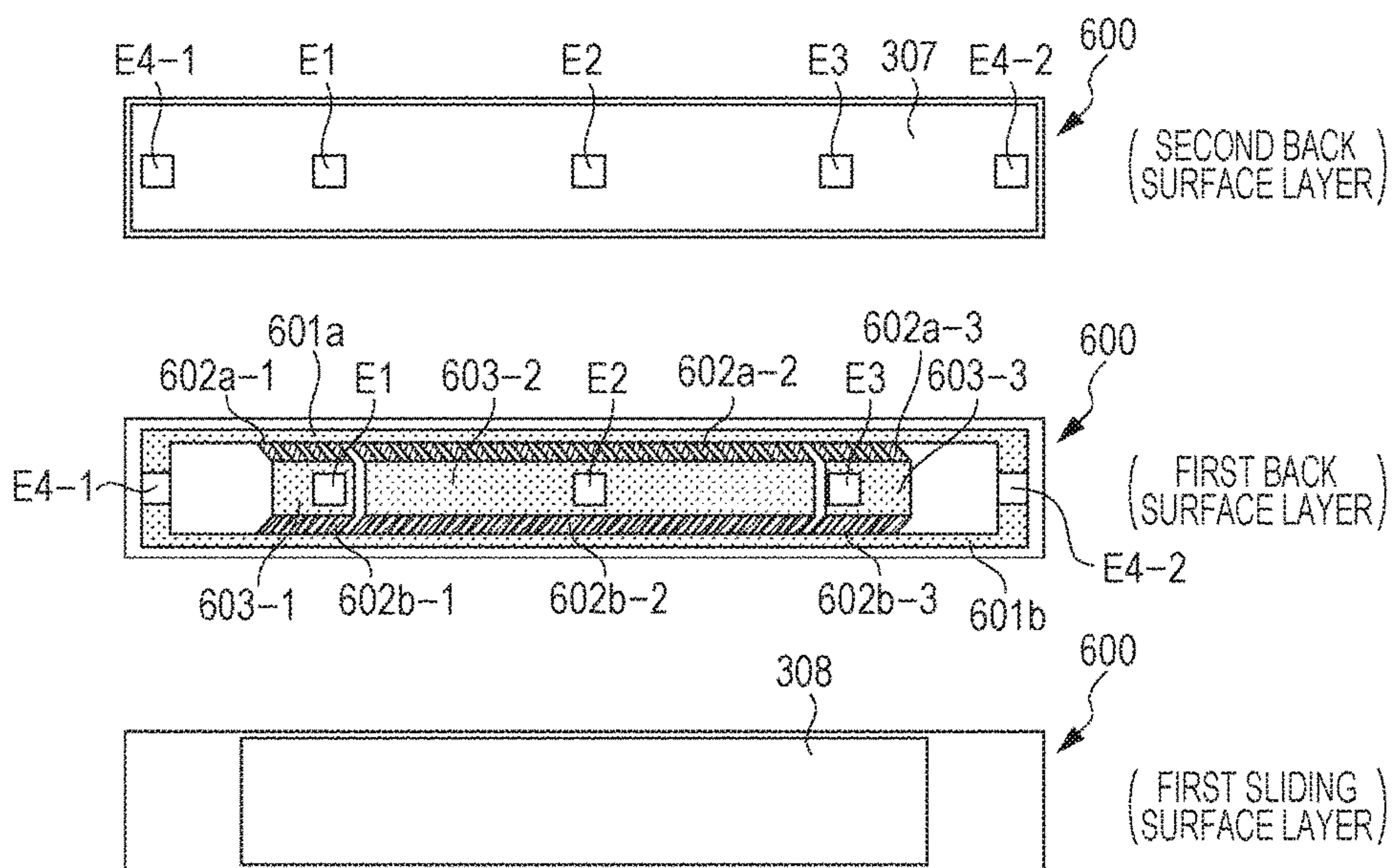
FIG. 12B
