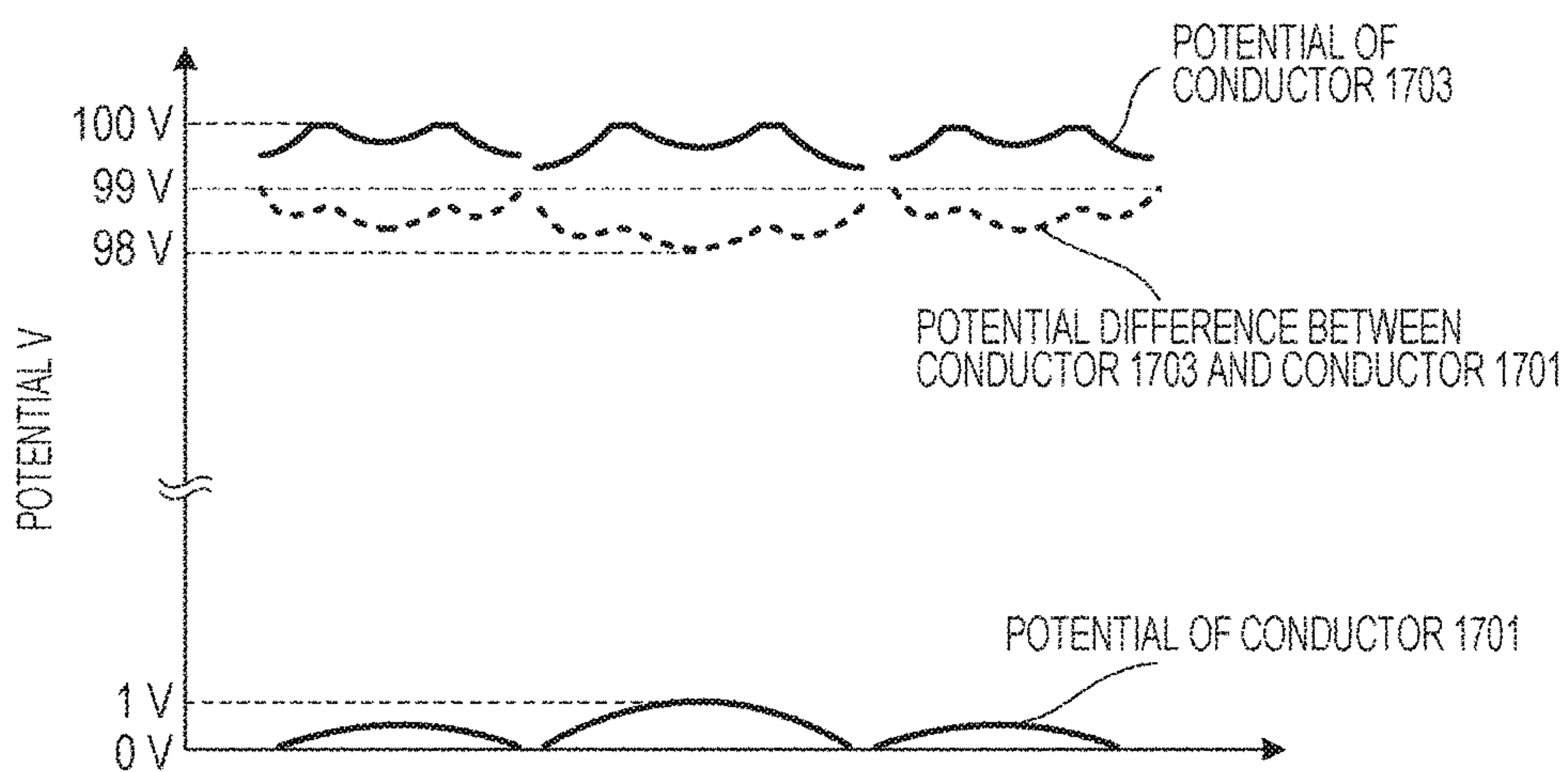
FIG. 17B
