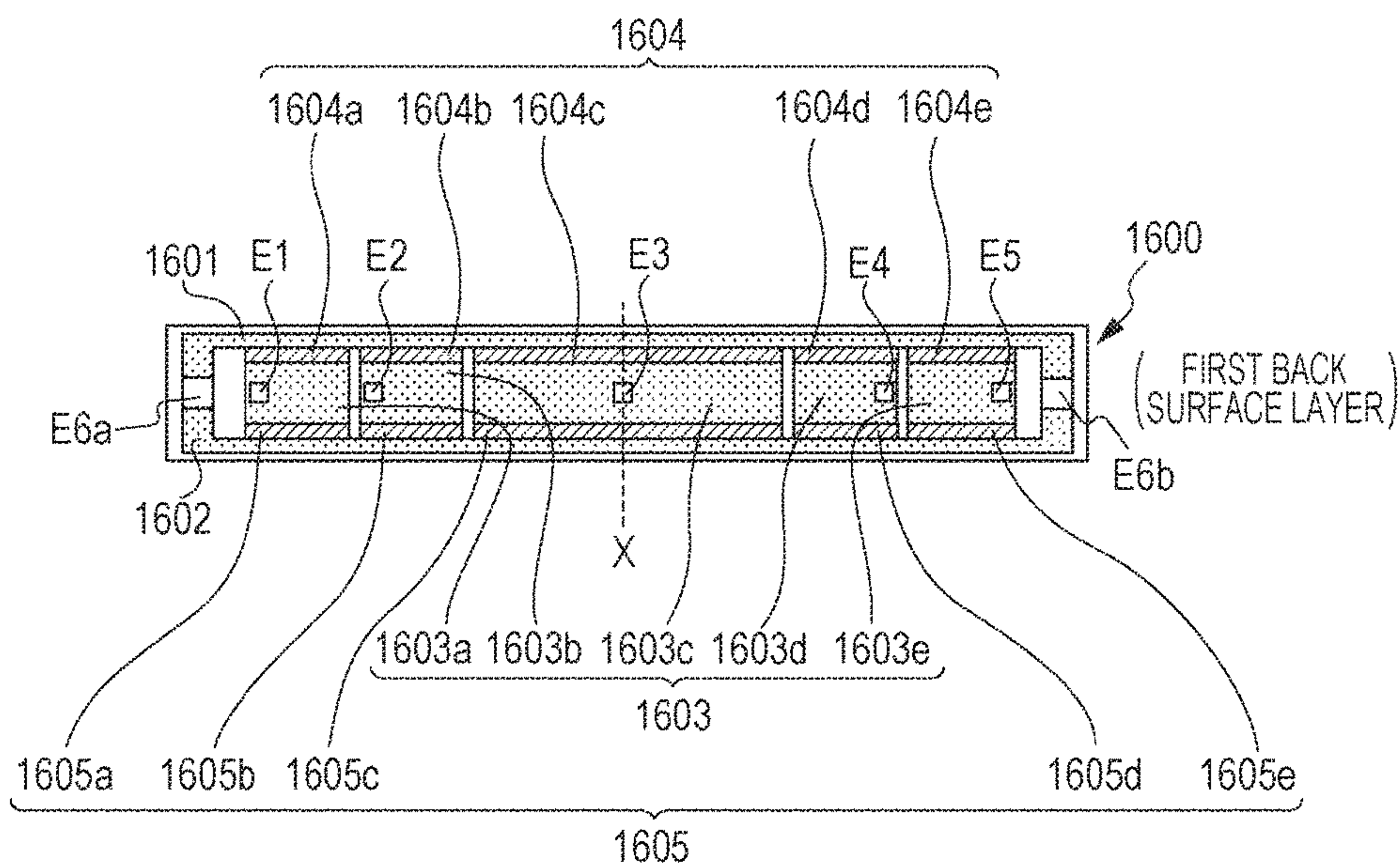
FIG. 16A
