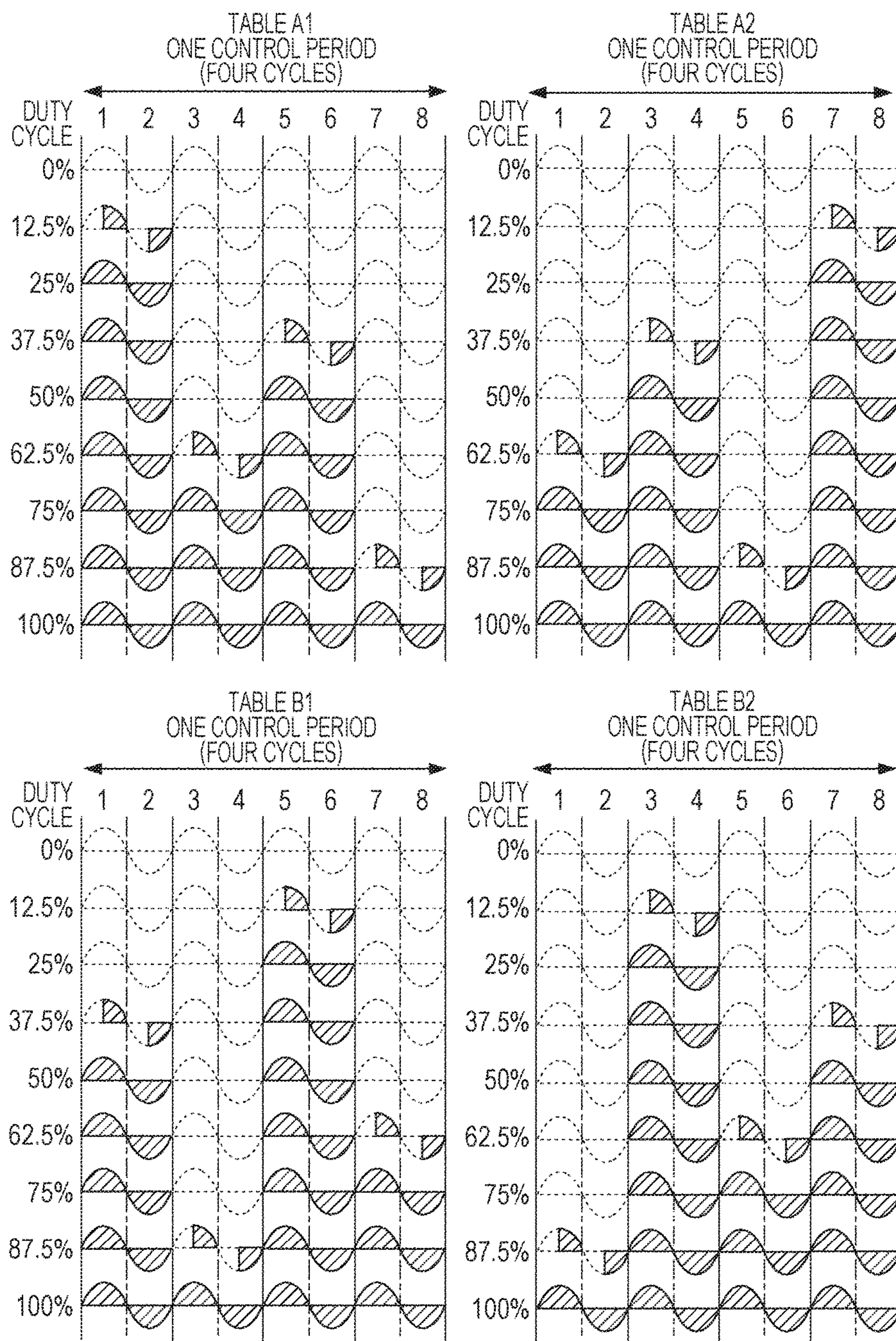
FIG. 27
