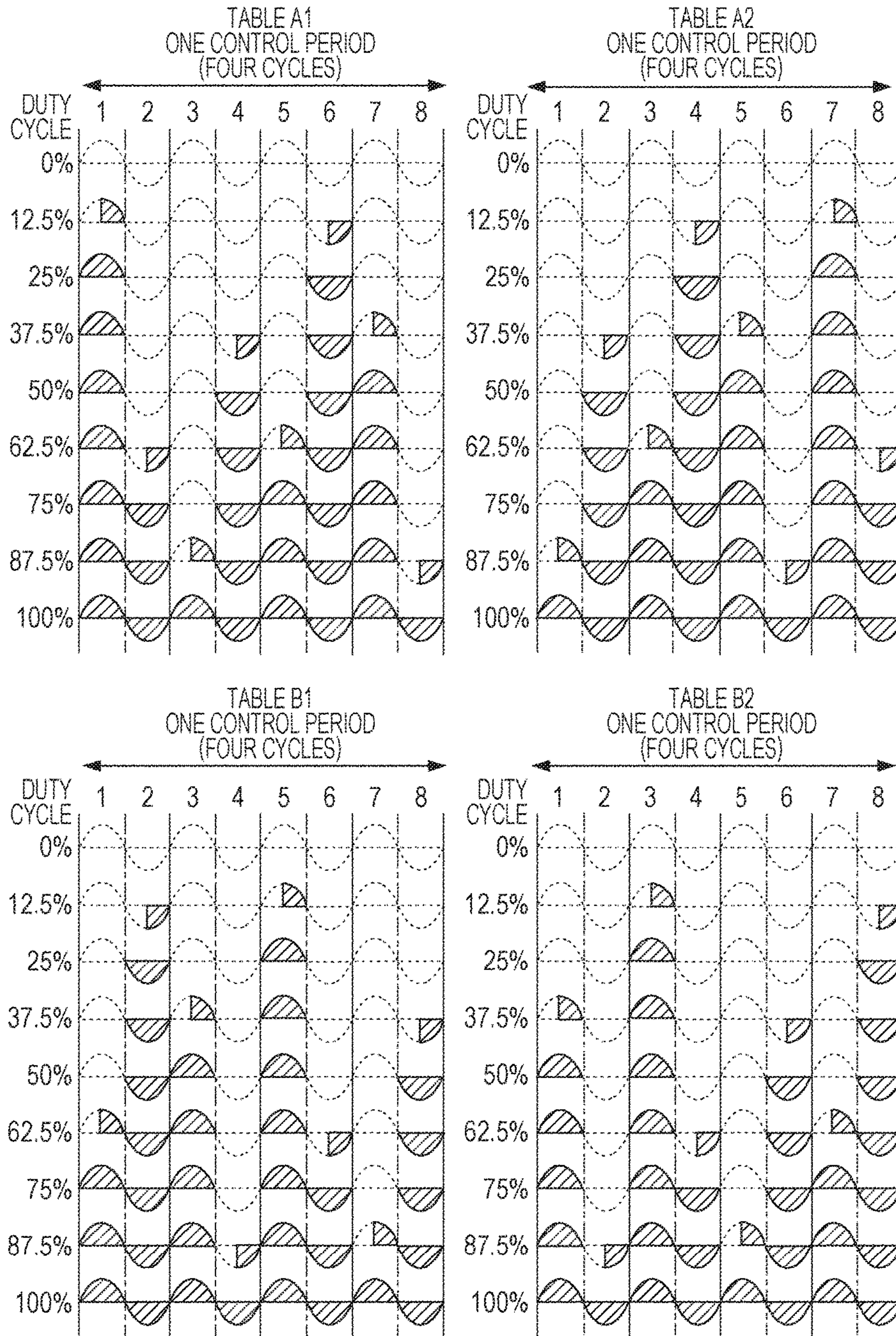
FIG. 28
