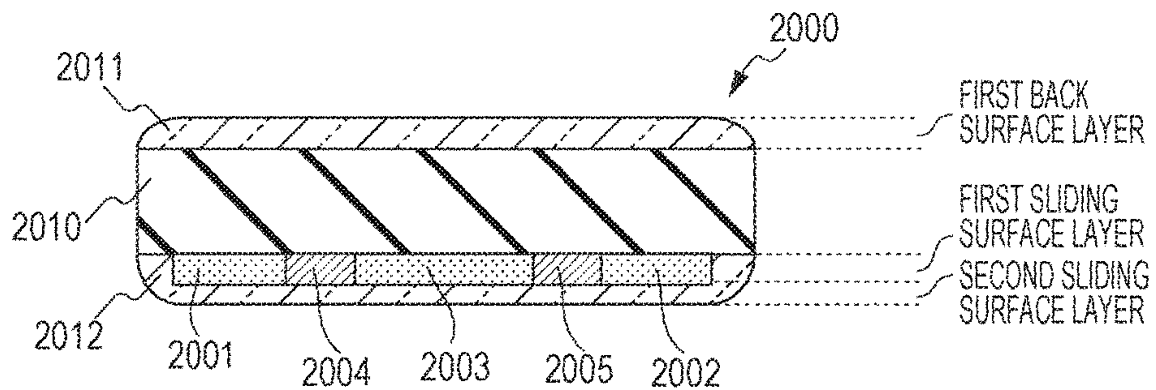
FIG. 20A
