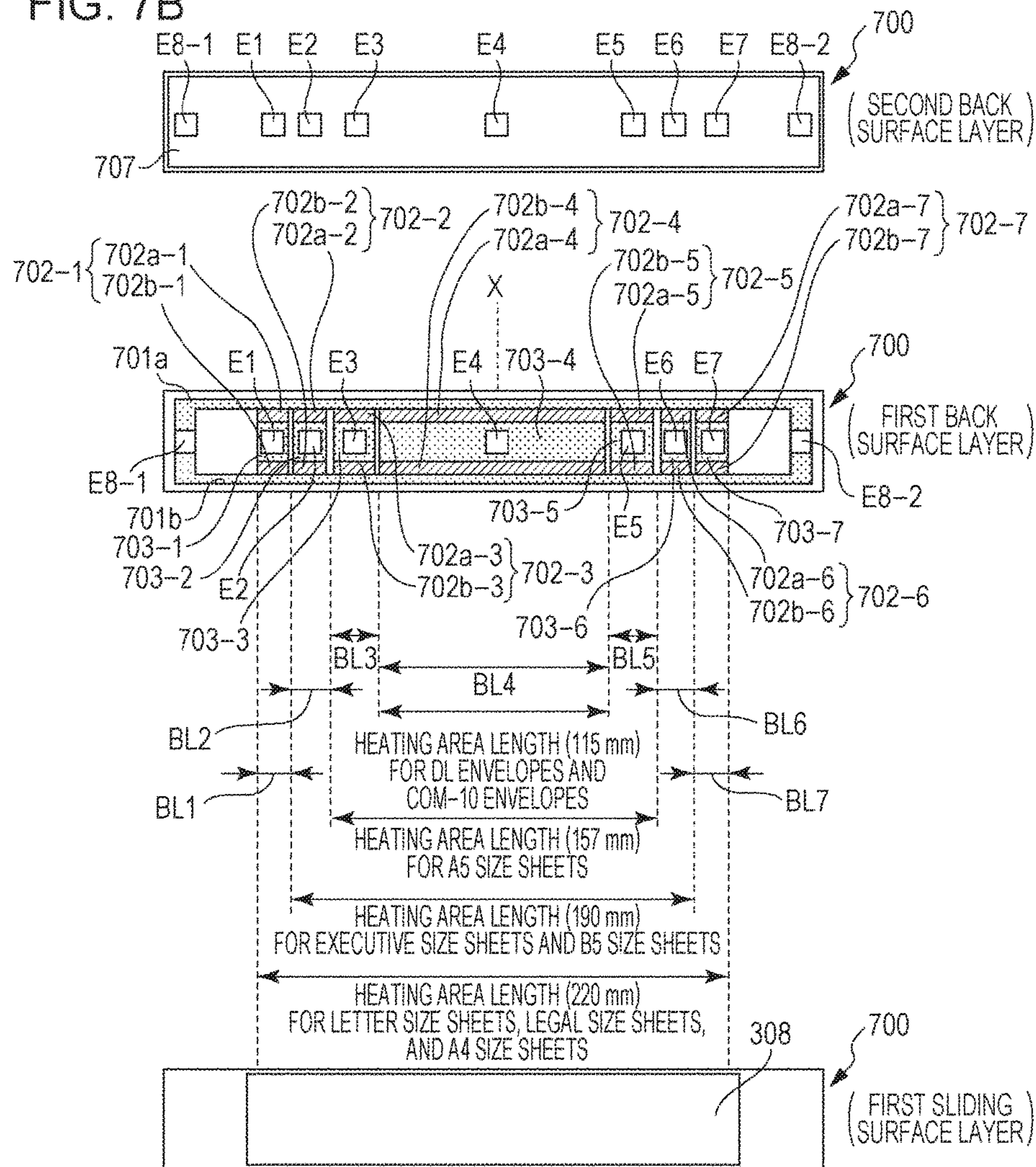
FIG. 7B
