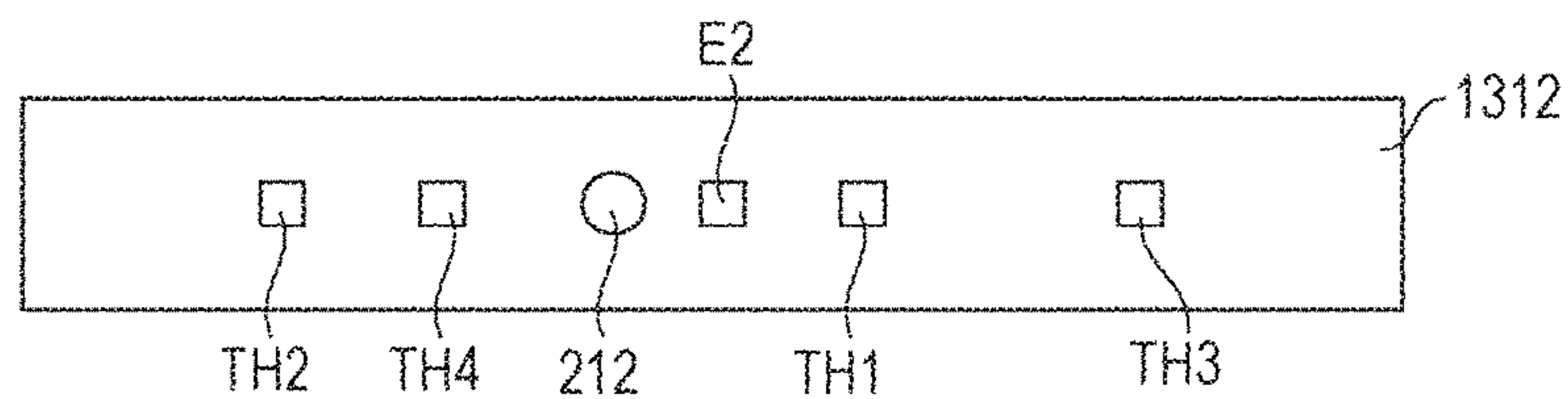
FIG. 13C
