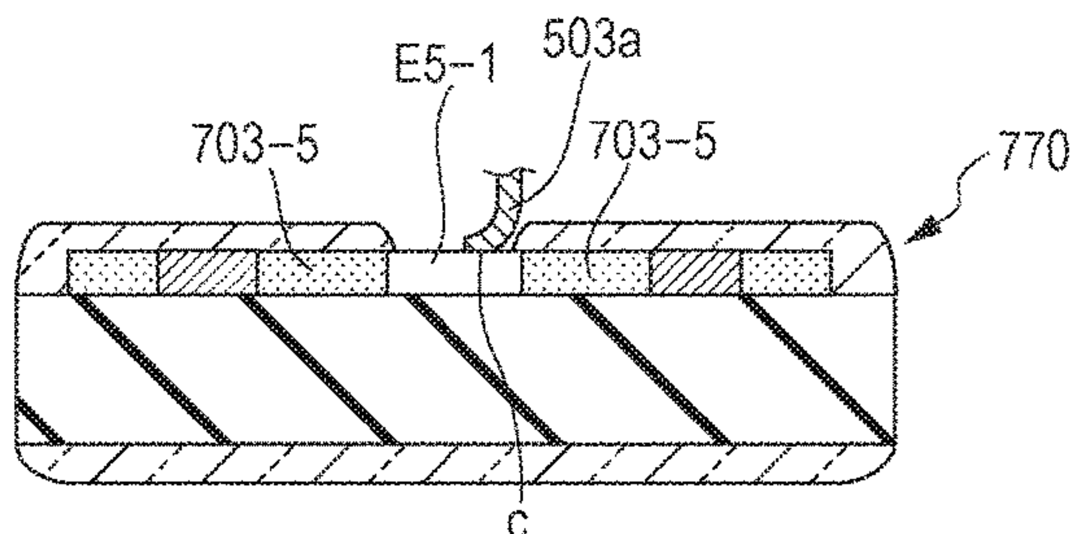
FIG. 32C
