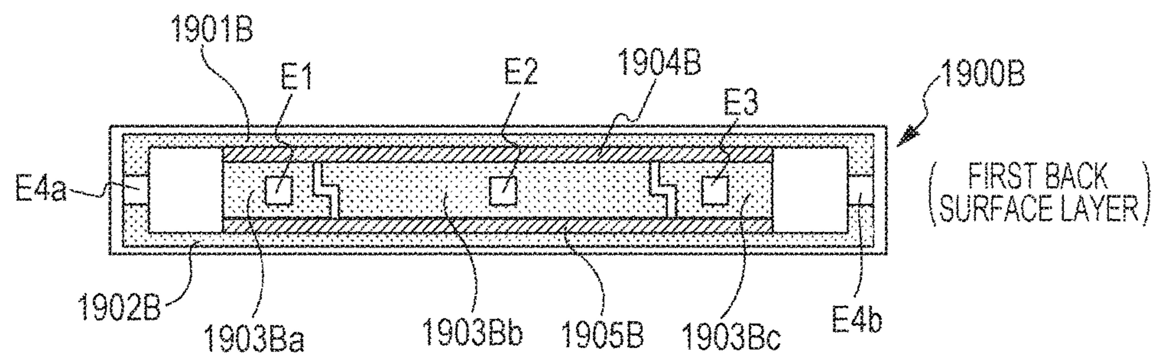
FIG. 19B
