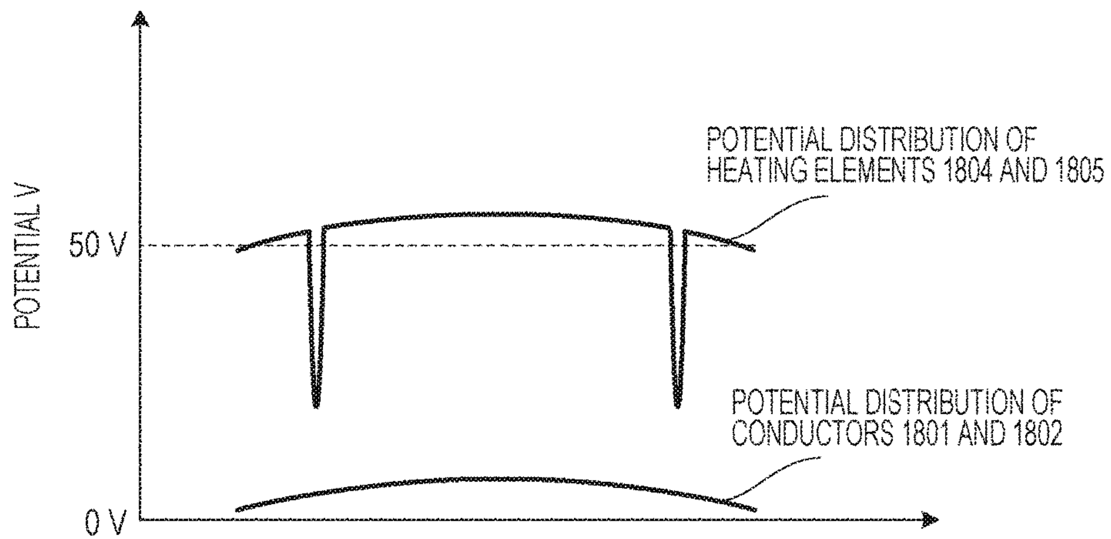
FIG. 18B
