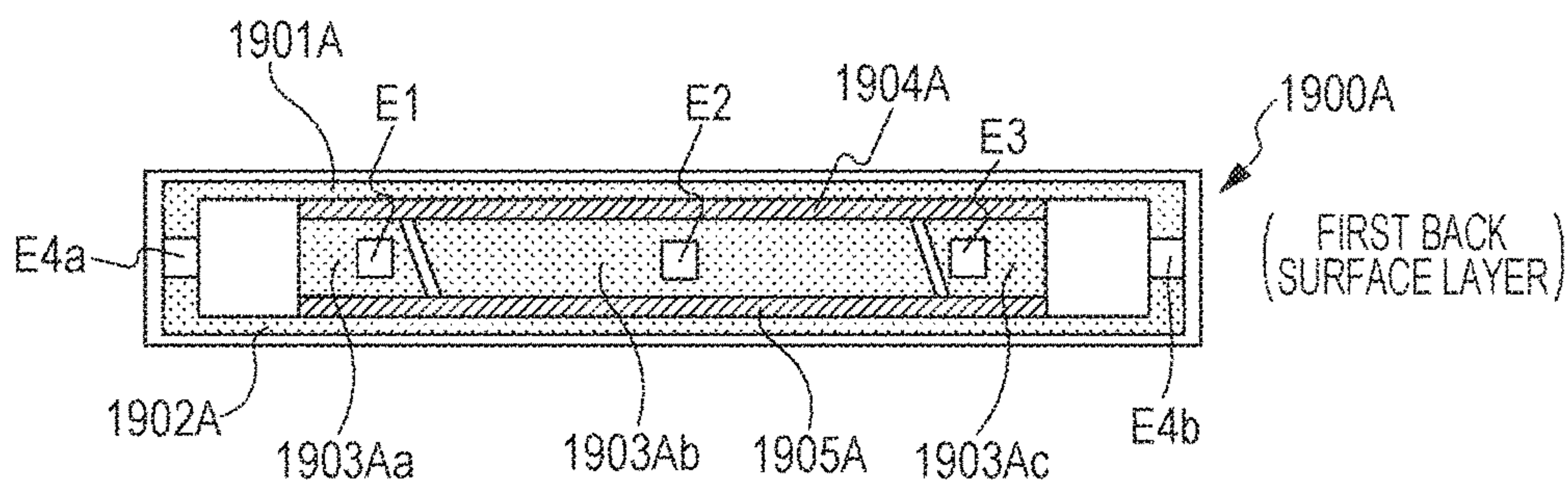
FIG. 19A
