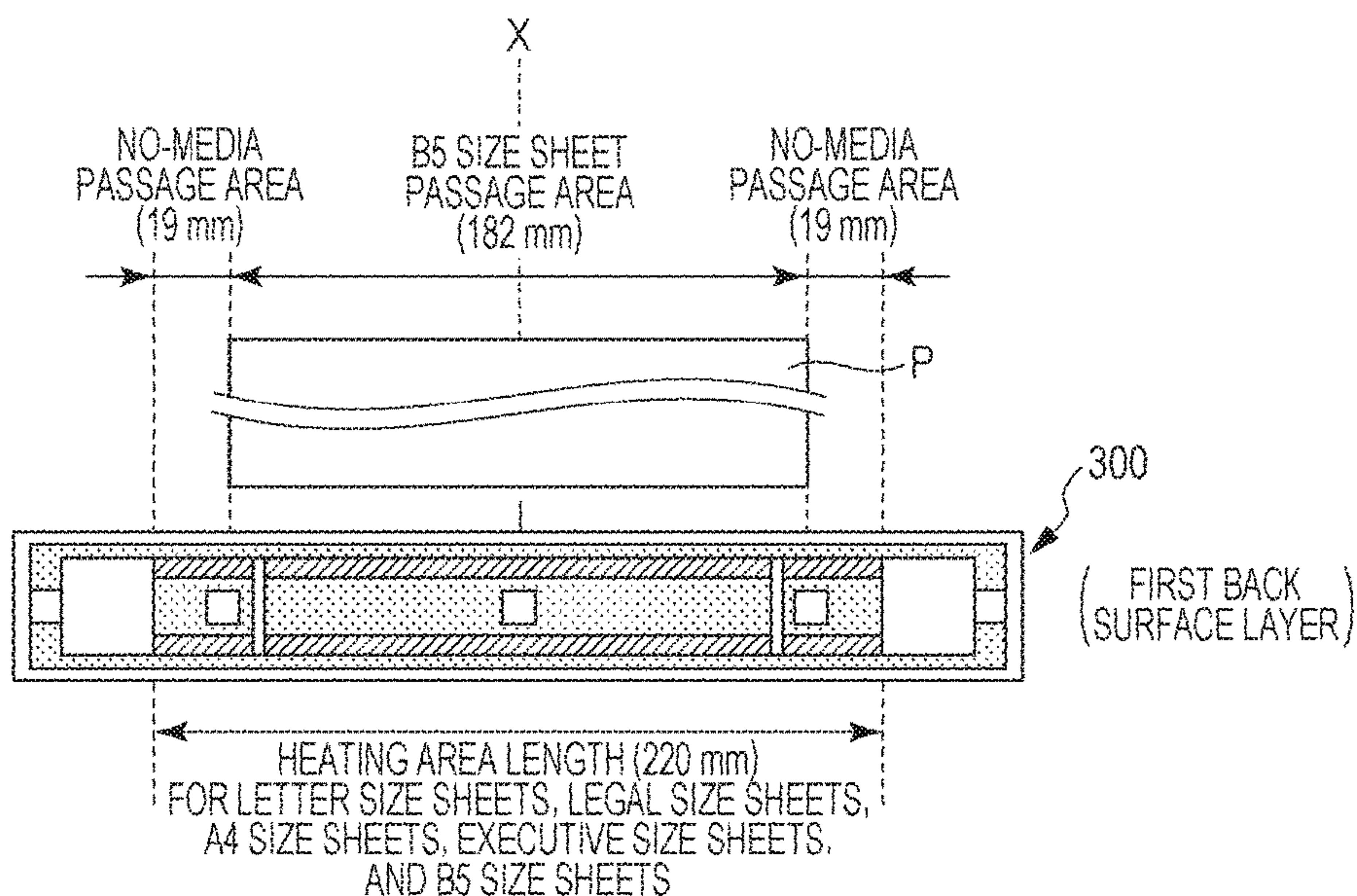
FIG. 6A
