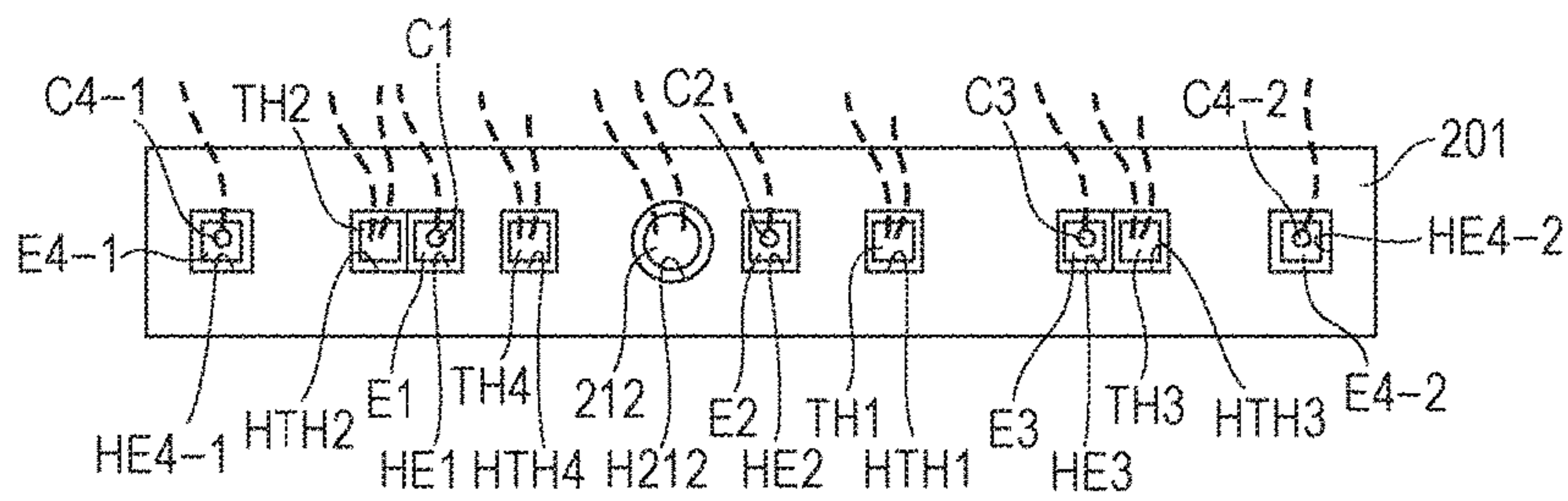
FIG. 3C
