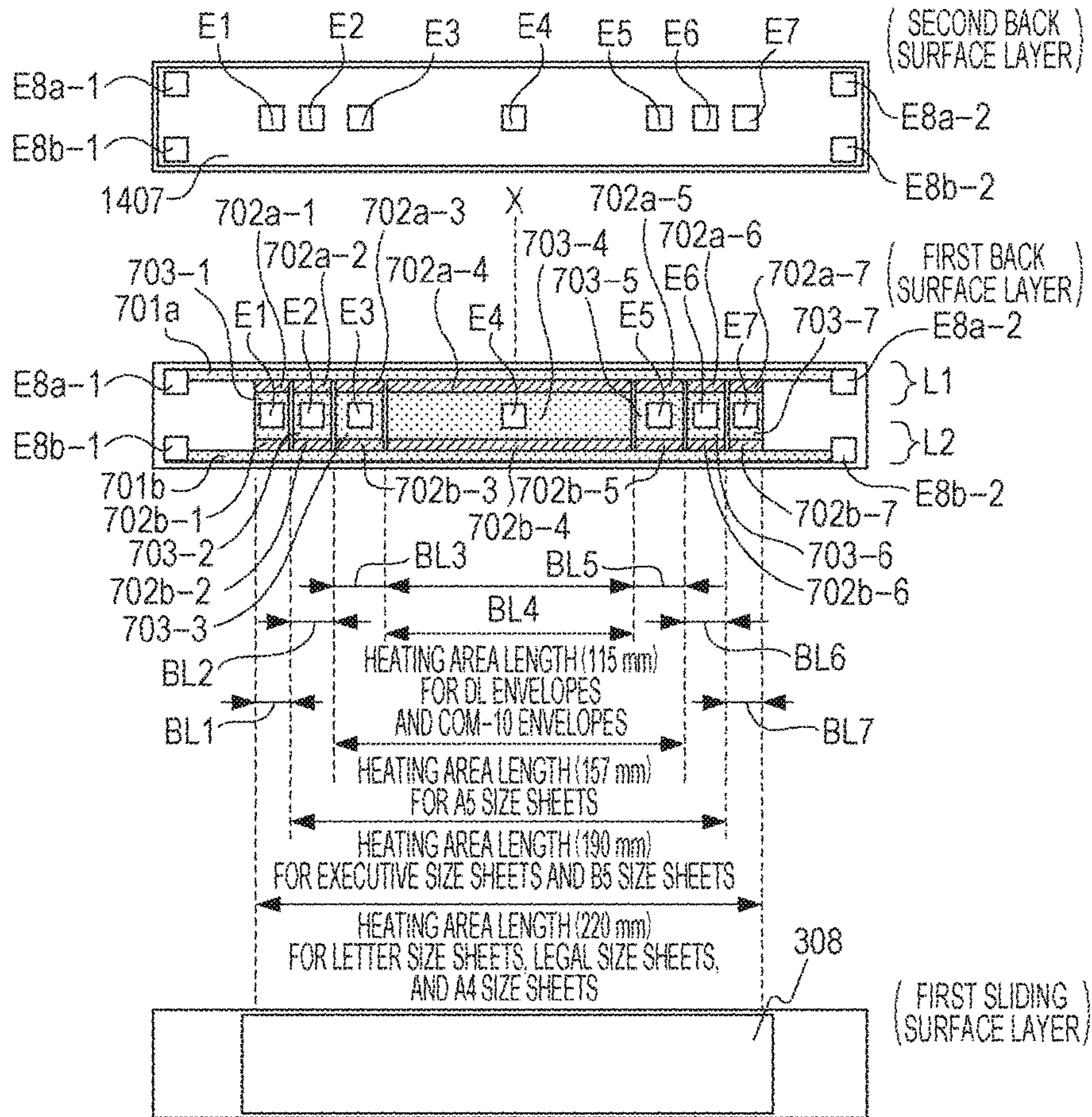
FIG. 21B
