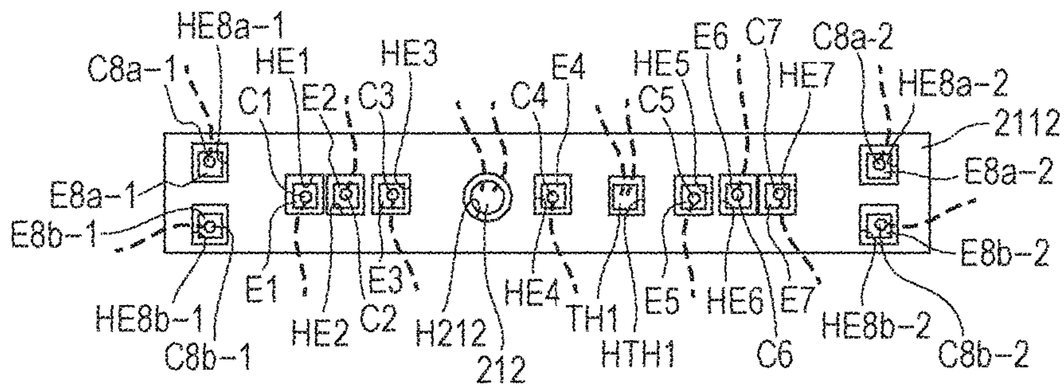
FIG. 21C
