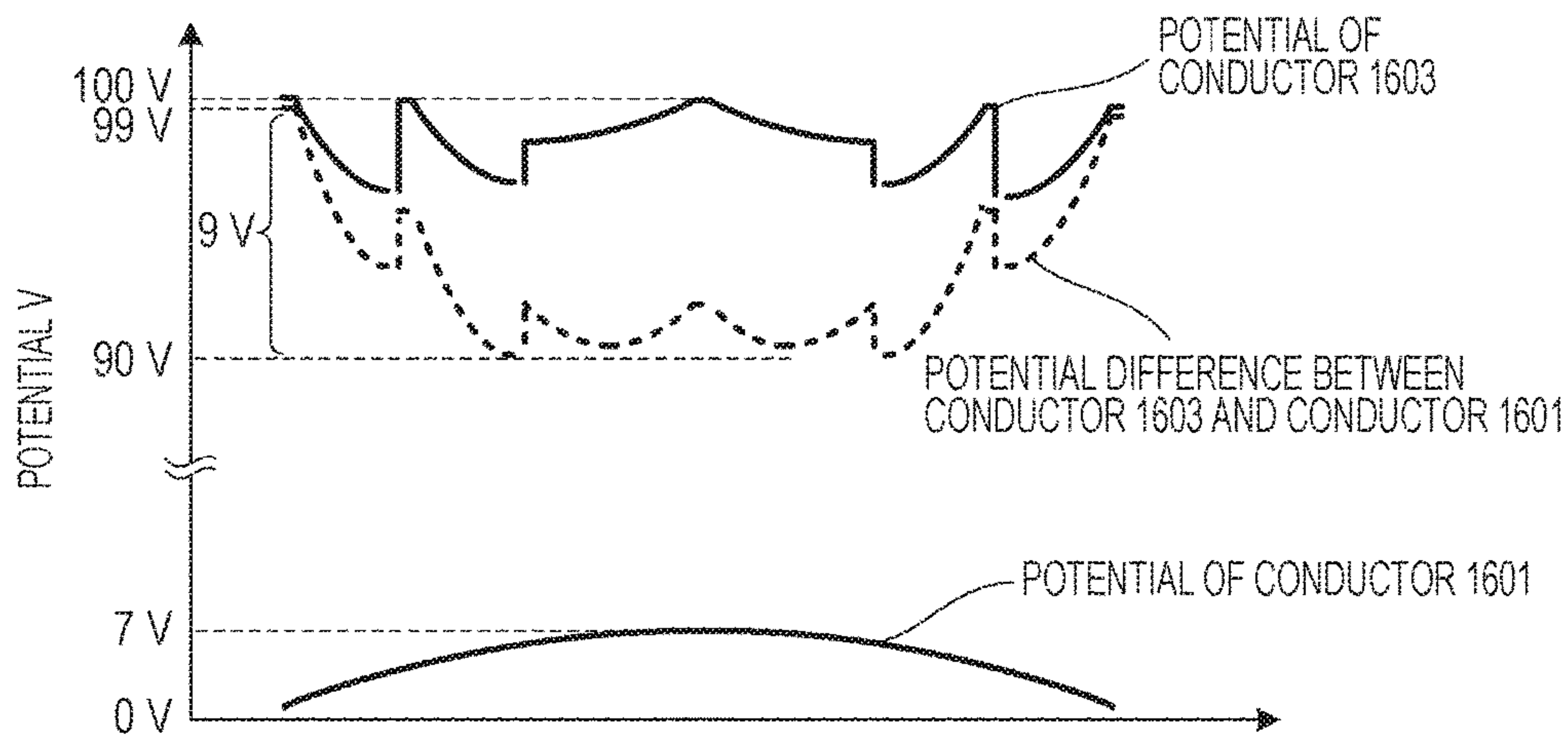
FIG. 16B
