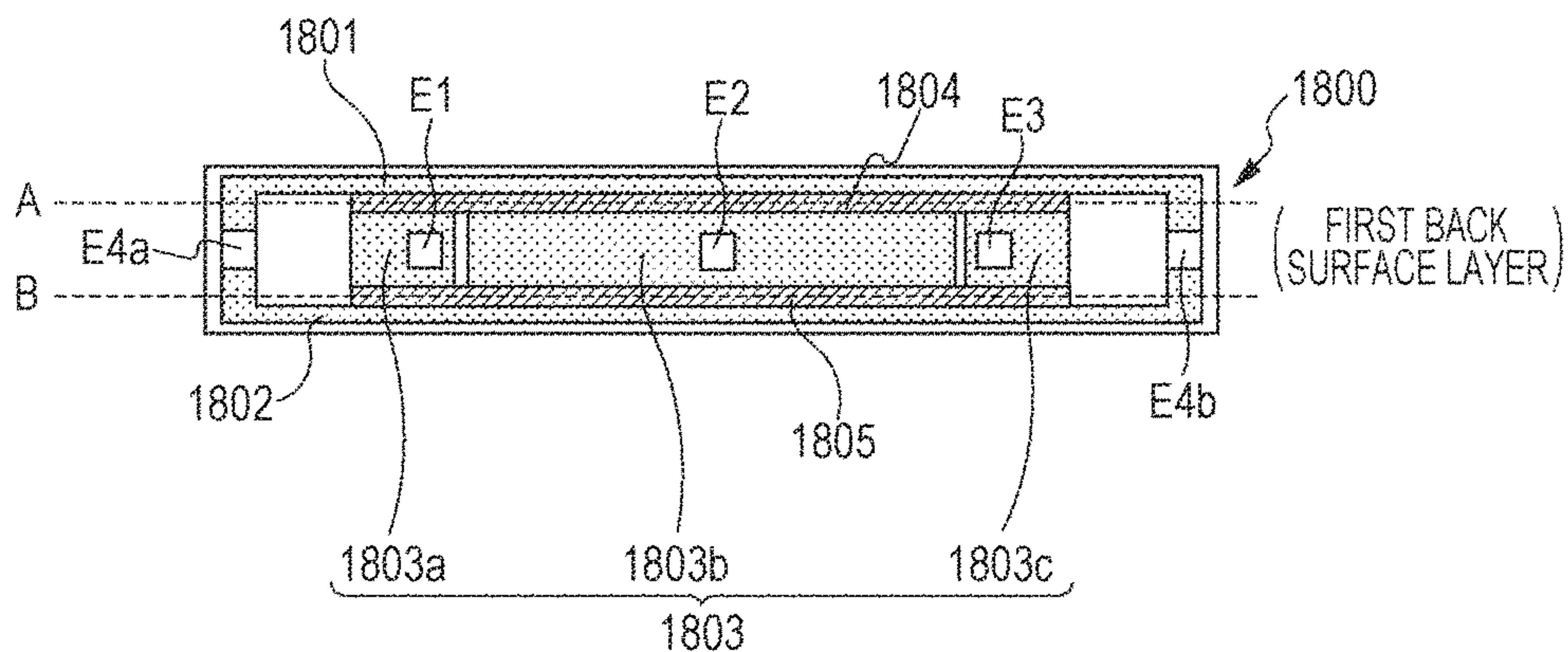
FIG. 18A
