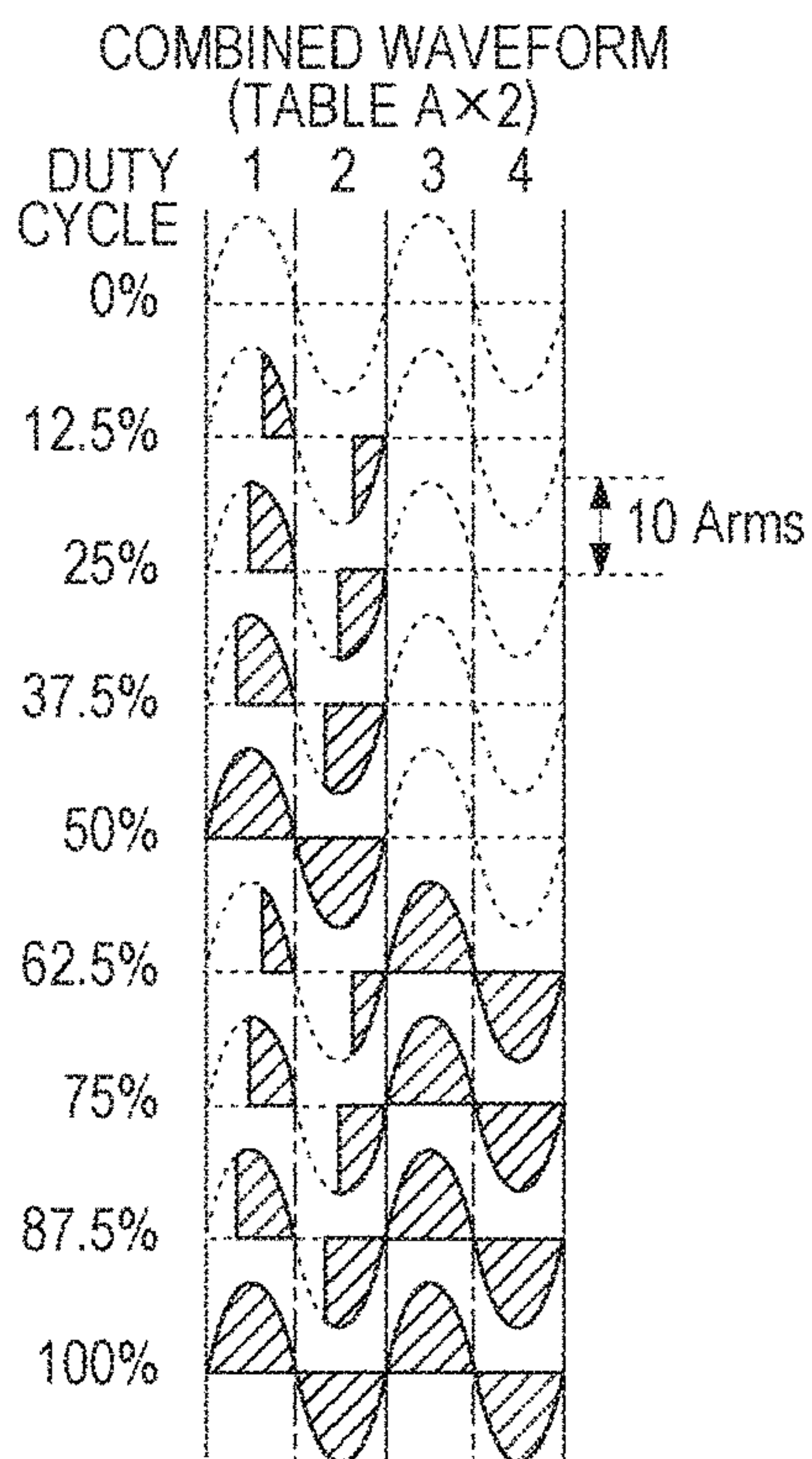
FIG. 23B
