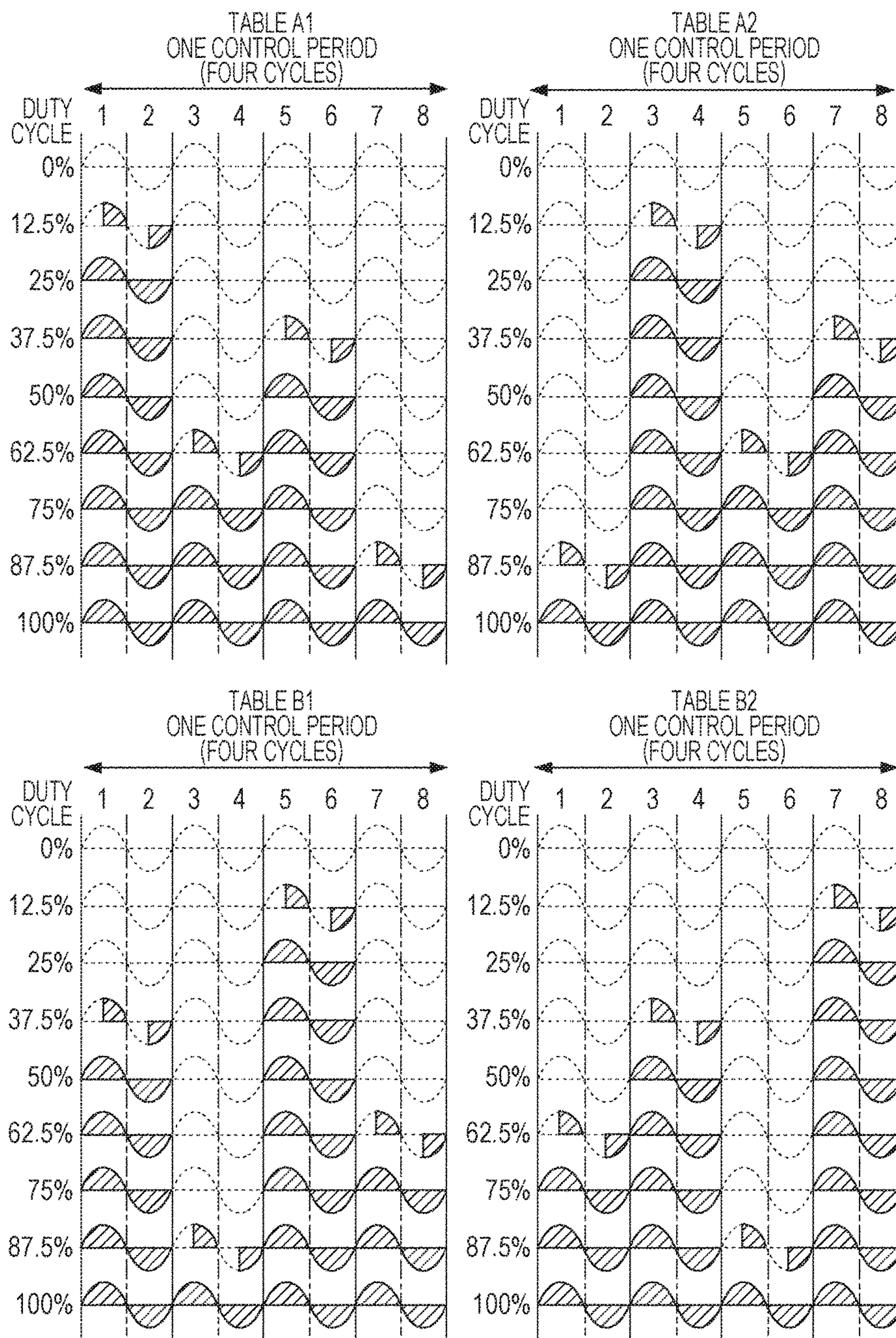
FIG. 26
