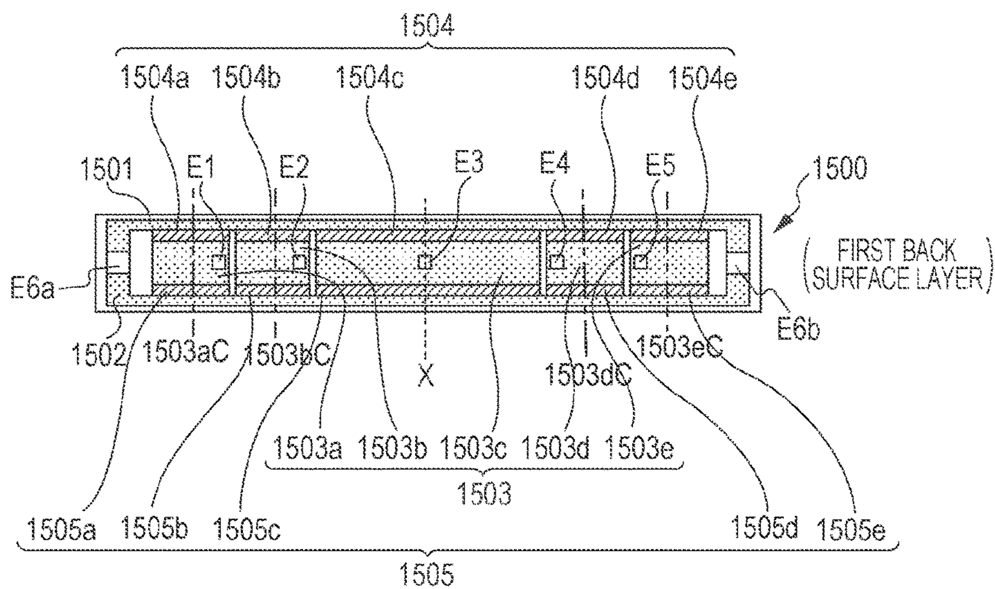
FIG. 15A
