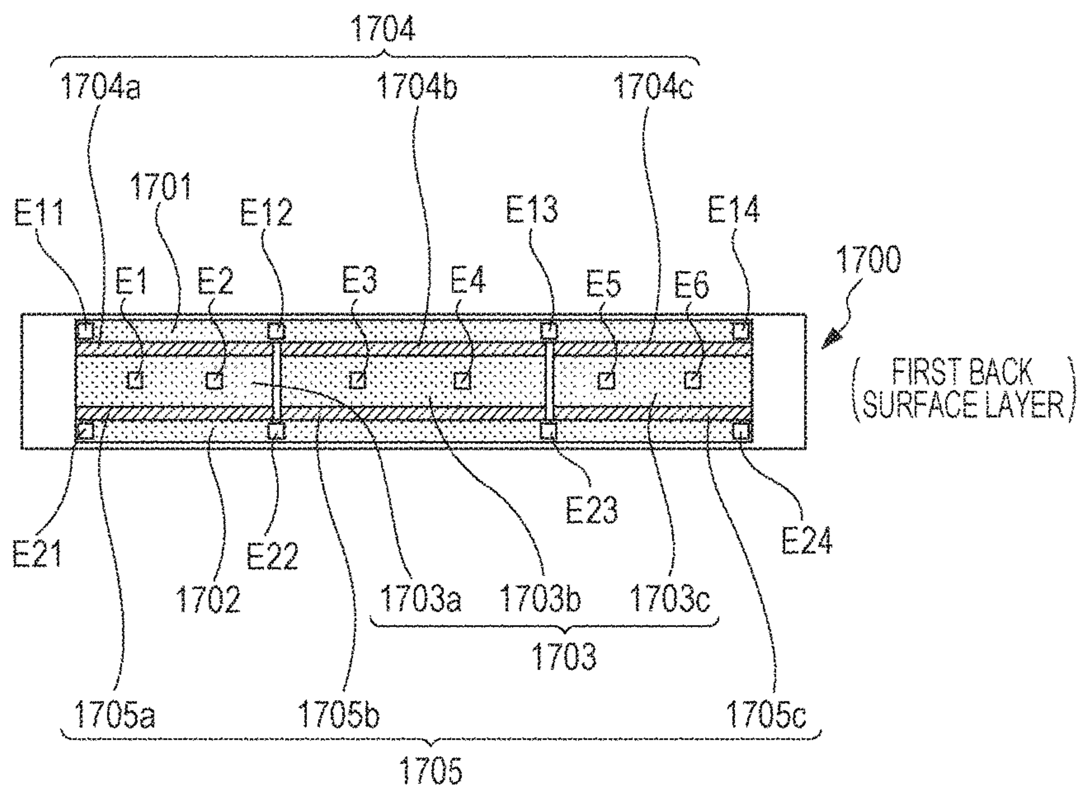
FIG. 17A
