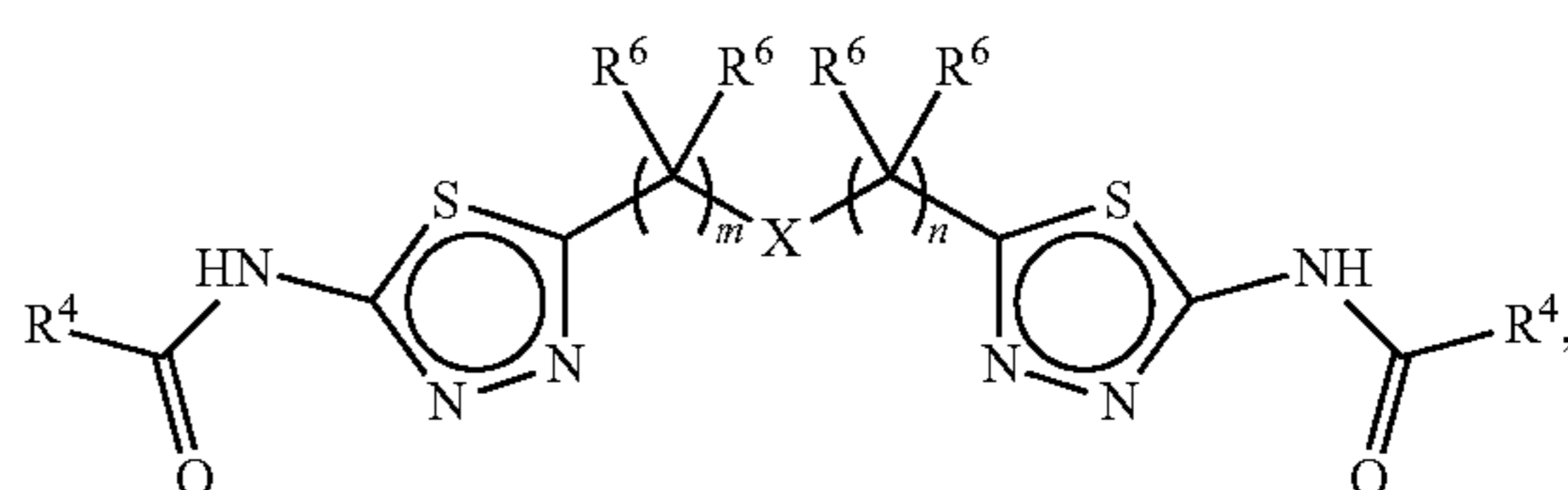
(III)
