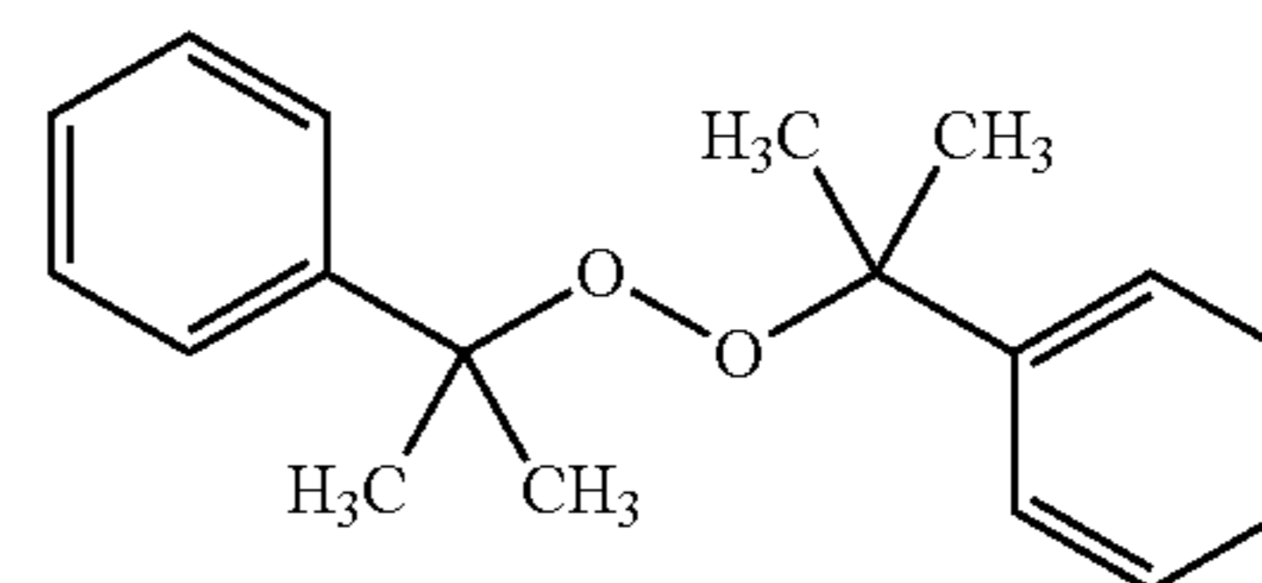
Dicumyl peroxide
