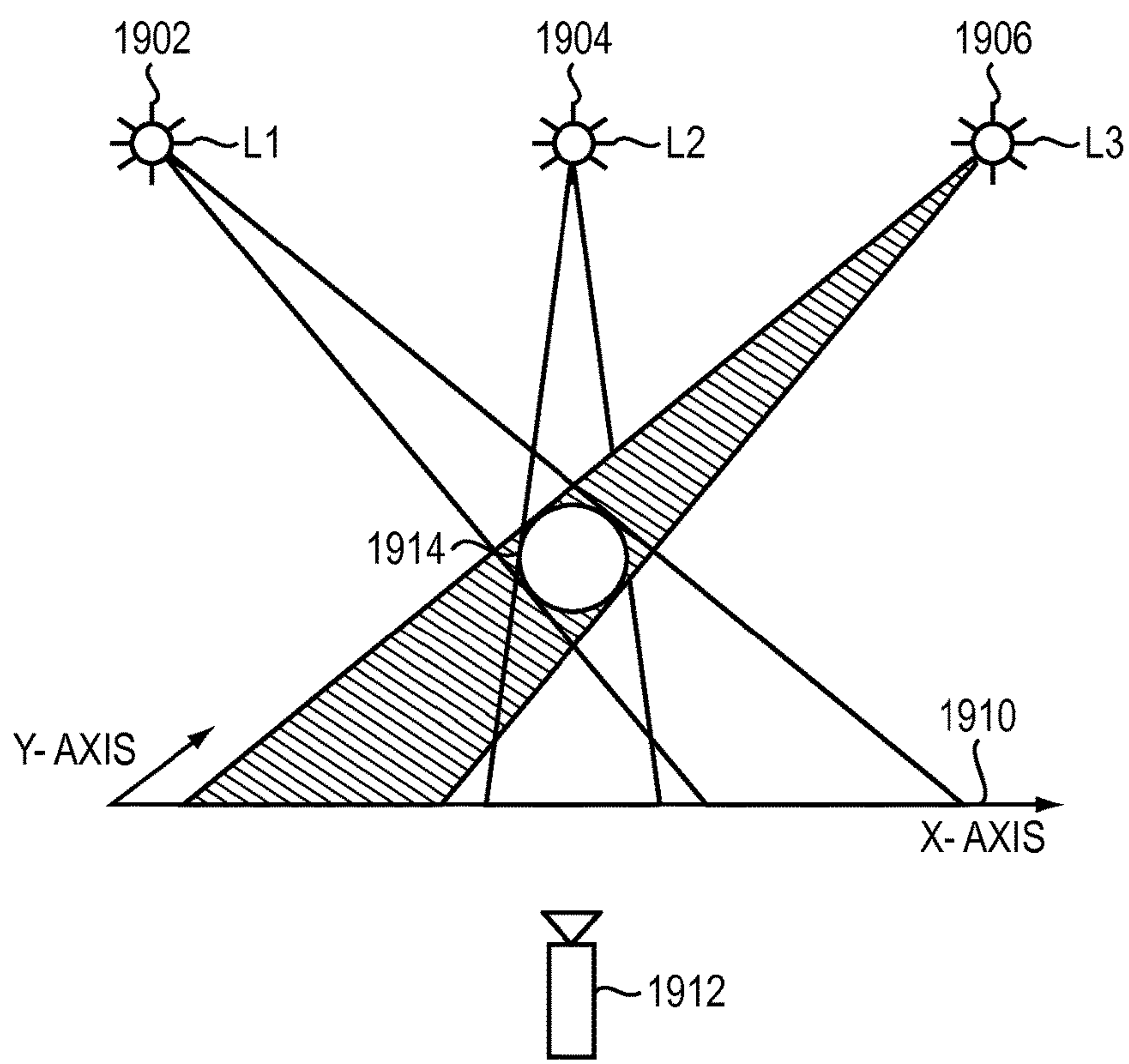
FIG. 19
