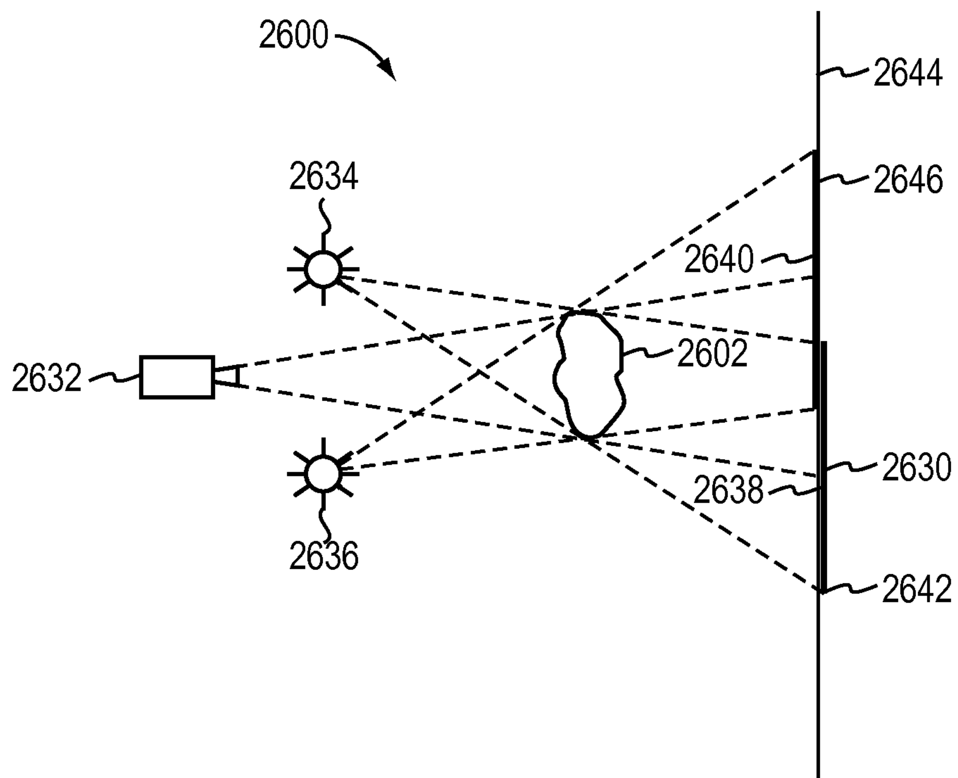
FIG. 26C
