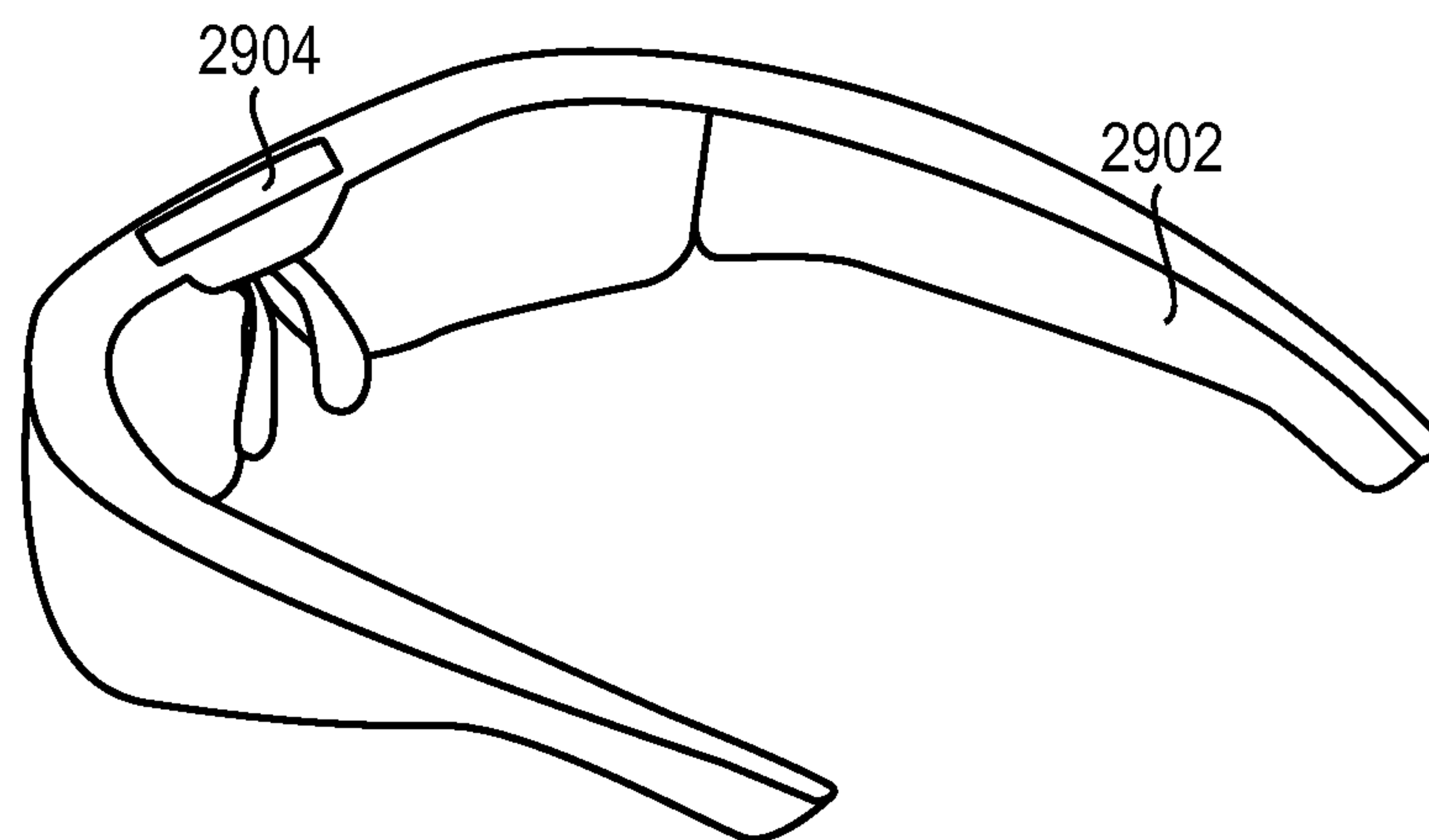
FIG. 29A
