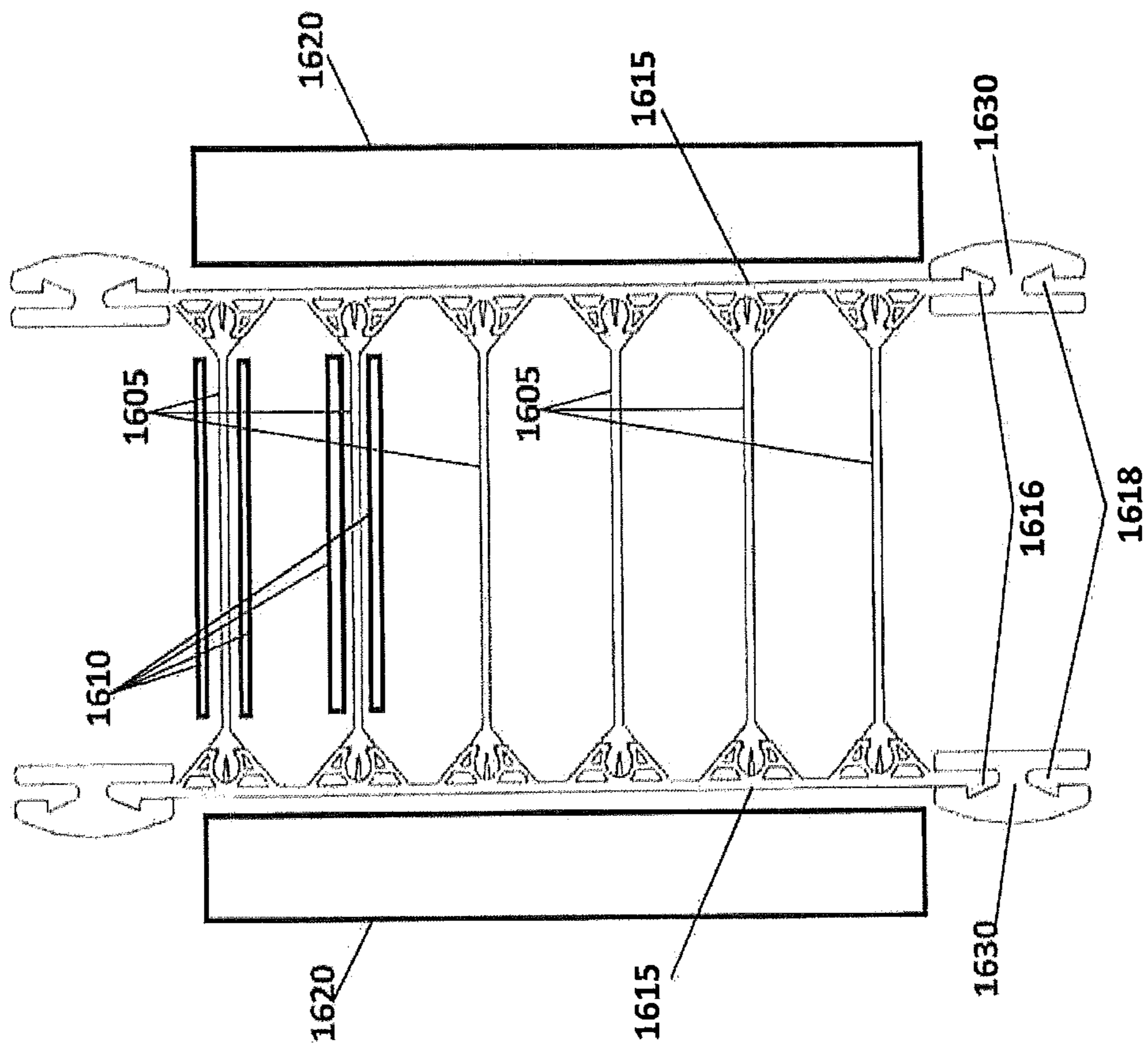
FIG. 16A
