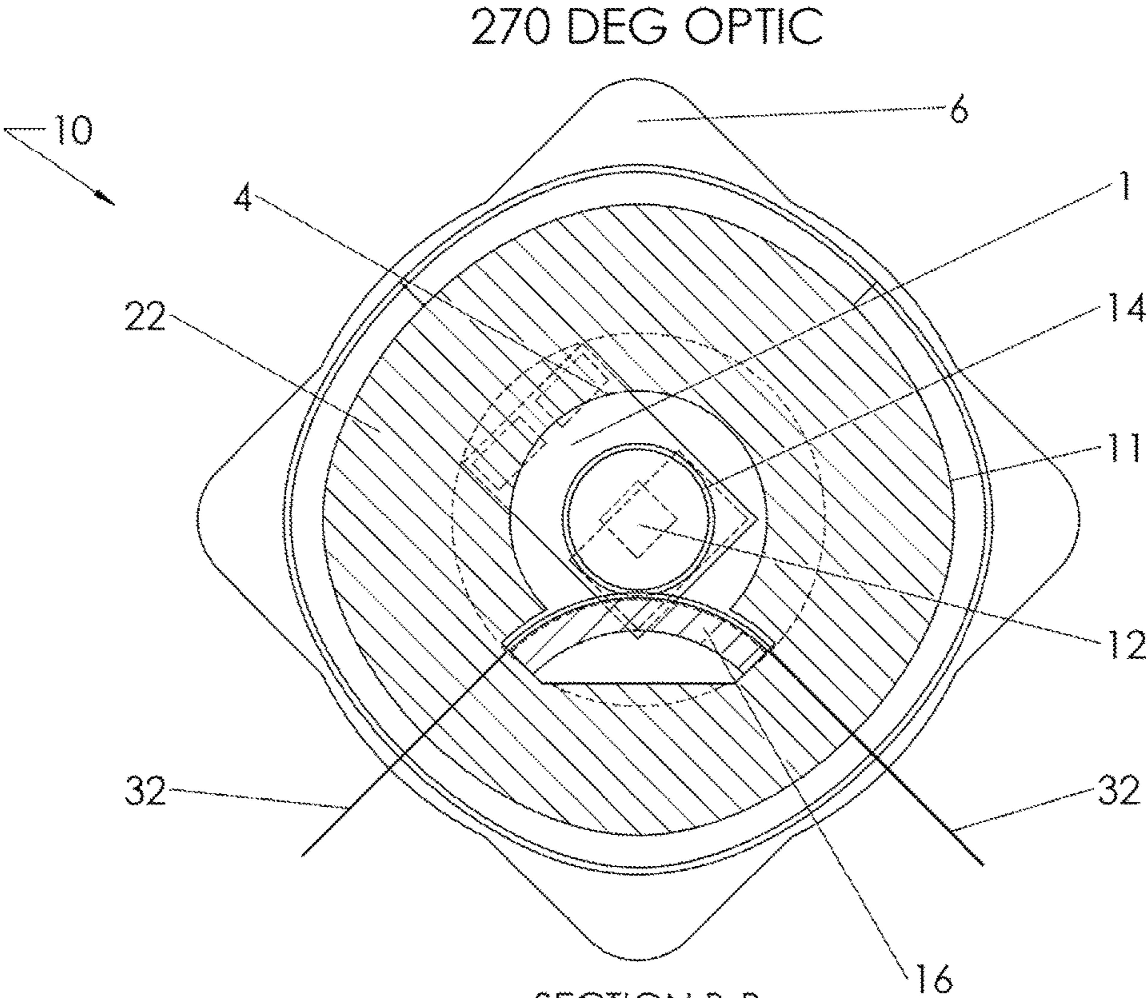
SECTION B-B FIG. 11a
