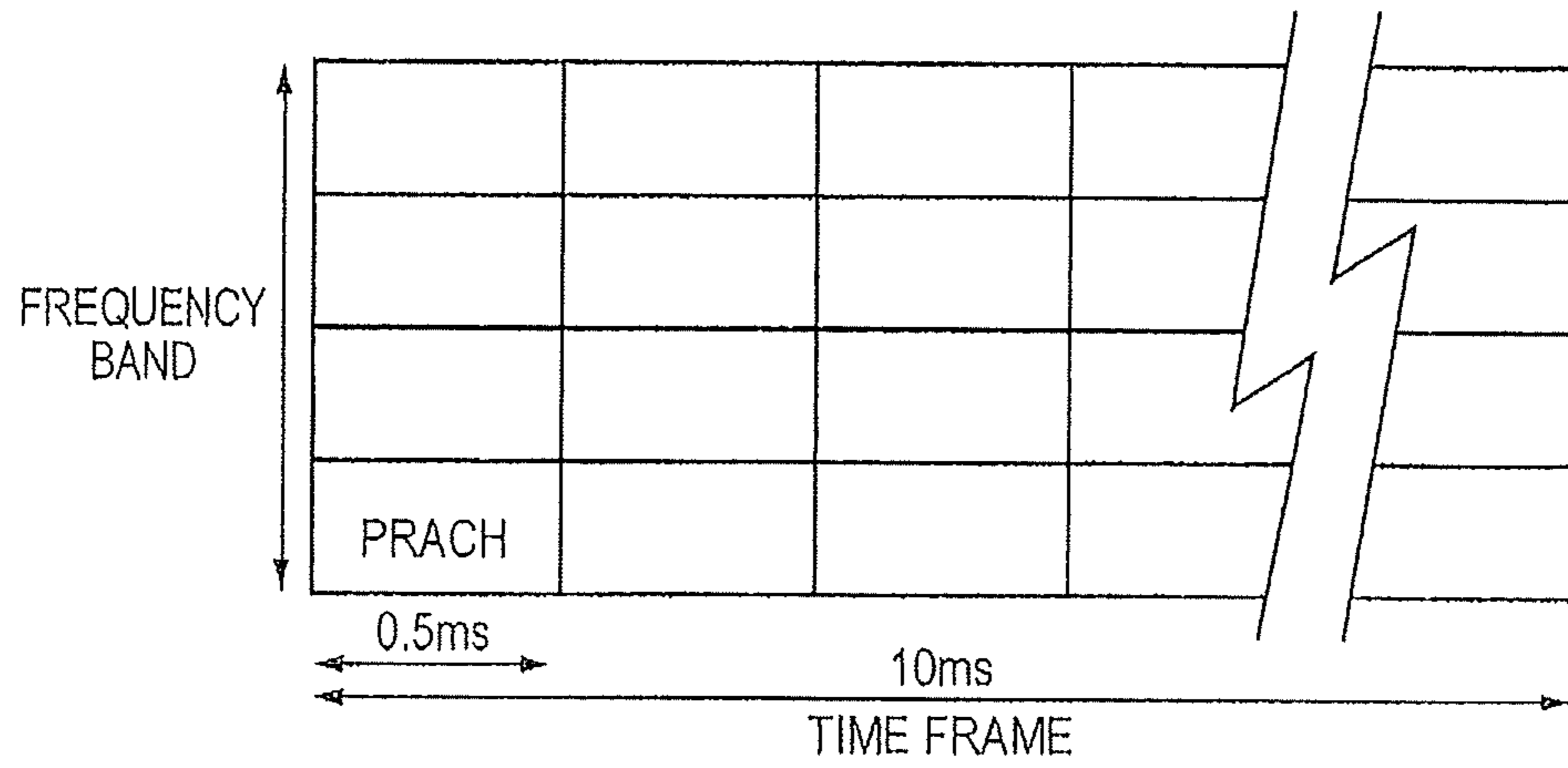
LTE UP-LINK
