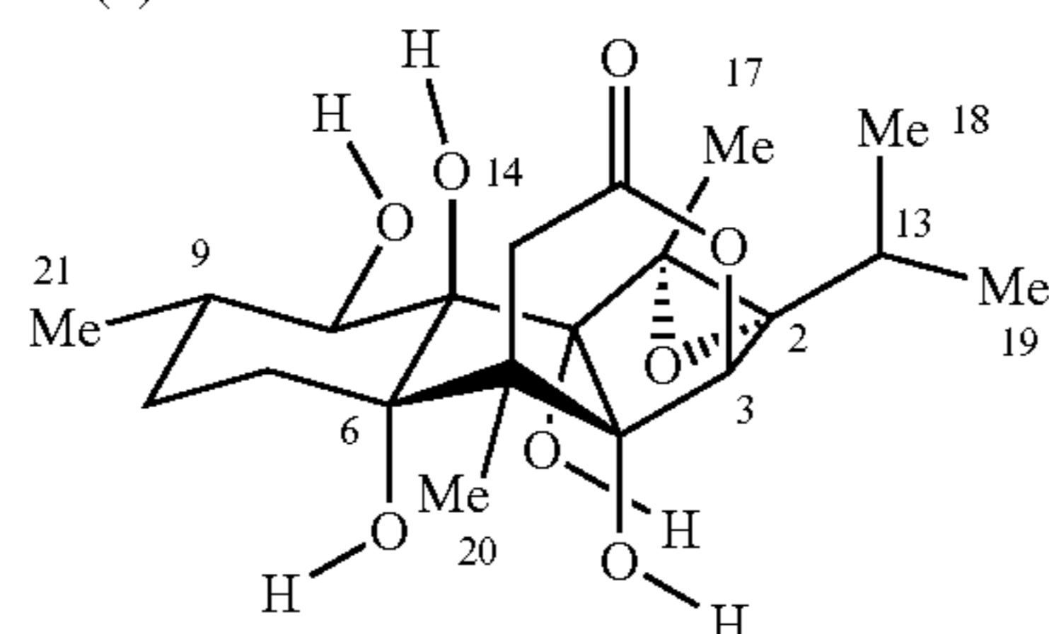
SI-4
