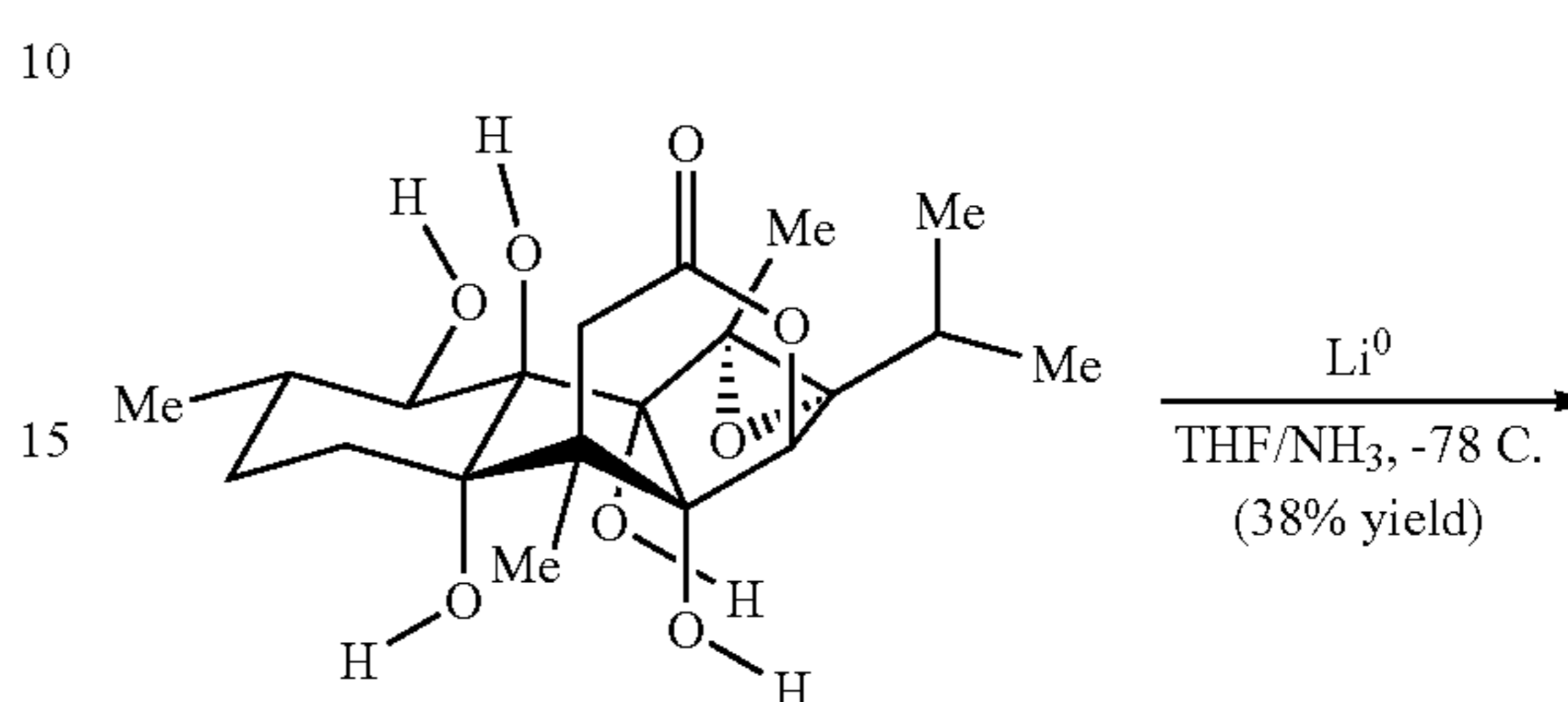
SI-4
