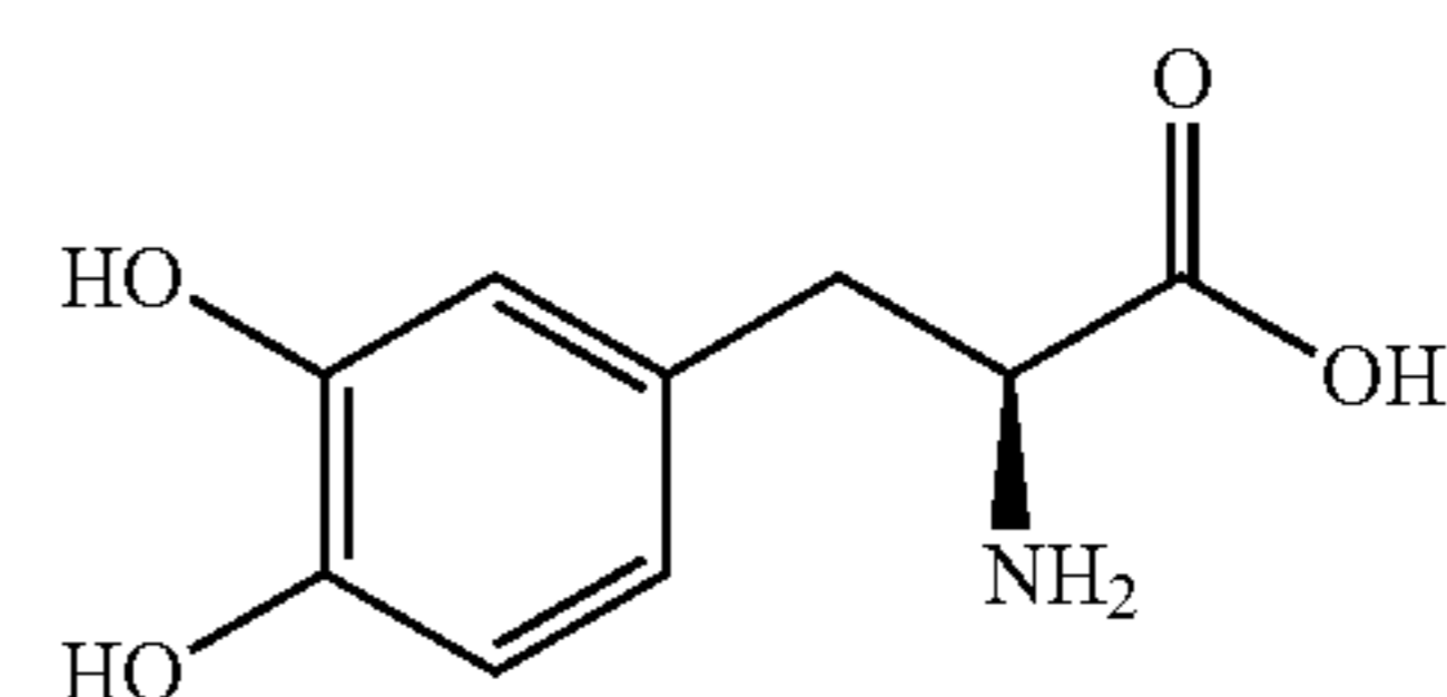
L-DOPA
