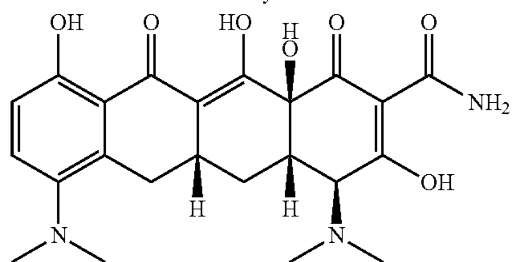
Monocycline
