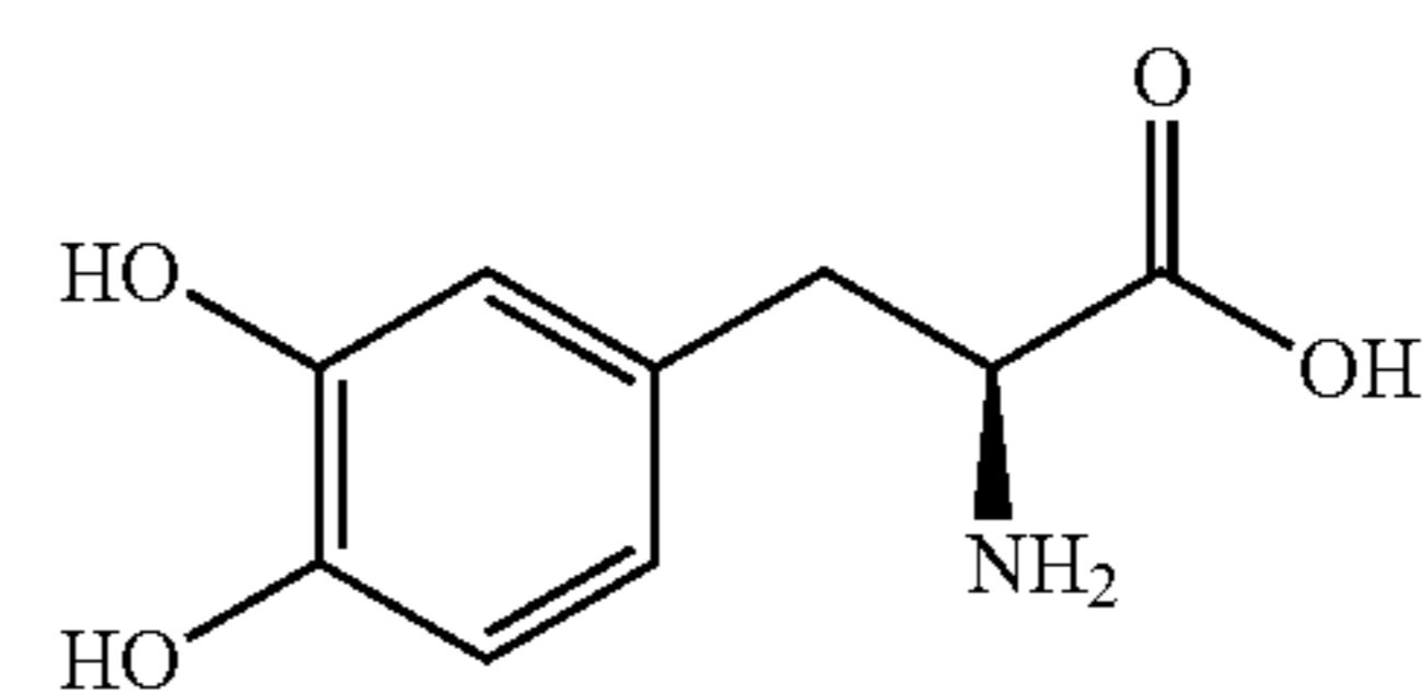
L-DOPA
