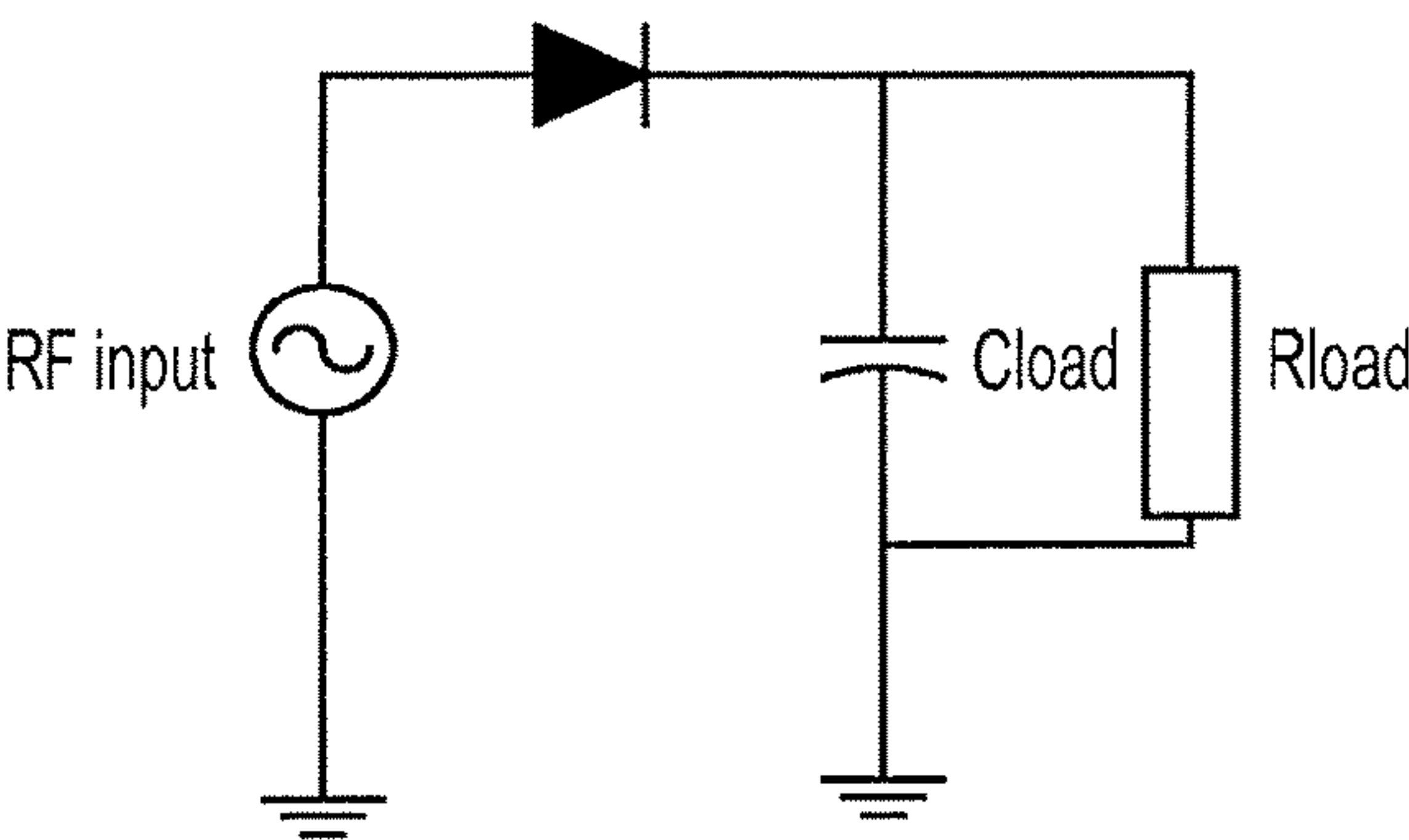
DIODE RECTIFIER FIG. 18A
