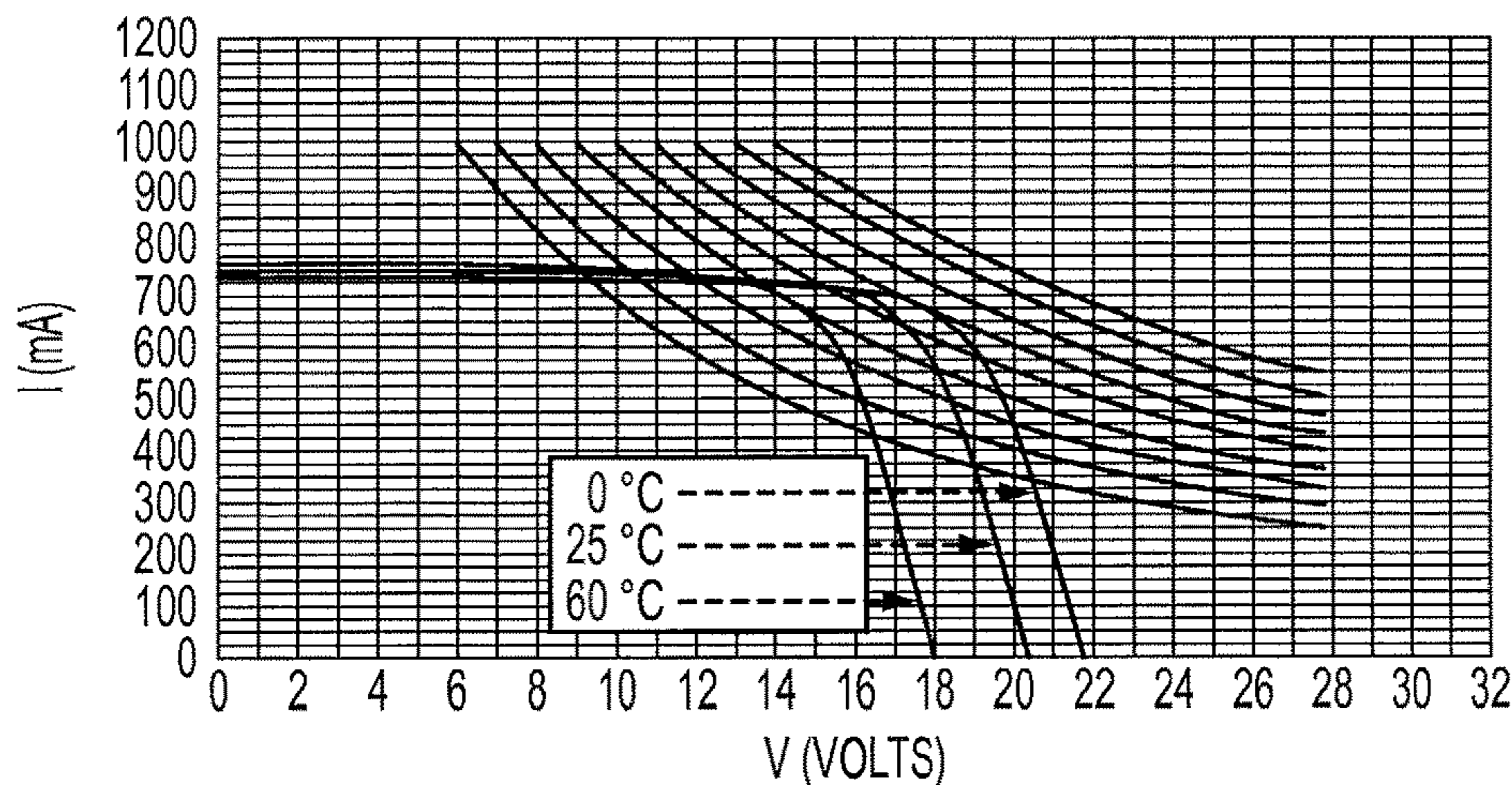
WIRED SOLAR CELLS FIG. 7E
